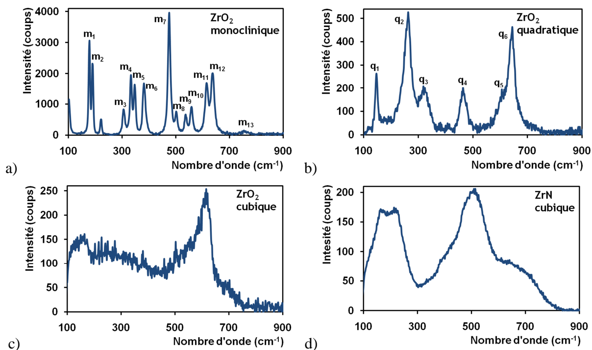
Figure III-2 : Spectres Raman acquis, dans les mêmes conditions, sur des échantillons de référence de a) zircon monoclinique, b) zircon quadratique, c) zircon cubique et d) nitrure de zirconium cubique
