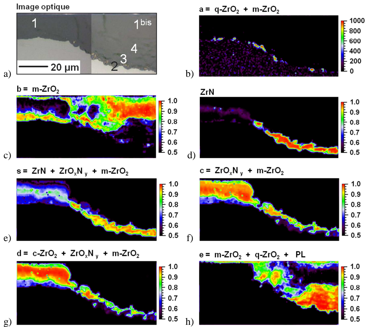
Figure IV-27 : a) Métallographie d'un oxyde de Zy-4 RXA formé à 800°C, avec la coexistence des couches pré- et post-transitoires. Images Raman de la b) zone a, c) zone b, d) ZrN, e) zone s, f) zone c, g) zone d et h) zone e
