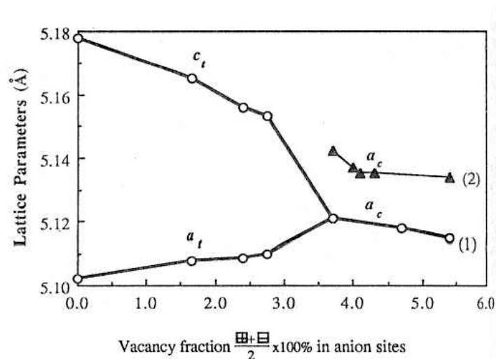
Figure I-22 : Variation de paramètres de maille de la zirconie en fonction du pourcentage de lacunes anioniques pour (1) (3Y)ZrO_2 + N_2 , et (2) (8Y)ZrO_2 + N_2 (Cheng & Thompson 1993)
