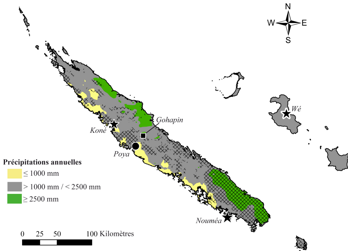
Figure 2.5 Carte des précipitations annuelles. La zone grise (précipitations comprises entre 1000 et 2500 mm par an) hors zone hachurée (correspondant aux substrats ultramafiques et serpentineux), représente la zone où les savanes et les forêts denses humides peuvent être deux états alternatifs stables (voir Figure 2.3). Carte réalisée à partir des données de l'Atlas de Nouvelle-Calédonie.
