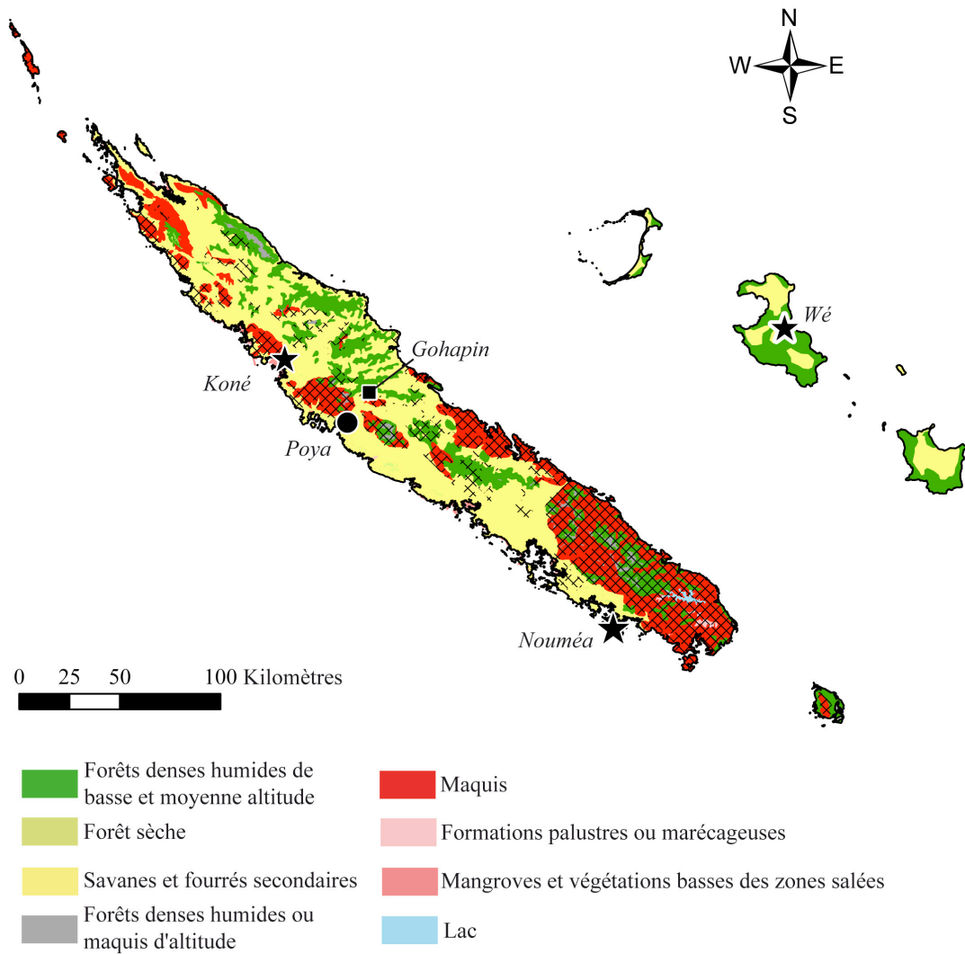
Figure 2.1 Carte simplifiée de la végétation de la Nouvelle-Calédonie (modifiée de l'Atlas de Nouvelle-Calédonie). Les zones hachurées représentent les sols ultramafiques et serpentineux.
