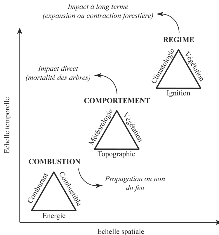
Figure 2.6 Interactions entre les principaux facteurs caractérisant l'écologie du feu à différentes échelles spatiales et temporelles.
