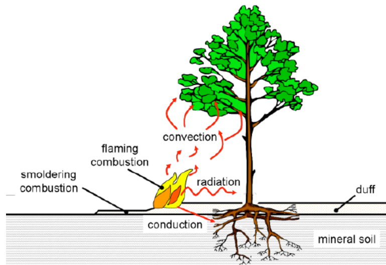
Figure 2.7 Processus de transferts de chaleur depuis la combustion vers un arbre (tiré de Michaletz and Johnson 2007).
