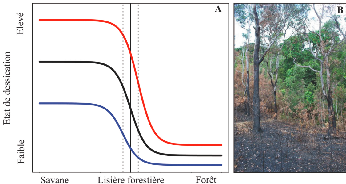
Figure 12.2 (A) Conditions microclimatiques (état de dessiccation) le long de la zone de transition entre la savane et la forêt dense humide durant des périodes anormalement humides (type La Niña, ligne bleue), anormalement sèches (type El Niño, ligne rouge)
