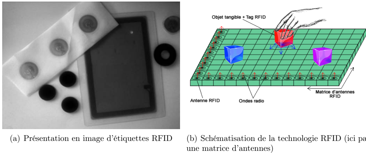
FIGURE 1.6 – Exemple d'étiquettes (ou tags) RFID (a) et schéma de la technologie de capture par matrice d'antennes RFID (b)
