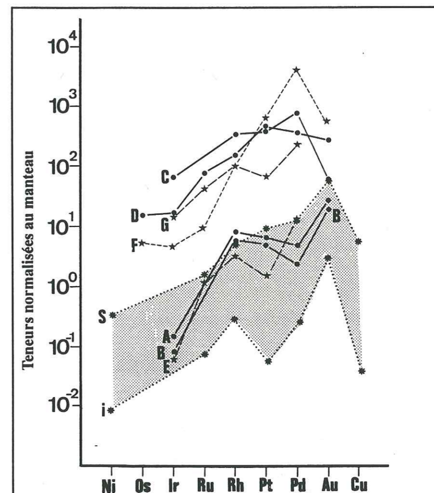
Fig. III-7: Spectres de teneur en PGE normalisées au manteau des principaux complexes stratifiés et du filon Robert A Basal Zone, bordure Figée, Bushweld ( Sharpe 1982 ) B Middle Zone, bordure Figée, Bushweld ( Sharpe 1982 ) C UG2, Bushweld ( Mc Laren et De Villers 1982 ) D Merensky Reef, Bushweld ( Hiemstra 1979 ) E Basal Zone, bordure figée, Stillwater ( Page et al. 1972 et 1976 ) F J.M. Reef, Stillwater ( Barnes 1983 ) G Chromitites, Stillwater ( Page et al. 1972 et 1976 ) I Filon Robert, limite supérieure (ce travail) S Filon Robert, limite inférieure (ce travail)
