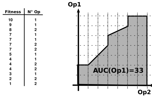
Figure 4.2 – Calcul de l’AUC pour l’opérateur op_1 .
