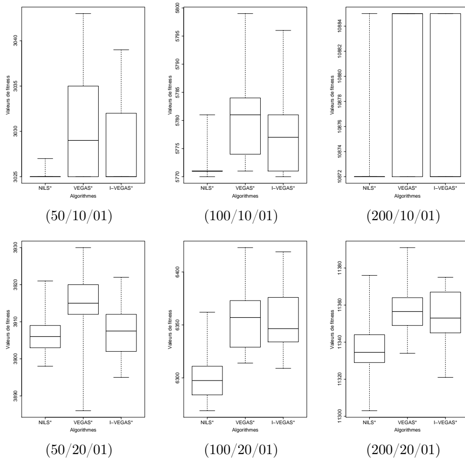
Figure 5.4 – Comparaison des performances de \text{NILS}_* , \text{VEGAS}_* et \text{I-VEGAS}_* pour les instances de Taillard, de gauche à droite, 50-, 100- 200- jobs 10- machines (haut) 20-machines (bas).
