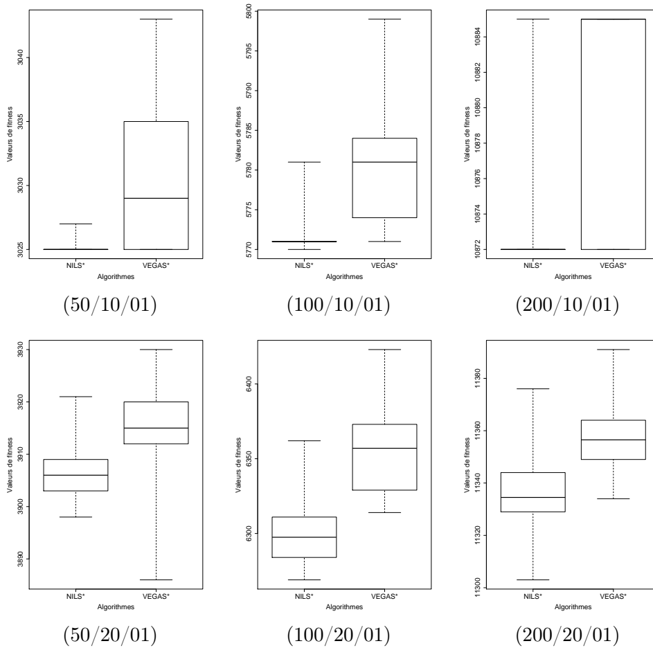
Figure 5.1 – Comparaison des performances de NLS* et VEGAS* pour les instances de Taillard, de gauche à droite, 50-, 100- 200- jobs 10- machines (haut) 20- machines (bas).
