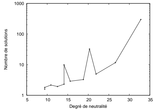
Figure 4.3 – Nombre moyen de solutions évaluées par plateaux par rapport au degré de neutralité pour VEGAS 100 .
