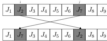
Figure 1.9 – Opérateur échange pour le problème de flowshop.
