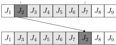
Figure 1.8 – Opérateur insertion pour le problème de flowshop.
