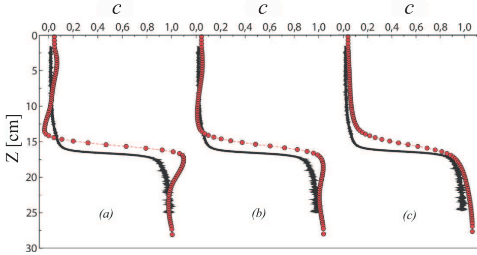
FIGURE III.9 – Variations verticales de la concentration relative c moyennées de x = 3,5 à 5,5 cm (o) au temps t_7 = 1854 s. Le facteur d'acceptance sur les paramètre est fixé à 0,001 , \lambda_f = 0,001 (a), \lambda_f = 0,02 (b), \lambda_f = 0,1 (c). La courbe noire est obtenue par l'analyse vidéo.
