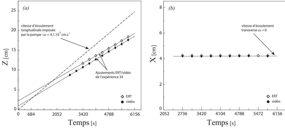
FIGURE III.28 – Evolution du centre de masse du panache de dispersion au cours de l'expérience 34 selon les directions longitudinale z en (a) et transverse x en (b) à l'écoulement pour le \text{NaCl} dissout ( \diamond ) et le colorant ( \bullet ).
