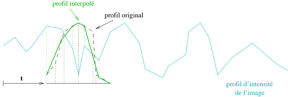
FIG. 6.9 – Interpolation linéaire des valeurs du profil de référence pour estimer la corrélation avec le profil de l'image.
