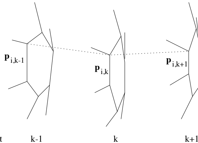
FIG. 8.1 – Trajectoire d'un sommet d'un maillage simplexe 4D entre trois instants.
