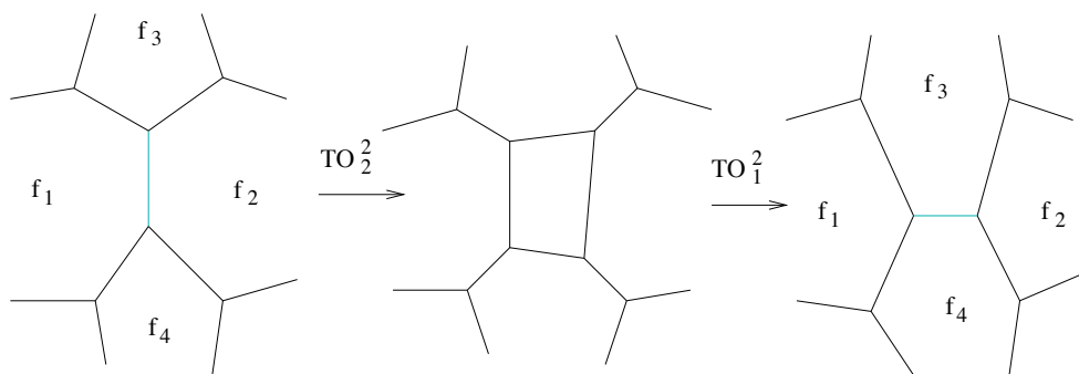
FIG. 2.15 – Opération topologique d'échange.
