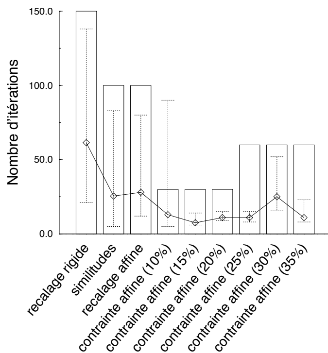
FIG. 6.32 – Nombres moyen (courbe) et maximal (histogramme) d'itérations nécessaires à la convergence du modèle à chaque étape.
