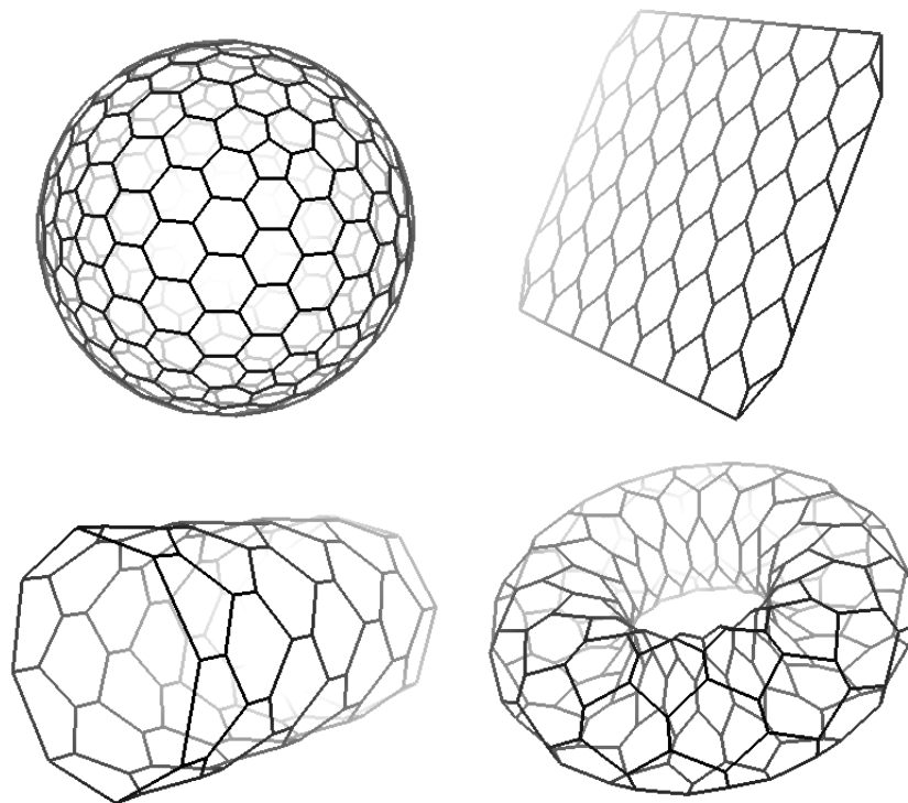
FIG. 2.5 – Quatre exemples de 2-maillages simplexes de \mathbb{R}^3 .
