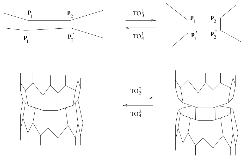
FIG. 2.22 – Opérations non-Euleriennes TO_3 et TO_4 sur les maillages simplexes.
