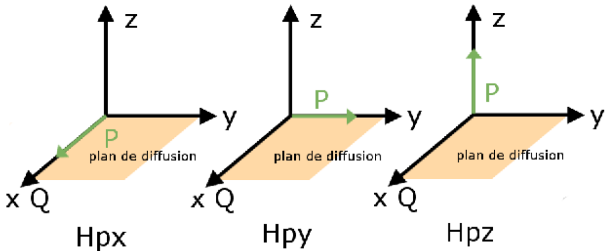
FIGURE 4.4 – Schéma des 3 configurations possibles : Hpx , Hpy , et Hpz . La polarisation en vert correspond à la direction du champ de guide H et donc à la direction des spins des neutrons. x , y et z correspondent respectivement à la direction du vecteur d'onde Q , à la direction perpendiculaire au vecteur d'onde Q dans le plan de diffusion, et à la direction perpendiculaire au plan de diffusion.
