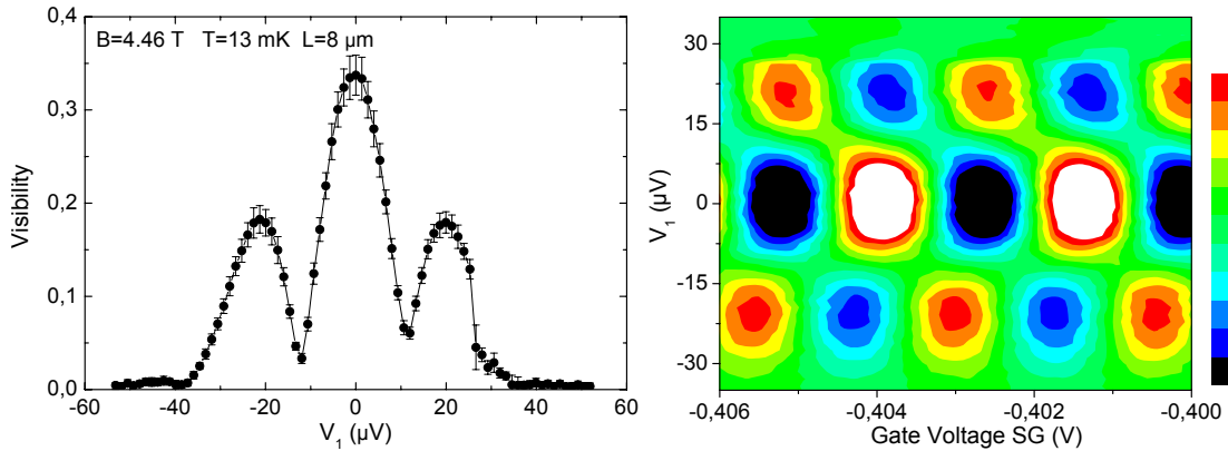
Figure 1.2.: (gauche) Visibilité décroissant avec la tension appliquée en entrée |V_1| montrant des oscillations avec de multiples extinctions pour un échantillon de longueur de bras L = 8 \mu\text{m} , à B = 4.46 \text{ T} et T = 13 \text{ mK} . Il y a deux lobes de chaque côté du lobe central. (droite) Transmission différentielle de l'état de bord externe en code couleur, en fonction de la tension de polarisation de la grille SG selon l'axe des abscisses, et en fonction de la tension V_1 sur l'axe des ordonnées. À l'intérieur d'un lobe la phase des interférences est rigide, et subit un saut de \pi aux extinctions.
