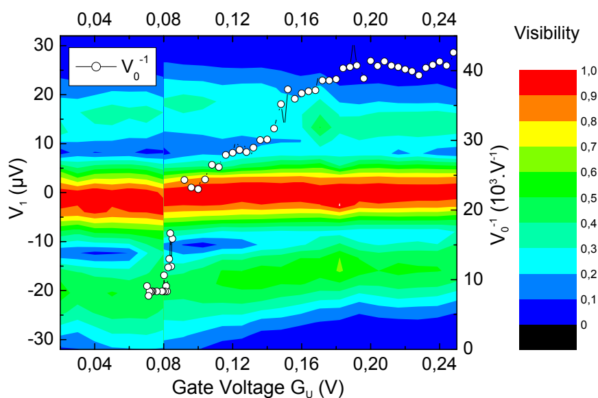
Figure 1.8.: Échelle gauche: plot couleur de la visibilité normalisée en fonction de la tension de grille V_{GU} sur l'axe des x , et de la tension de bias V_1 sur l'axe des y . Échelle droite: V_0^{-1} en fonction de V_{GU} .
