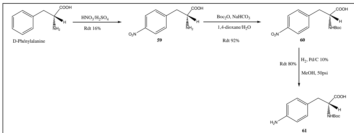
Figure 170 : Synthèse de la N ( \alpha )-Boc-4-amino-D-phénylalanine 61 .
