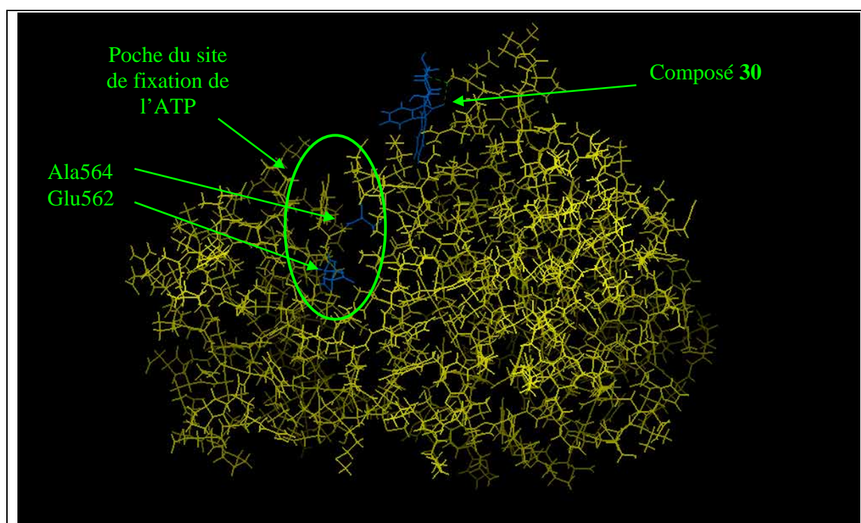
Figure 237 : Vue complète du FGFR 1 et du composé 30 .
