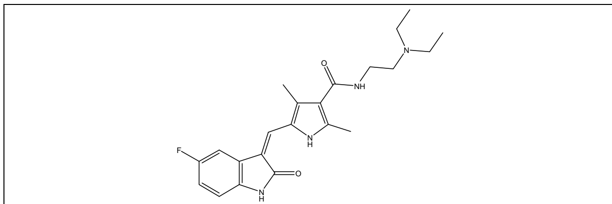
Figure 80 : Structure du SU11248.
