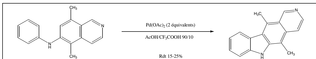
Figure 205 : Cyclisation de l'anilinoisoquinoline en présence d'acétate de palladium dans de l'acide acétique contenant 10% d'acide trifluoroacétique.
