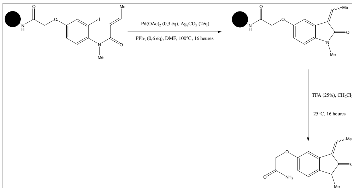
Figure 100: Synthèse d'oxindole par réaction de Heck intramoléculaire sur support solide.
