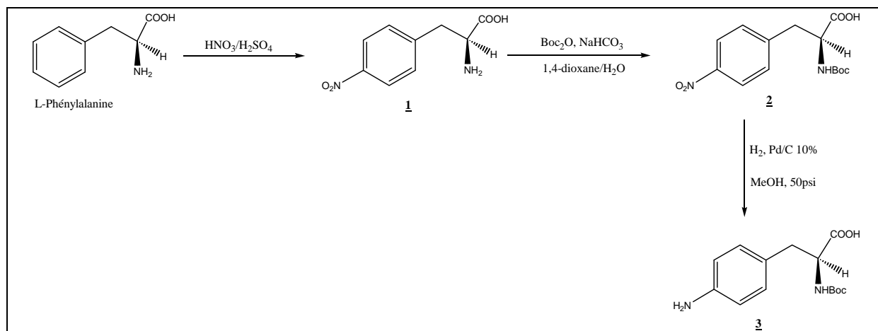
Figure 169 : Synthèse de la N ( \alpha )-Boc-4-amino-L-phénylalanine décrite par Atkinson et al.
