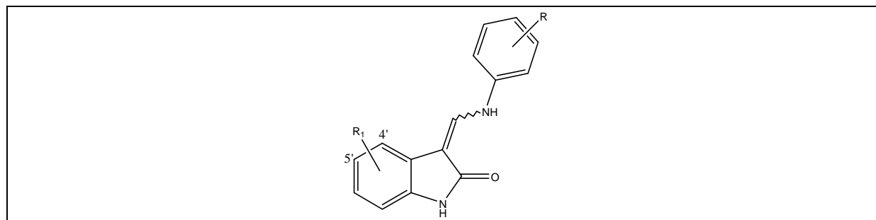
Figure 83 : Structure des composés brevetés par Allergan.
