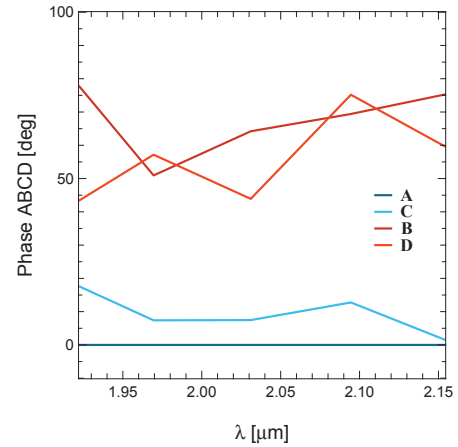
FIGURE 6.7 – Phases ABCD mesurées sur le composant 2T-ABCD en bande K. On a soustrait 180^\circ aux phases C et B afin de voir que l’opposition de phase est loin d’être parfaite. La quadrature entre les sorties AC et BD est également loin de l’idéal avec une valeur moyenne autour de 60^\circ environ.
