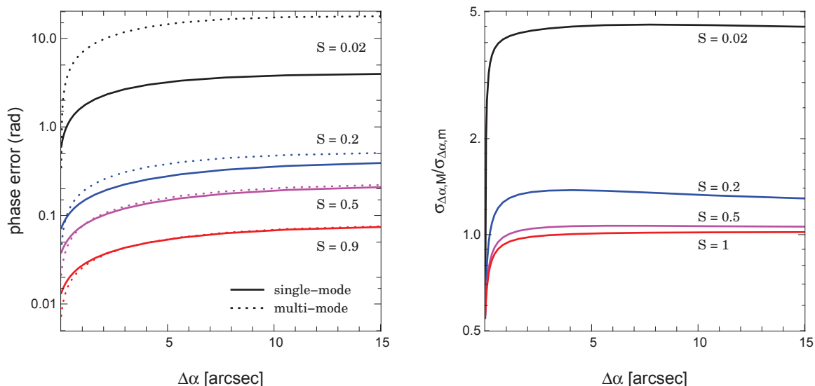
FIGURE 4.7 – Gauche – Bruit astrométrique fonction de la séparation angulaire dans les cas monomode (ligne continue) et multimode (pointillés). Droite – Rapport \sigma_{\Delta\alpha, M}^{multi} / \sigma_{\Delta\alpha, M}^{mono} . Pour les deux figures D/r_0 = 8 et on considère une unique couche turbulente située à une altitude h de 10 km.
