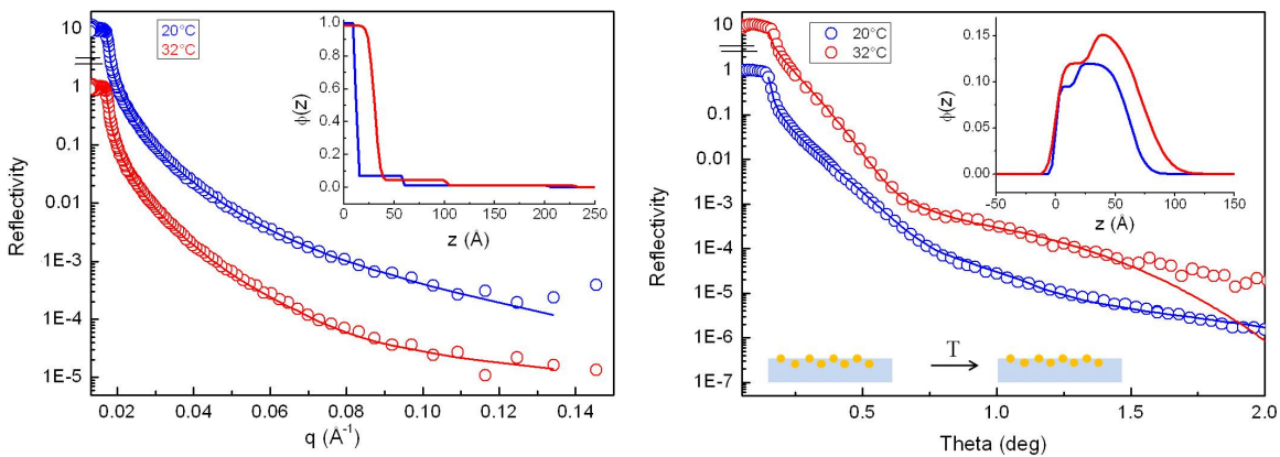
Figure 8.20: Effet de température sur la monocouche de Au-PNIPAM 127 : (a) courbes de réflectivité de neutron et (b) courbes de réflectivité de X à T = 20°C (bleu) et T = 32°C (rouge) ( 1/\text{area} = 0.00524 \text{ NPs/nm}^2 , 150 mM NaCl) (les courbes sont séparées verticalement pour une meilleure visualisation). Ligne continue = fit, insets = profils de concentration correspondants.
