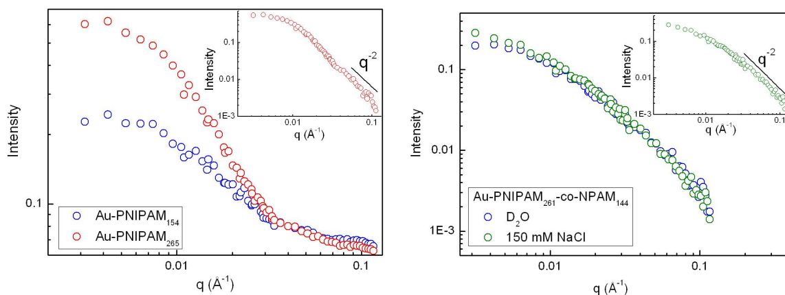
Figure 8.10: Courbes de diffusion des nanoparticules de (a) Au-PNIPAM 154 (bleu) et Au-PNIPAM 265 (rouge) dispersées dans le D 2 O et (b) Au-PNIPAM 261 -co-NPAM 144 dispersées dans le D 2 O en absence (bleu) et présence de NaCl (vert) (T = 20°C. Insets: pente en q^{-2} pour les courbes de diffusion après soustraction du bruit de fond).
