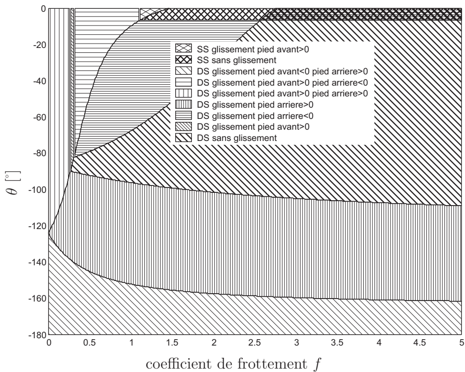
FIG. 2.10 – Comportements obtenus pour l'impact algébrique, dans le cas minimisant le coefficient de frottement nécessaire pour obtenir un double support avec l'impact différentiel.
