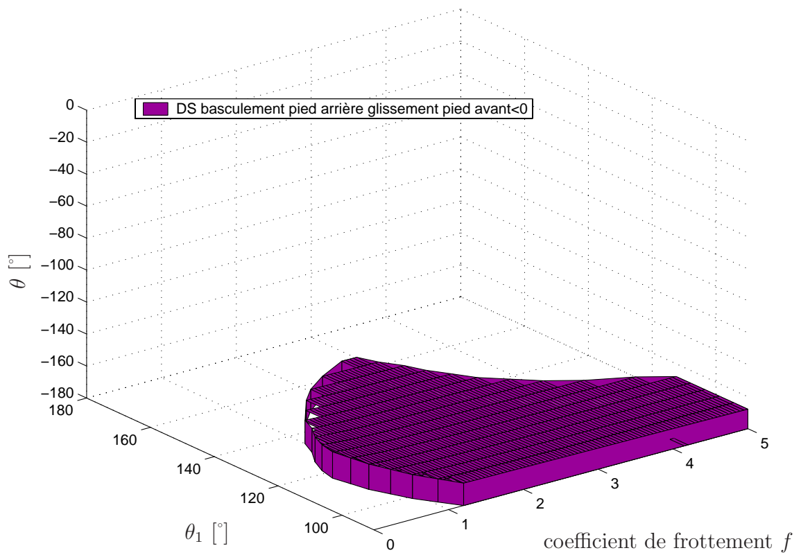
FIG. D.6 – Comportement de non glissement et basculement du pied arrière dans le cas où les deux pieds sont à plat au sol au moment de l'impact, en fonction de \theta , \theta_1 et f .
