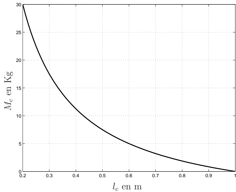
FIG. 1.10 – Relation entre la masse du contrepoids M_c et la longueur de barre à faire dépasser l_c afin que l'ensemble constitué de la barre et du contrepoids soit équivalent à l'ajout d'une masse ponctuelle sur le robot.
