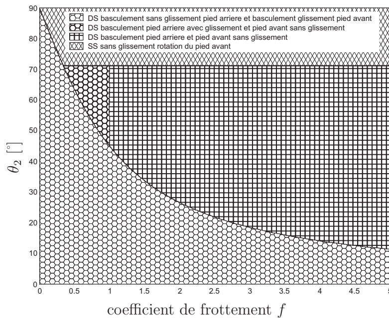
FIG. D.12 – Comportements après impact dans le cas où le pieds arrière était en basculement et le pied avant sur le talon au moment de l'impact, en fonction de \theta_2 et f pour \theta_1 = 135^\circ .
