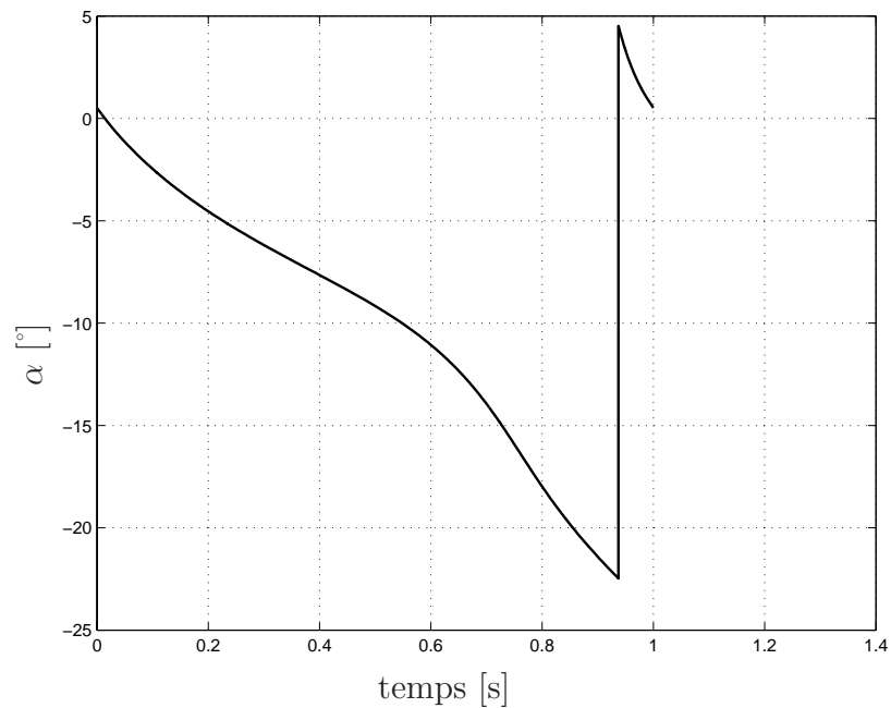
FIG. 3.14 – Evolution de \alpha en fonction du temps. Nous constatons bien qu'il a une évolution monotone, et de surcroît régulière.
