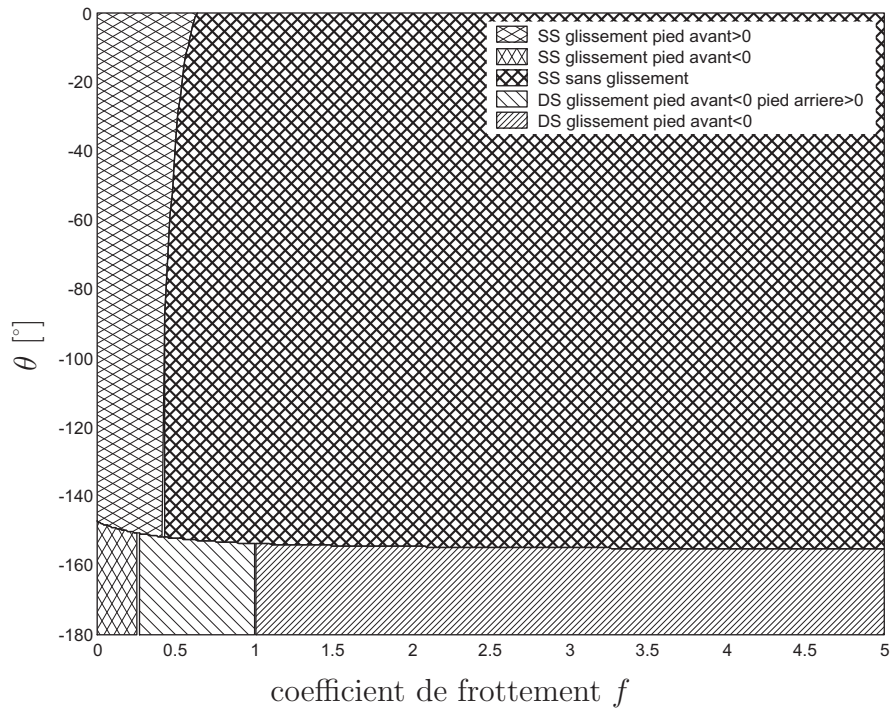
FIG. 2.14 – Comportements du modèle différentiel, obtenus pour la configuration la plus proche de la configuration de marche présentée figure 2.2 et pour laquelle un double support est possible pour un coefficient de frottement de 1 avec le modèle algébrique.
