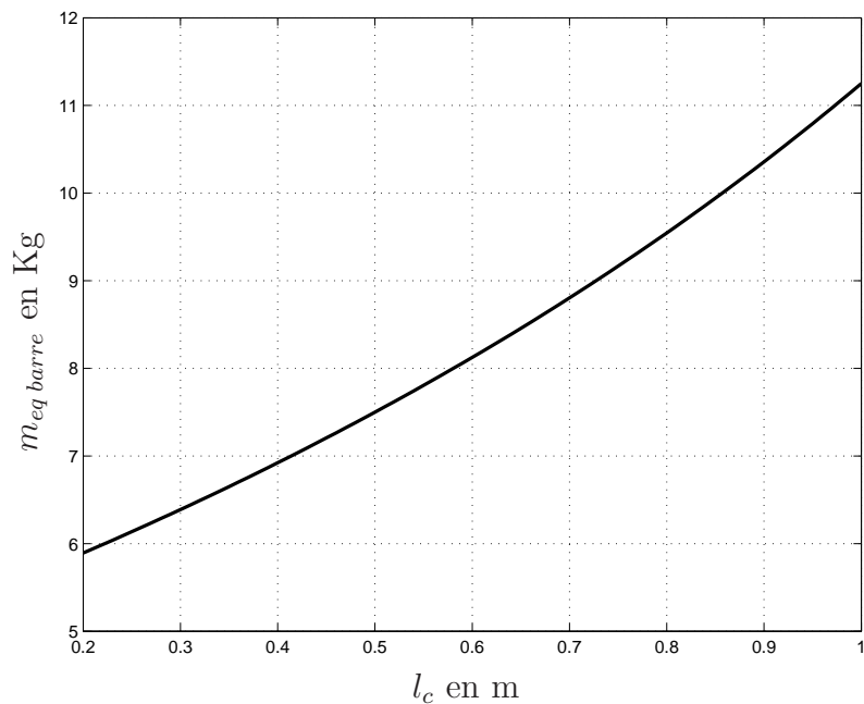
FIG. 1.11 – Relation entre la masse équivalente au niveau du point d'attache de la barre et la longueur de barre qui dépasse l_c . La masse du contrepoids M_c est celle déterminée afin que l'ensemble constitué de la barre et du contrepoids soit équivalent à l'ajout d'une masse ponctuelle sur le robot.
