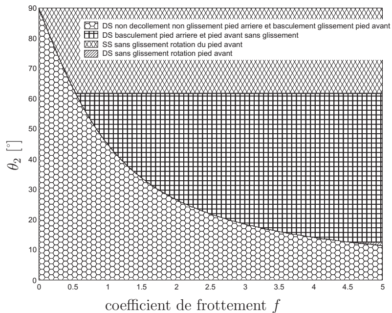
FIG. D.11 – Comportement de non glissement et basculement des deux pieds dans le cas où le pied arrière était à plat et le pied avant sur le talon au moment de l'impact, en fonction de \theta_2 et f pour \theta_1 = 118,35^\circ .
