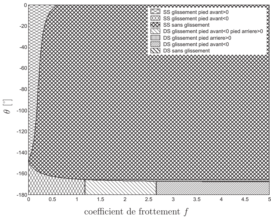
FIG. 2.3 – Comportements obtenus avec le modèle d'impact algébrique pour la configuration de marche.
