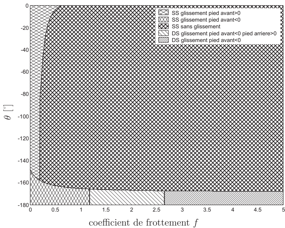
FIG. 2.5 – Comportements obtenus avec le modèle d'impact différentiel pour la configuration de marche.
