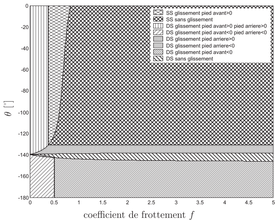
FIG. 2.7 – Comportements obtenus pour l'impact algébrique, dans le cas minimisant le coefficient de frottement nécessaire pour obtenir un double support avec l'impact algébrique.
