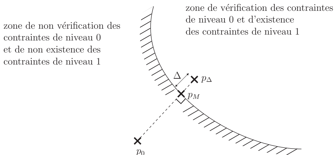
FIG. 3.7 – Représentation du vecteur de paramètres d'origine p_0 ne vérifiant pas les contraintes de niveau 0, et sa projection p_M sur la frontière du domaine de vérification des contraintes de niveau 0. Le point p_\Delta utilisé pour le calcul par prolongement du critère et des contraintes en p_0 est également représenté.
