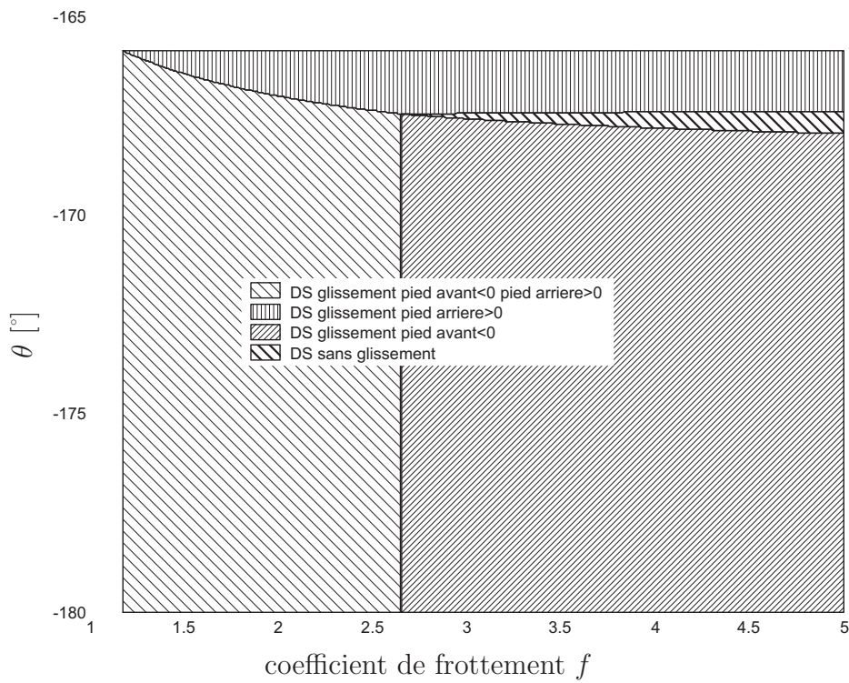
FIG. 2.4 – Comportements obtenus avec le modèle d'impact algébrique pour la configuration de marche, zoom sur la zone de double support.
