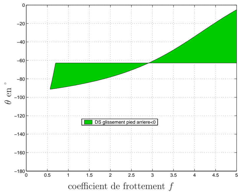
FIG. B.3 – Représentation de la zone de double support avec glissement du pied arrière en fonction de \theta et f dans le cas d'une indétermination.
