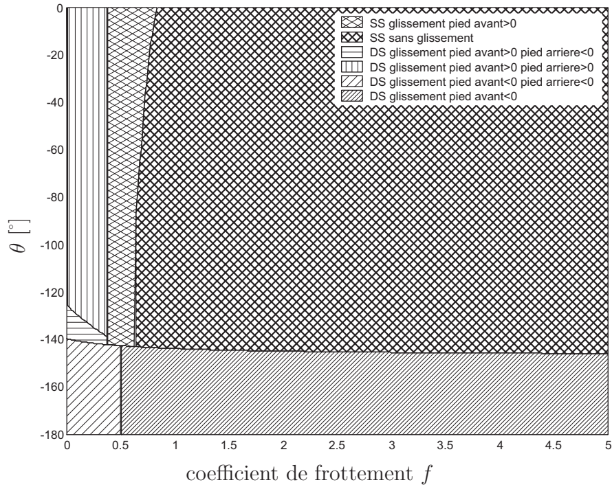
FIG. 2.8 – Comportements obtenus pour l'impact différentiel, dans le cas minimisant le coefficient de frottement nécessaire pour obtenir un double support avec l'impact algébrique.
