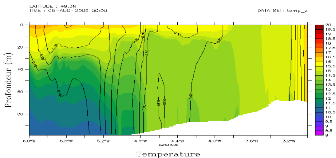
(a) 09.08.2009, coupe Manche
