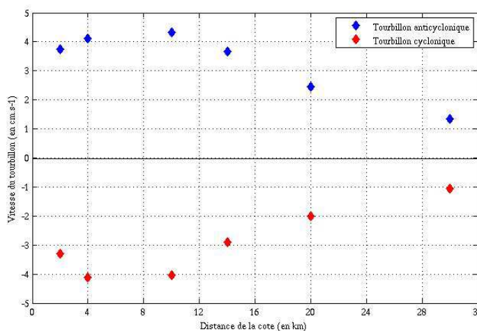
FIGURE 2.9 – Vitesse d'advection des tourbillons en fonction de leur distance à la côte
