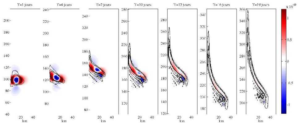
FIG. 4.22: Critère d'Okubo-Weiss (couleur) et contours de PVA pour (\Delta Q^0 = 0,5 ; R_t = 5 \text{ km} ; D_c = 14 \text{ km}) .
