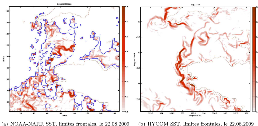
FIG. 5.11: Gradients de température obtenu par la méthode de Scharr pour les images NOAA-NAAR SST et les sorties modèle.
