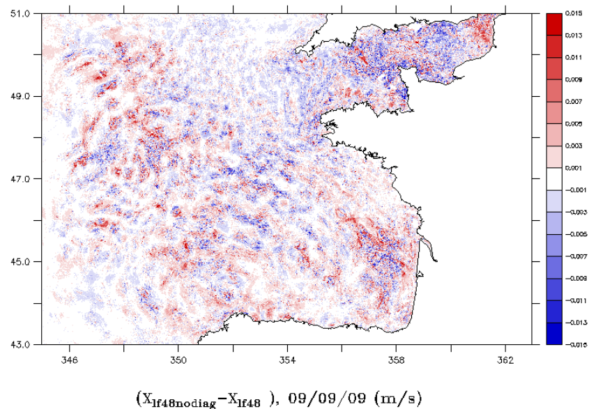
FIG. 5.20: Erreur sur le résidu basse fréquence en surface après filtrage optimisé sur 48h sans diagnostique préalable par rapport au cas référence avec diagnostique, en m/s (09 septembre 2009)
