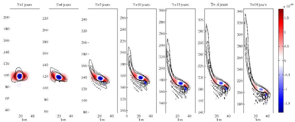
FIG. 4.21: Critère d'Okubo-Weiss (couleur) et contours de PVA pour (\Delta Q^0 = 0,5 ; R_t = 5 \text{ km} ; D_c = 20 \text{ km}) .
