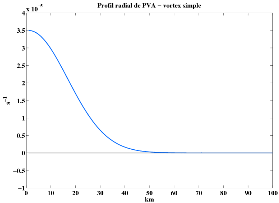
FIG. 4.5: Profil radial de PVA du vortex prescrit dans la première couche, vortex cyclonique ( \Delta Q^0 = 0,5 \times f = 3,5 \cdot 10^{-5} s^{-1} , R_t = 11 km )
