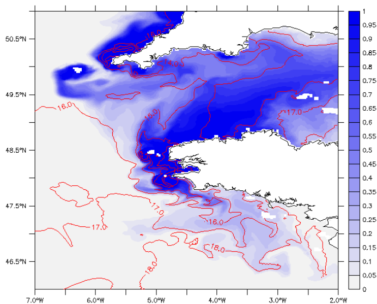
Traceur global T=21799, Surface
