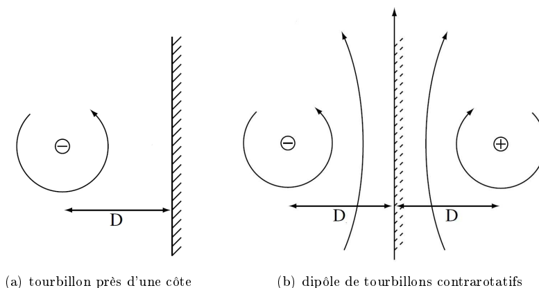
FIGURE 2.8 – Un tourbillon initial près d'une côte 2.8(a), auquel on rajoute un compagnon virtuel image, se comporte comme un dipôle de tourbillons contrarotatifs 2.8(b)
