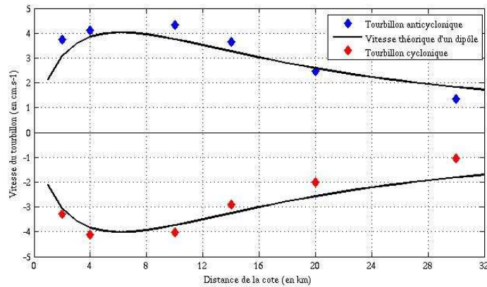
FIGURE 2.10 – Vitesse de translation d'un dip ole de tourbillons contrarotatifs
