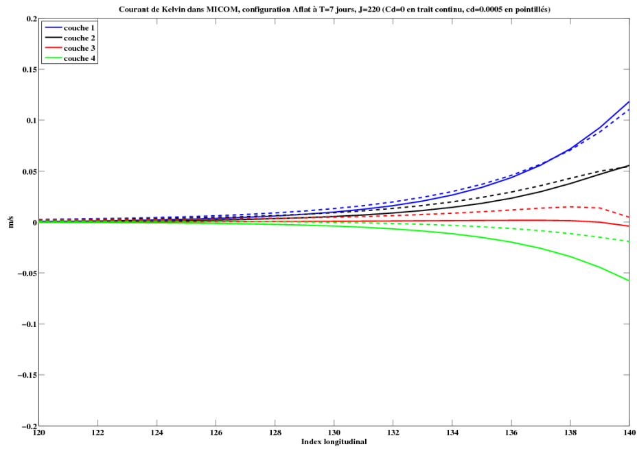
FIG. 4.4: Profil de vitesse vertical observée dans le cas Aflat, à la latitude J=220 ( Y=440\text{km} ) à T=7 jours sans friction (trait continu) et avec Cd = 0.0005 (pointillés). Après 7 jours le courant est installé et n'est pas encore perturbé. L'inhibition de la dynamique dans la couche 4 est rééquilibrée par une augmentation de la vitesse dans la couche 3, tandis que les vitesses dans les deux premières couches ne sont pas significativement modifiées.
