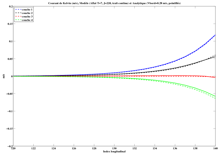
FIG. 4.3: Profil de vitesse vertical observée dans le cas Aflat, à la latitude J=220 ( Y=440\text{km} ) à T=7 jours (trait continu) et calculé analytiquement (pointillés) avec une condition V_{bord} = 0.28\text{m/s} . Après 7 jours le courant est installé et n'est pas encore perturbé. Le modèle analytique d'un courant barocline de gradient de PV constant est en accord avec la sortie modèle, confirmant qu'il s'agit d'un courant de gravité barocline de PVA nulle.
