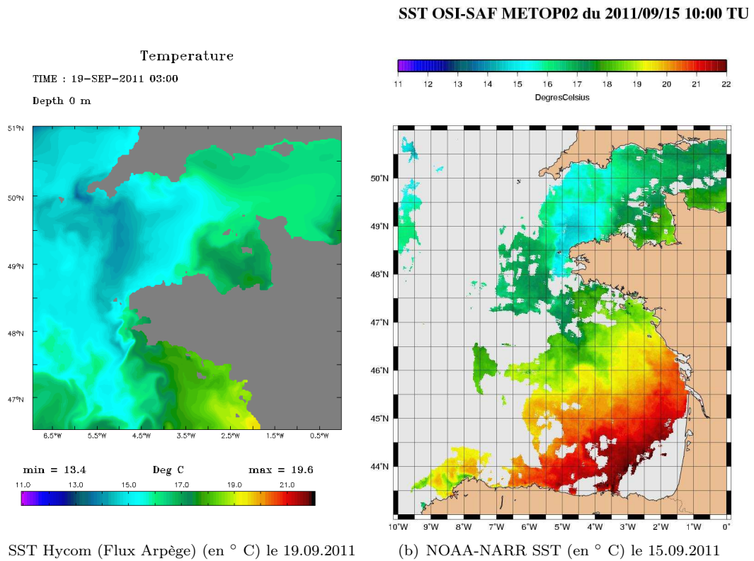
FIG. 5.59: Champ de température de surface dans Hycom (flux Arpège) et image satellite OSI-SAF correspondante le 15/09/2011
