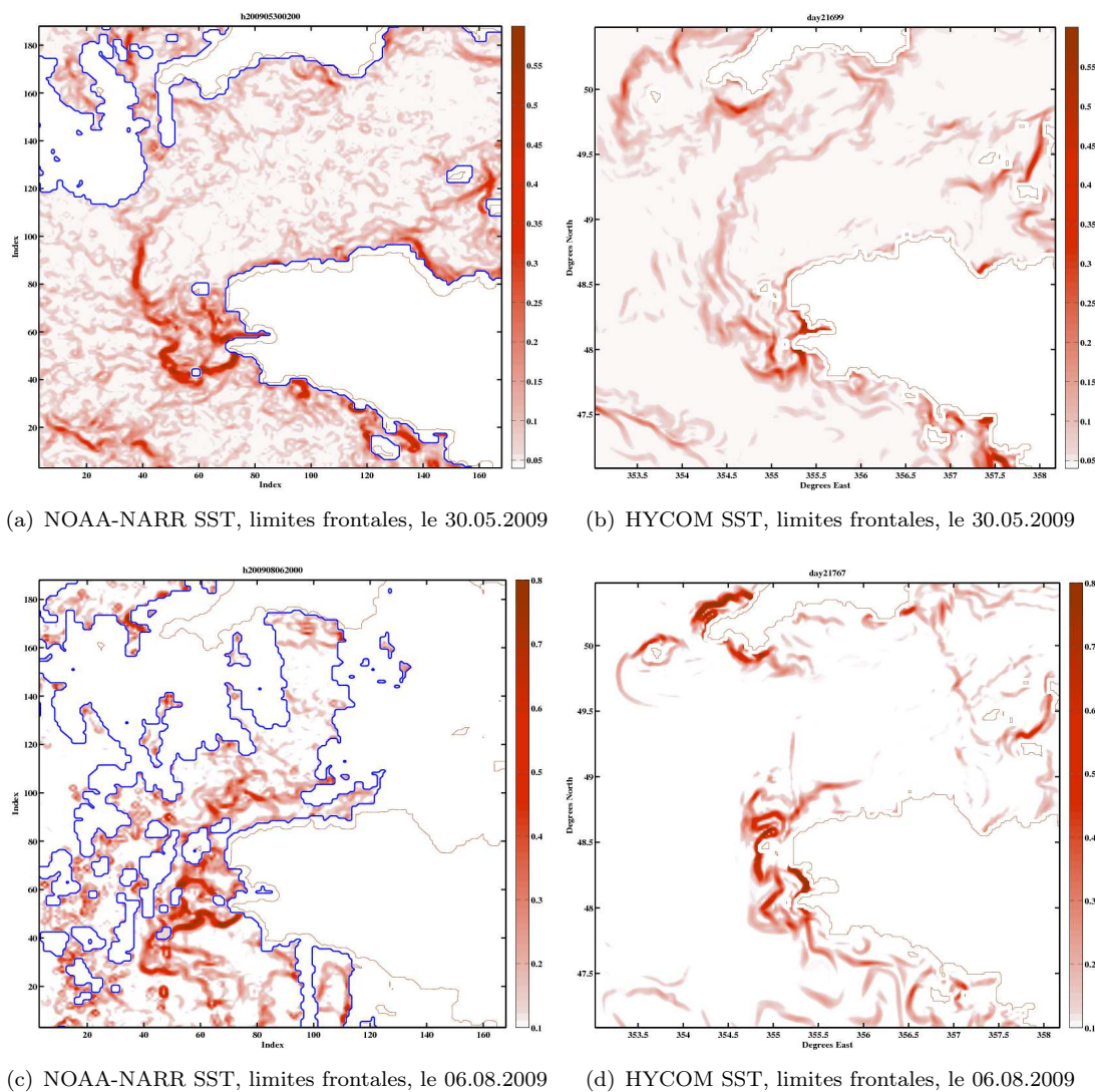
FIG. 5.9: Gradients de température obtenu par la méthode de Scharr pour les images NOAA-NAAR SST et les sorties modèle.
