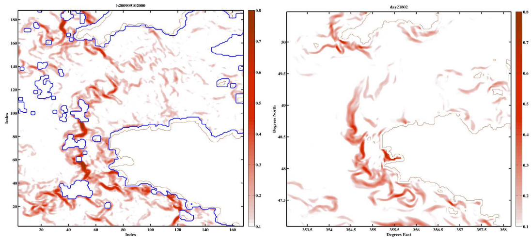
(a) NOAA-NARR SST, limites frontales, le 10.09.2009
