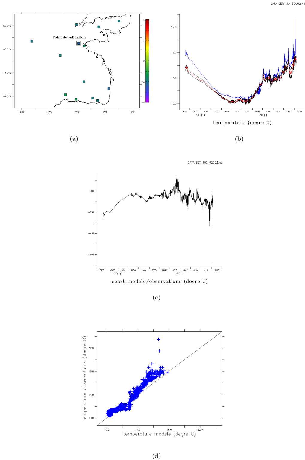
FIG. 5.8: Comparaison de SST de modèle HYCOM avec flux Arpegge et données in-situ
