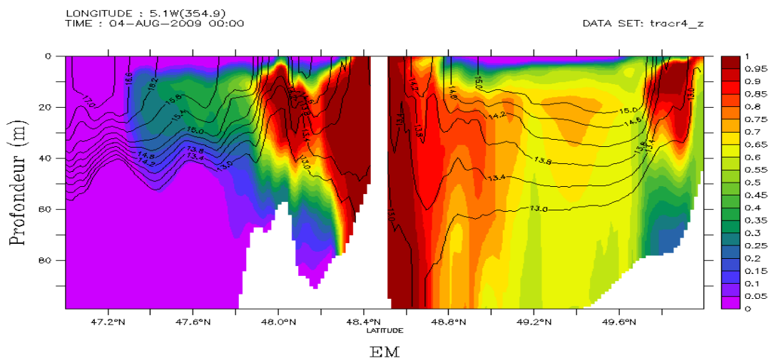
(b) coupe X=5.08W,Y=47N :50N, Tr_{global} et contours de température
