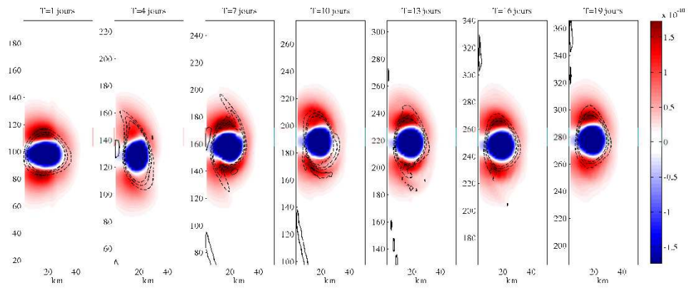
FIG. 4.20: Critère d'Okubo-Weiss (couleur) et contours de PVA dans la configuration C_{0-} .
