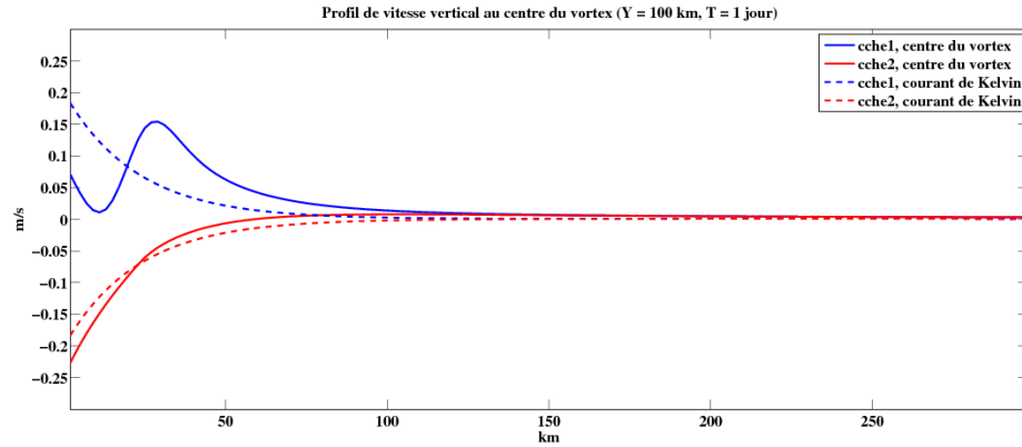
FIG. 4.8: Profil de courant, configuration de référence C_{0+} , vortex cyclonique
