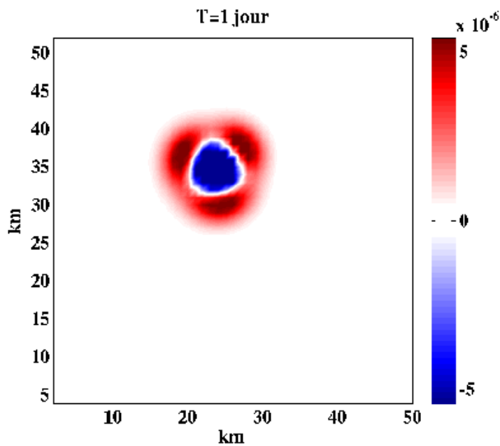
FIG. 4.12: PVA du vortex en couronne prescrit dans la première couche pour l'étude d'advection par le courant barocline, vortex anticyclonique ( \Delta Q^0 = -0,5 \times f = 3,5 \cdot 10^{-5} \text{ s}^{-1} , R_t = 11 \text{ km} ). La couronne de PVA positive autour du centre de PVA négative tend à se séparer en trois pôles positifs.
