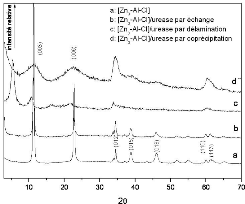
Figure 4 : Diffactogrammes X a) précurseur [Zn 3 -Al-Cl], b) phase échangée, c) phase délaminée-reconstruite, d) phase coprécipitée.
