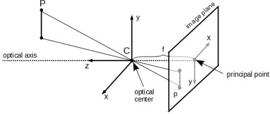
FIGURE 3.21 – Modèle de projection sténopée de la caméra.
