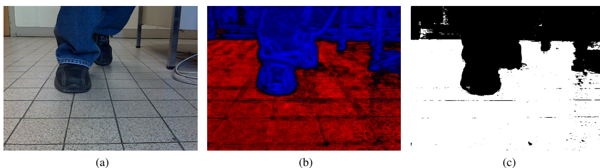
FIGURE 3.18 – Détection d'obstacles basée sur des attributs de couleur et de texture pour une scène comportant un piéton considéré comme un obstacle pour la méthode, (a) l'image originale, (b) l'image de probabilité de détection d'obstacles et (c) l'image binaire de détection d'obstacles
