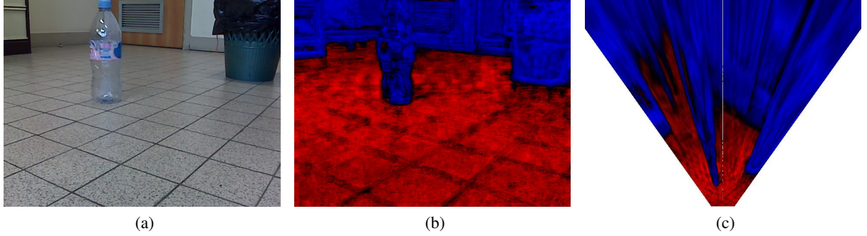
FIGURE 3.28 – Projection vers le sol de la détection d'obstacles obtenue à partir des attributs de la couleur et de la texture. Cette image a été acquise depuis une scène comprenant une bouteille en plastique et une poubelle qui sont considérées comme des obstacles pour la méthode de détection, (a) l'image originale, (b) l'image de probabilité de détection d'obstacles et (c) sa projection correspondante vers le sol.
