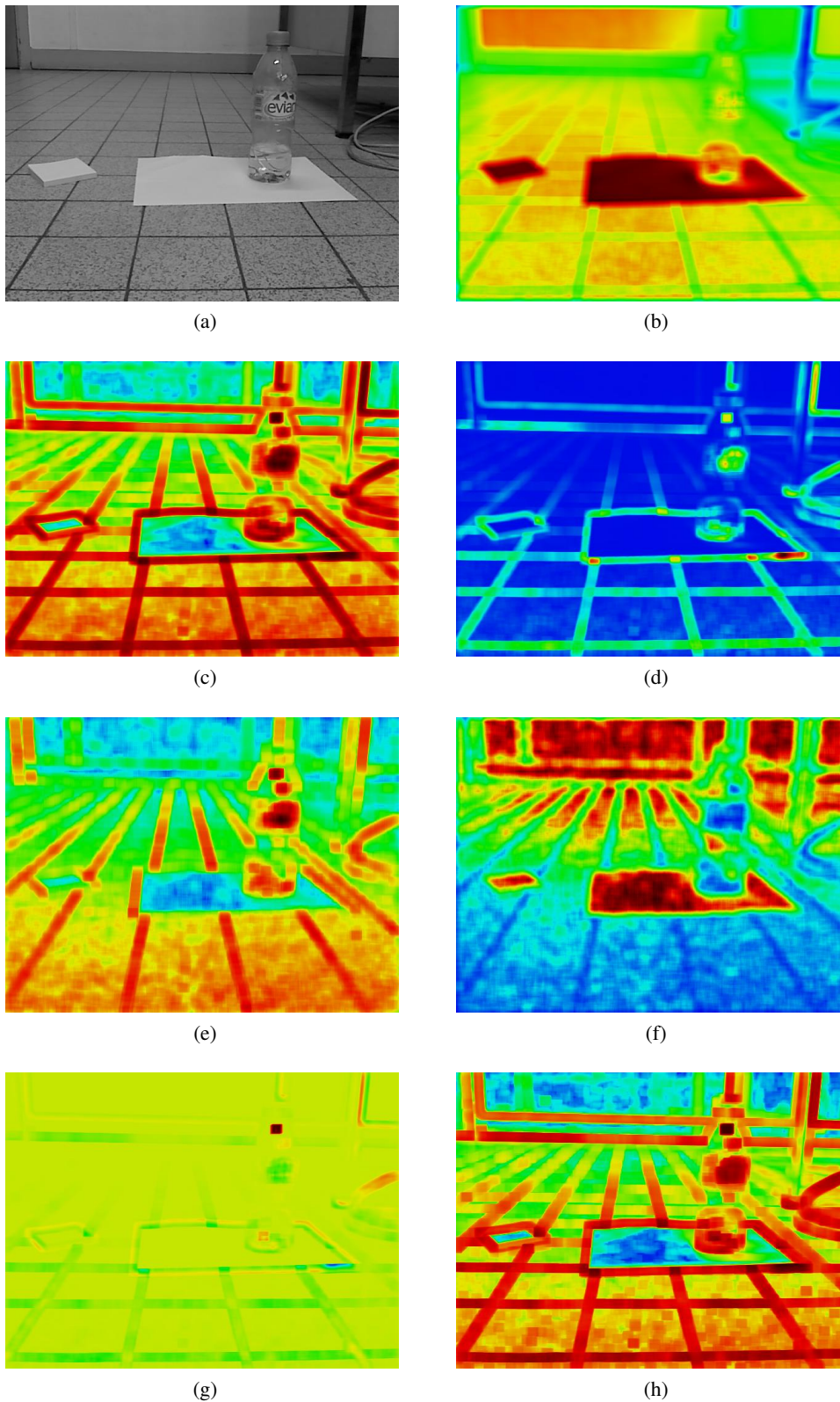
FIGURE 3.6 – Calcul des attributs de texture pour un déplacement de (-1, 0) . (a) Image d'origine, Images des attributs de la texture de (b) Moyenne, (c) Variance, (d) Corrélation, (e) Contraste, (f) Homogénéité, (g) Cluster de Nuance, (h) Cluster de Proéminence.
