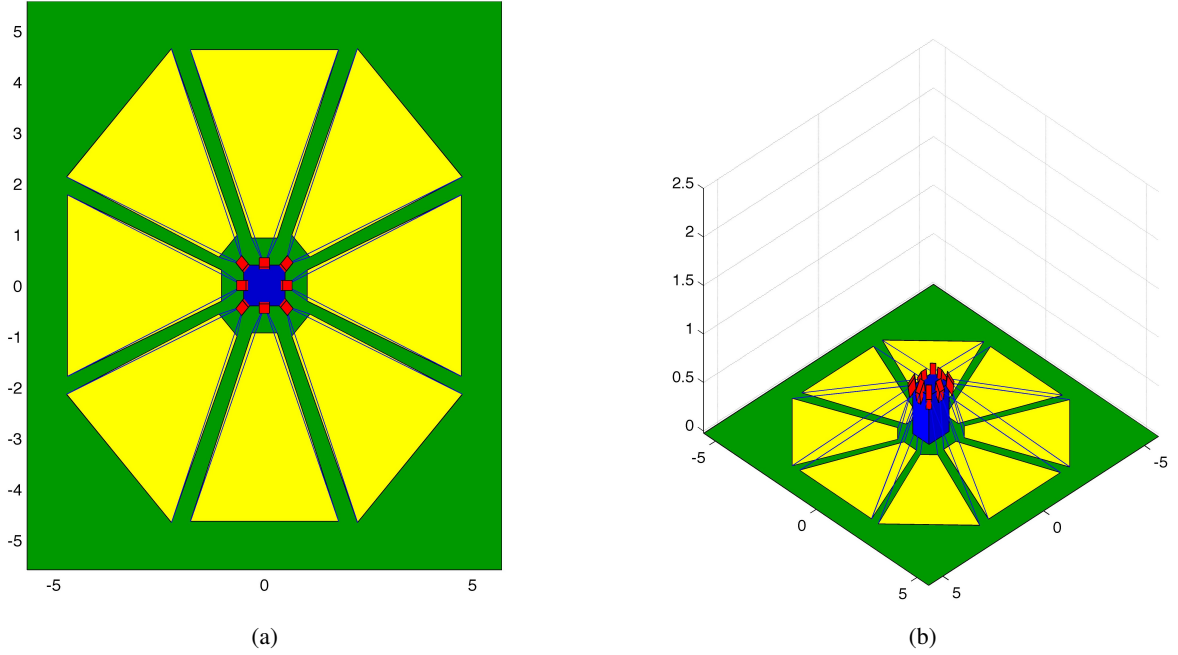
FIGURE 3.2 – Simulation de la zone couverte par la ceinture de micro-caméras placée autour du robot, (a) vue d'en haut, (b) vue à partir de 45^\circ
