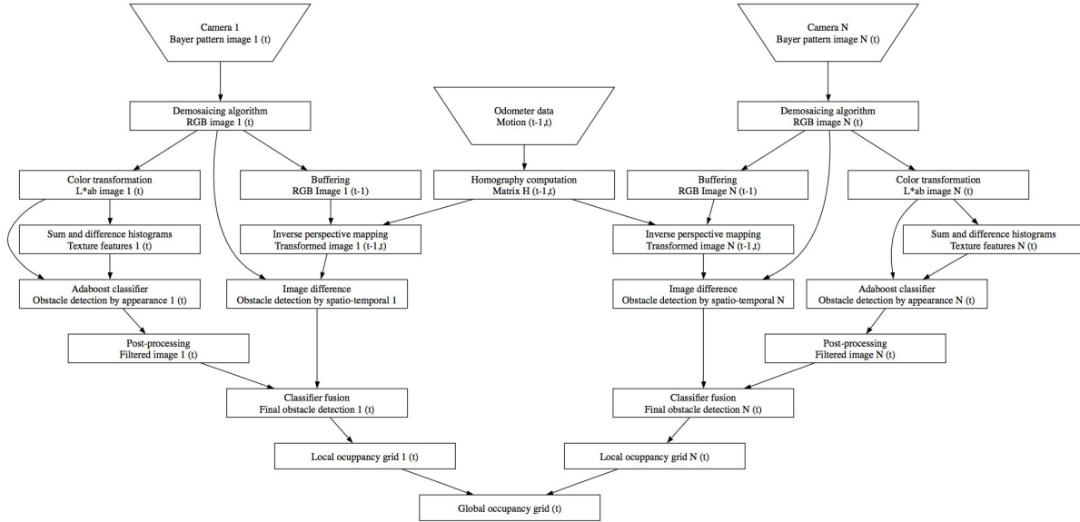
FIGURE 3.1 – Diagramme global de l'algorithme pour la détection d'obstacles.
