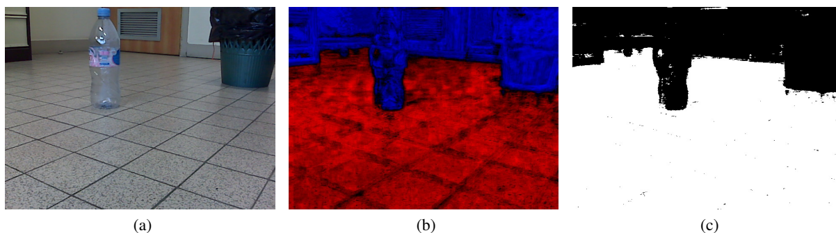
FIGURE 3.17 – Détection d'obstacles basée sur des attributs de couleur et de texture pour une scène avec une bouteille considérée comme un obstacle pour la méthode, (a) l'image originale, (b) l'image de probabilité de détection d'obstacles et (c) l'image binaire de détection d'obstacles
