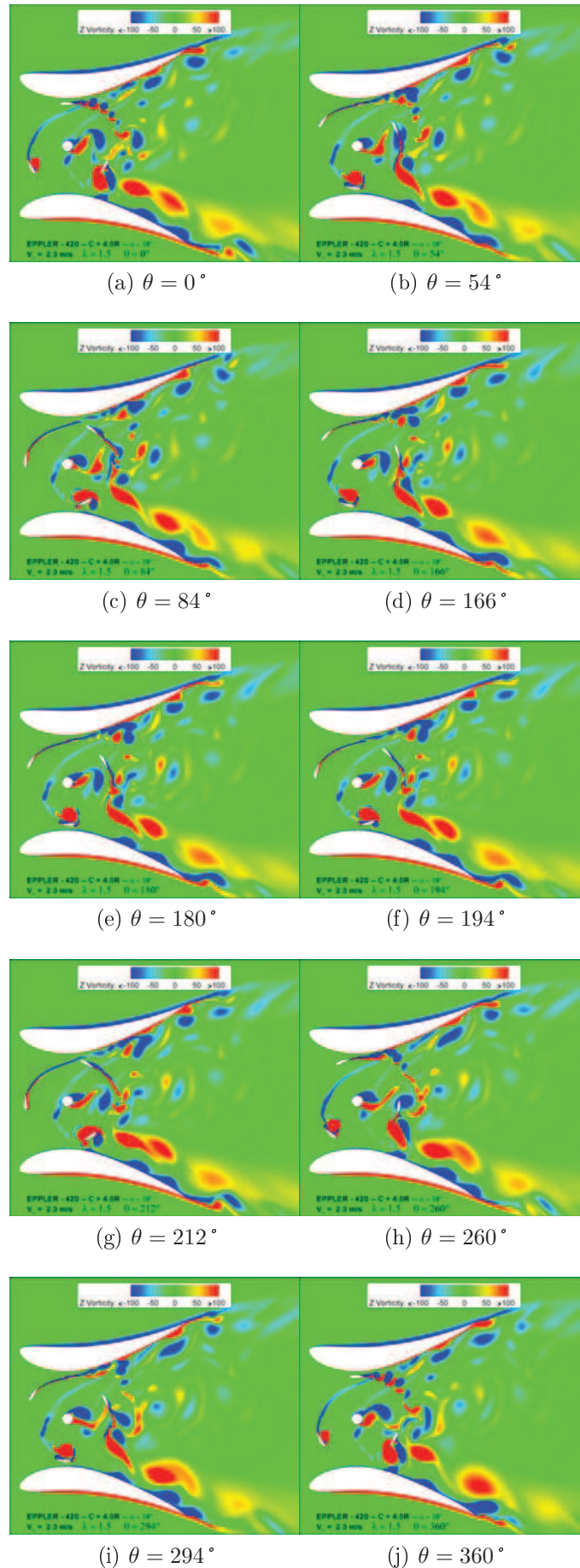
FIG. I.2: Cartes de vorticité instantannées . \lambda = 1.5 .
