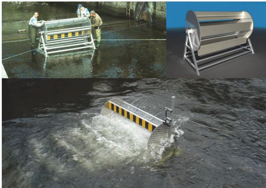
FIG. 1.4: Hydrolienne à flux transverse [Source : Atlantisstrom™, www.atlantisstrom.de].
