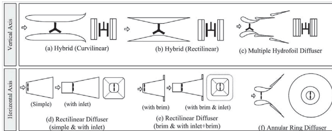
FIG. 1.9: Vue schématique de différents types de carénage. Pour chaque configuration une vue de dessus et une vue de face sont présentées. La Flèche indique le flux entrant.
