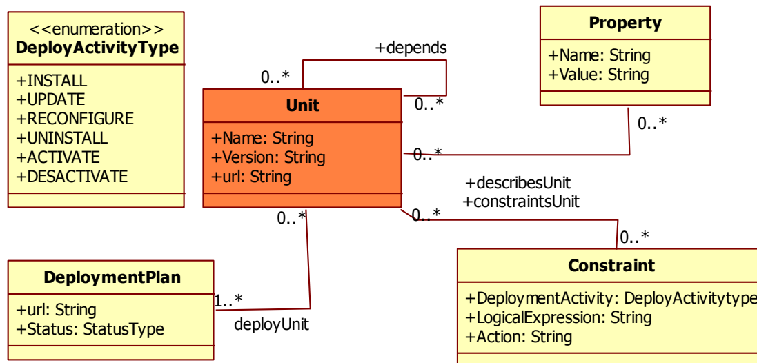
Figure 4 : Le méta-modèle ORYA
