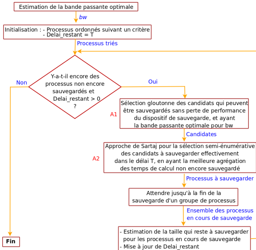
FIGURE 5.2 – Diagramme du schéma d'approximation
