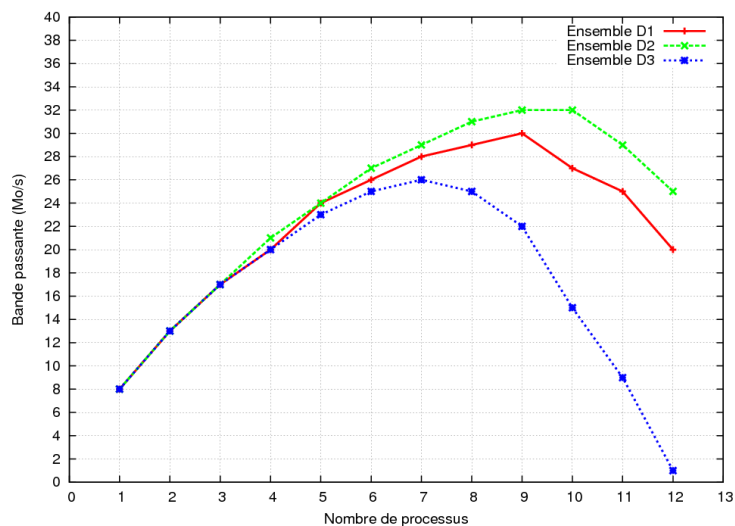
FIGURE 4.13 – Bandes passantes expérimentales
