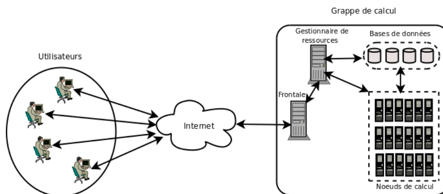
FIGURE 2.3 – Architecture générale des environnements de calcul de type grappe
