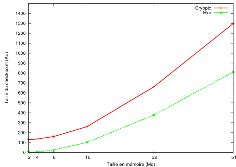
FIGURE 3.5 – Taille du point de reprise généré par BLCR et Cryopid sur le code Mandelbrot
