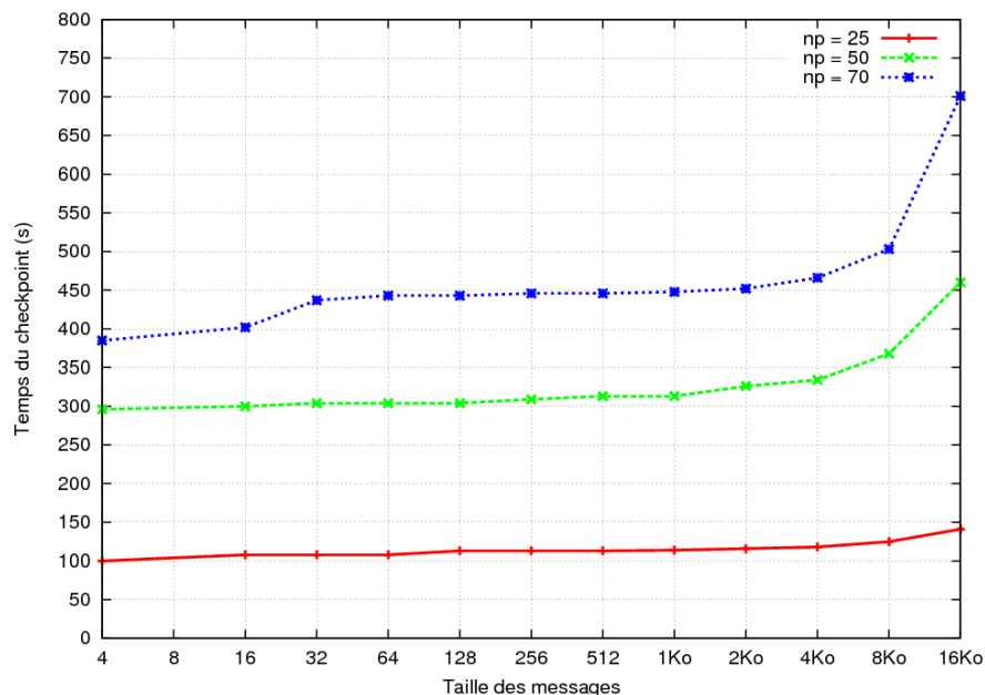
FIGURE 4.15 – Comparaison des temps de sauvegarde d'une application parallèle pour différentes tailles des messages dans les canaux de communication
