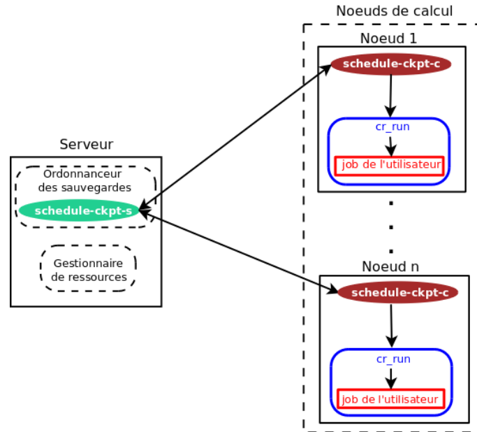
FIGURE 6.2 – Architecture de l'ordonnanceur des sauvegardes
