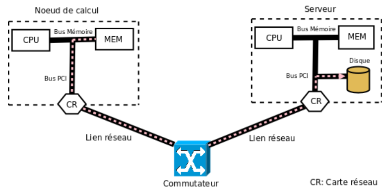
FIGURE 4.1 – Chemin d'une sauvegarde
