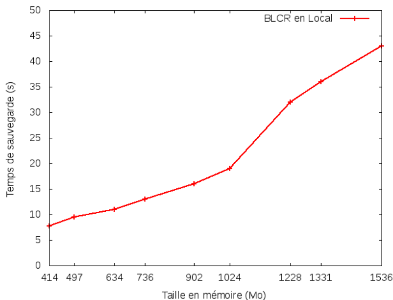
FIGURE 3.1 – Temps de sauvegarde en fonction du volume de données à sauvegarder : cas d'une application séquentielle
