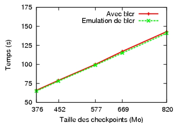
FIGURE 4.9 – Temps de sauvegarde du code de calcul multigrilles avec BLCR et par émulation de BLCR, à distance
