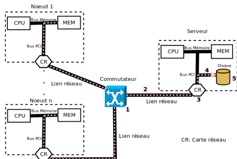
FIGURE 4.2 – Sauvegarde en parallèle
