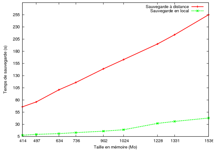
FIGURE 3.3 – Temps de sauvegarde en fonction de la proximité du support de sauvegarde
