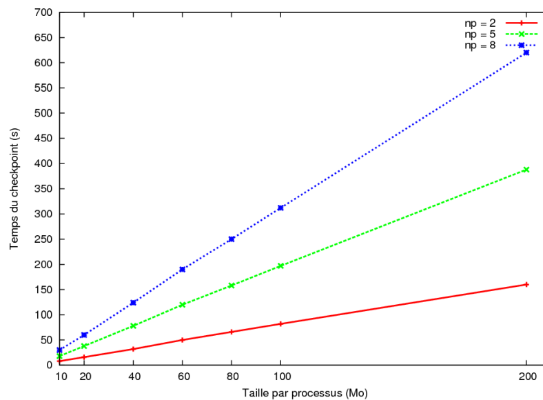
FIGURE 3.2 – Temps de sauvegarde en fonction du volume de données à sauvegarder : cas d'une application parallèle
