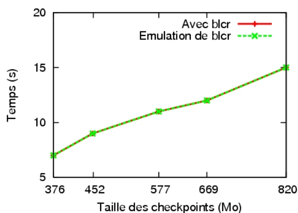
FIGURE 4.8 – Temps de sauvegarde du code de calcul multigrilles avec BLCR et par émulation de BLCR, en local
