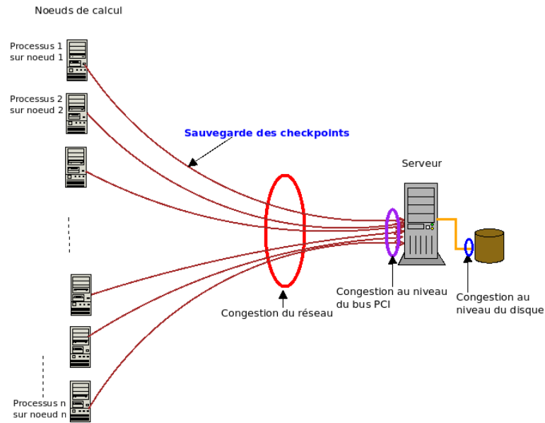
FIGURE 3.8 – Sauvegarde d'applications séquentielles avant restitution des ressources
