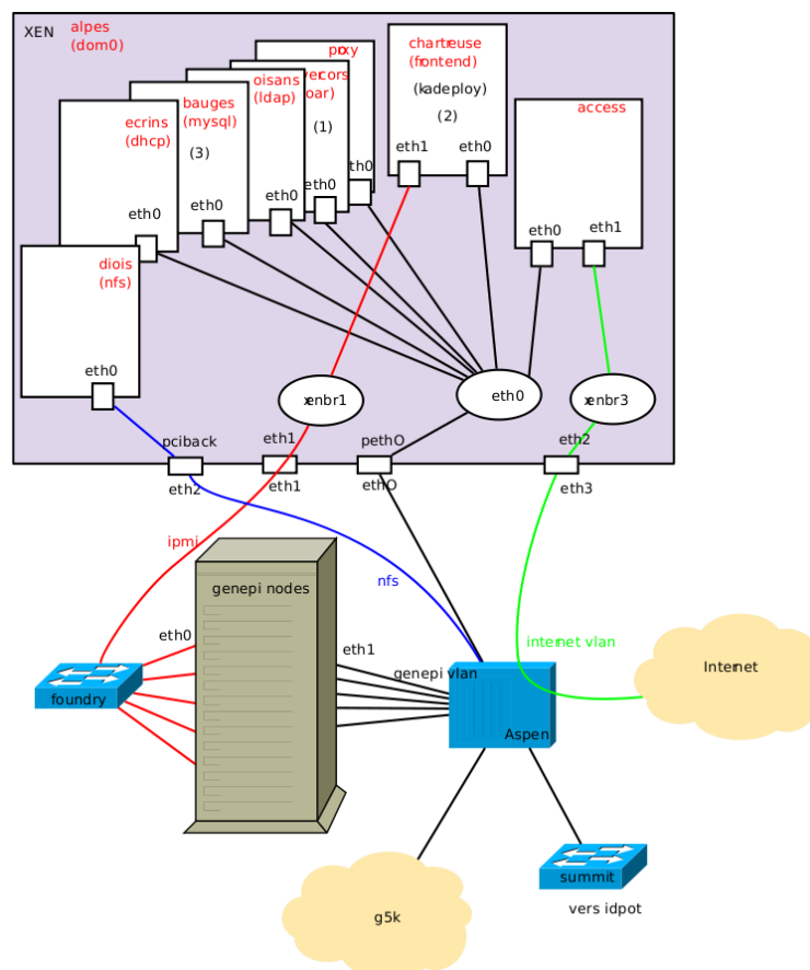
FIGURE B.1 – Placement des services sur des machines virtuelles au niveau du serveur d’une grappe de Grid5000 ( source : https://gforge.inria.fr/projets/grid5000 )
