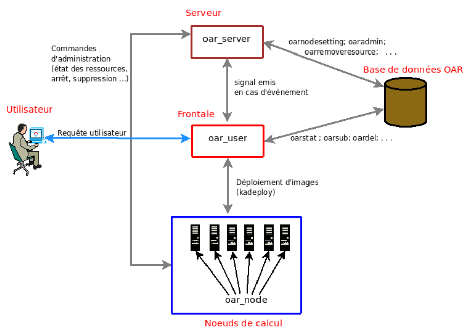
FIGURE 6.1 – Fonctionnement de OAR dans une grappe
