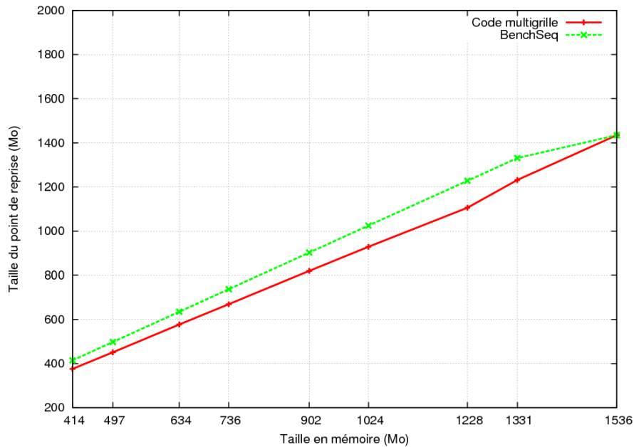
FIGURE 4.6 – Tailles du points de reprise générés par BLCR pour deux applications différentes occupant le même volume en mémoire
