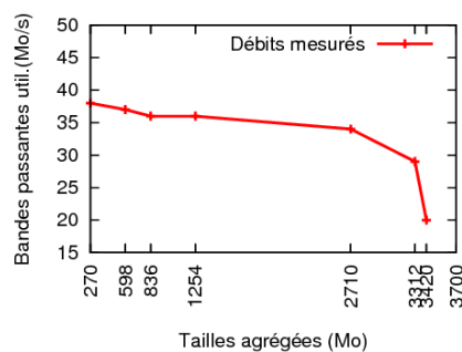
FIGURE 4.11 – Bande passante utilisée en fonction de V
