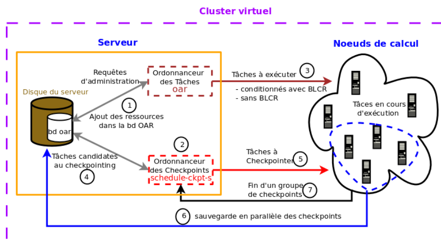
FIGURE 6.3 – Grappe virtuelle avec OAR et l'ordonnanceur des sauvegardes
