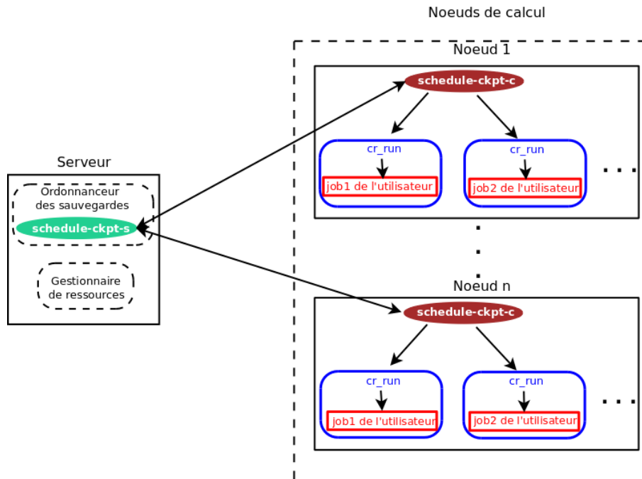
FIGURE 6.6 – Architecture étendue de l'ordonnanceur des sauvegardes
