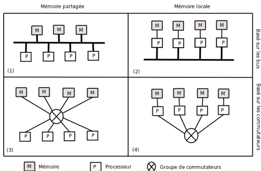
FIGURE 2.1 – Classification de Tanenbaum des architectures de machines de type MIMD
