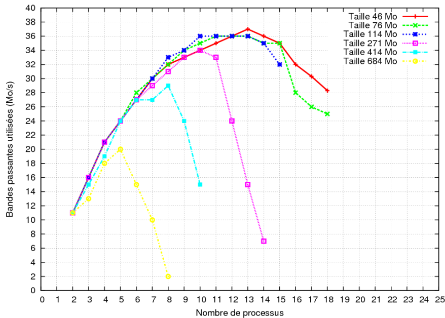
FIGURE 4.10 – Bande passante utilisée en fonction du nombre de processus selon la taille des applications
