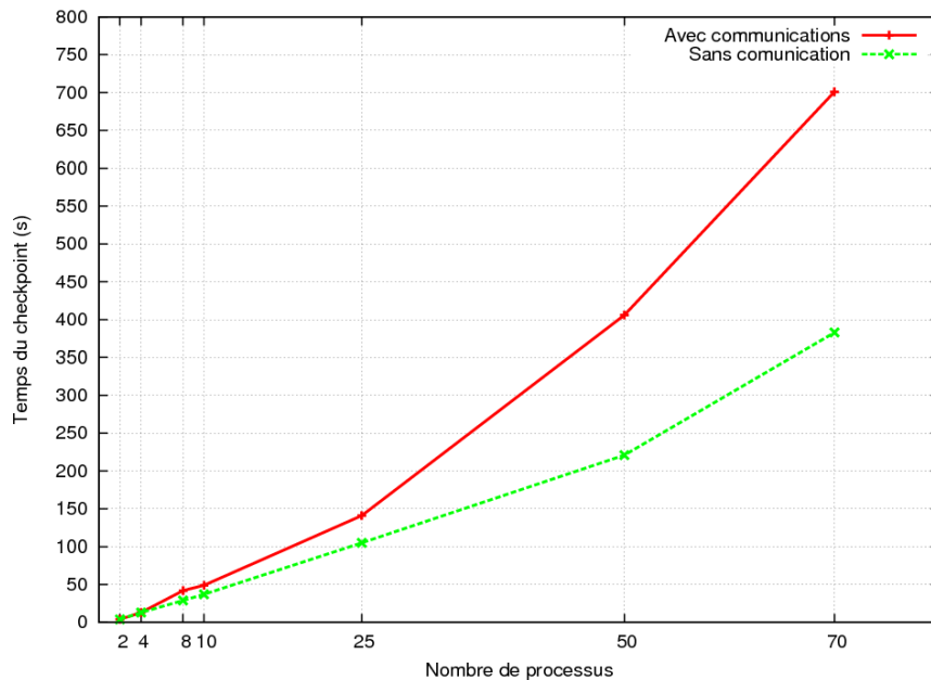
FIGURE 4.16 – Comparaison des temps de sauvegarde de deux applications parallèles dont l'une a des messages dans les canaux de communication
