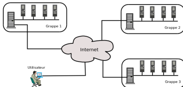
FIGURE 2.2 – Architecture générale des environnements de calcul de type grille
