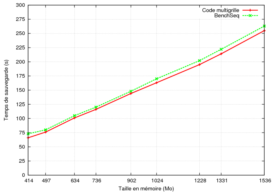
FIGURE 4.7 – Temps de sauvegarde correspondants
