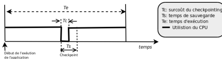
FIGURE 3.6 – Séquence de prise de point de reprise au cours de l'exécution d'une application
