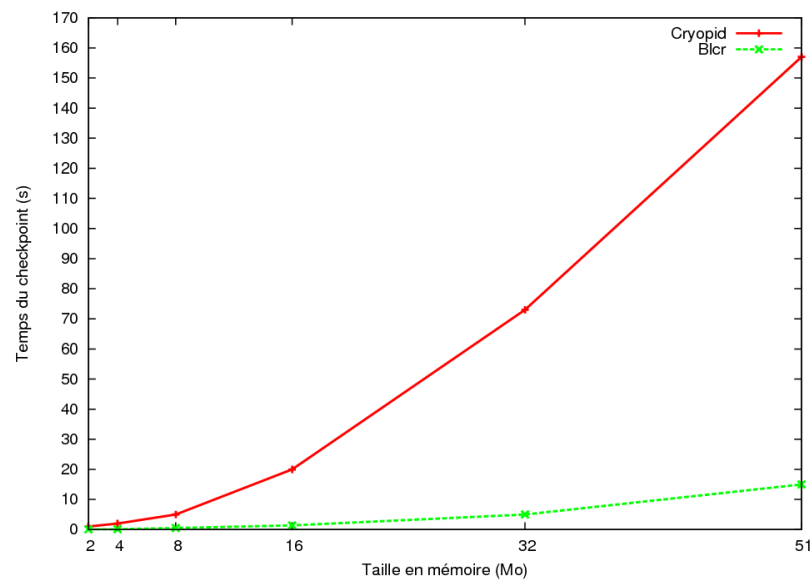
FIGURE 3.4 – Temps de sauvegarde réalisé avec BLCR et Cryopid sur le code Mandelbrot
