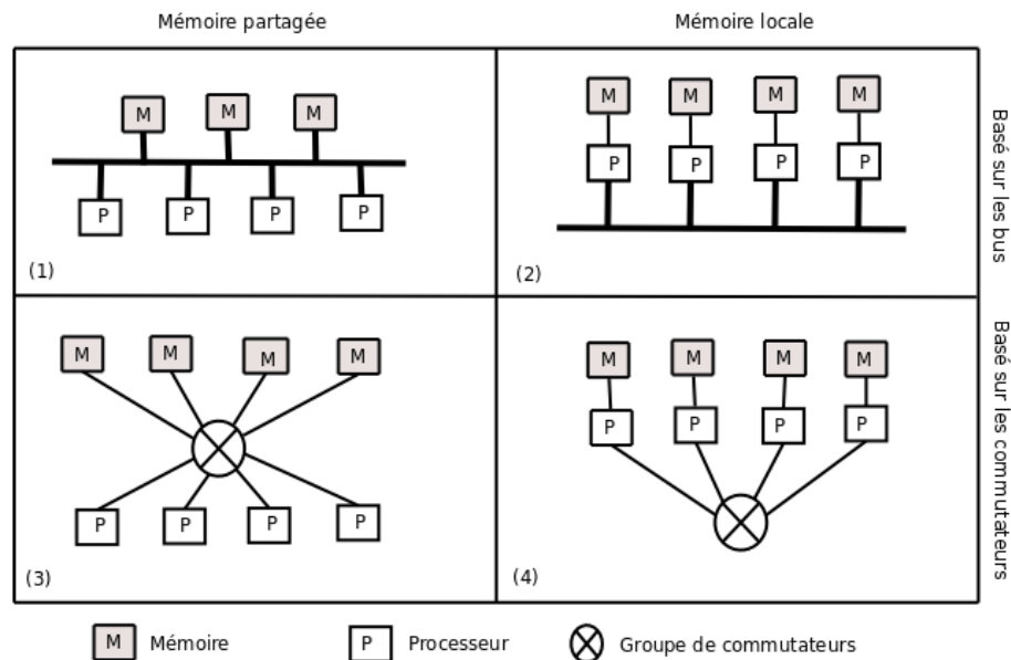
FIGURE 2.1 – Classification de Tanenbaum des architectures de machines de type MIMD
