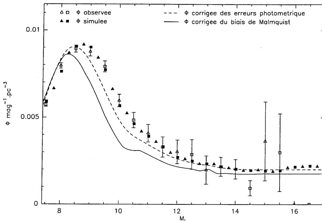
FIG. 2.37 – Fonction de luminosité corrigée des biais. La courbe en traits pointillés est la fonction de luminosité introduite dans le modèle simulant les erreurs photométriques. La fonction de luminosité en carré et triangle pleins est celle produite par le modèle après ajout des erreurs photométriques, elle est choisie pour ajuster la fonction de luminosité observée (triangle et carré vides). Enfin, la fonction de luminosité en trait plein est obtenue après la correction du biais de Malmquist. Les carrés et triangles symbolisent deux systèmes d'intervalles (de une magnitude) entrelacés.
