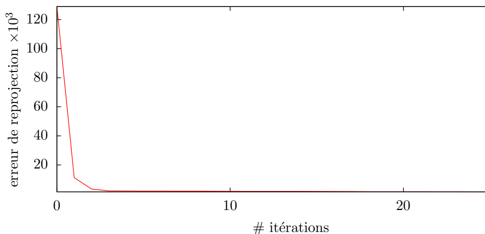
FIG. 3.7 – Étalonage du système d'acquisition : évolution de l'erreur de re-projection.
