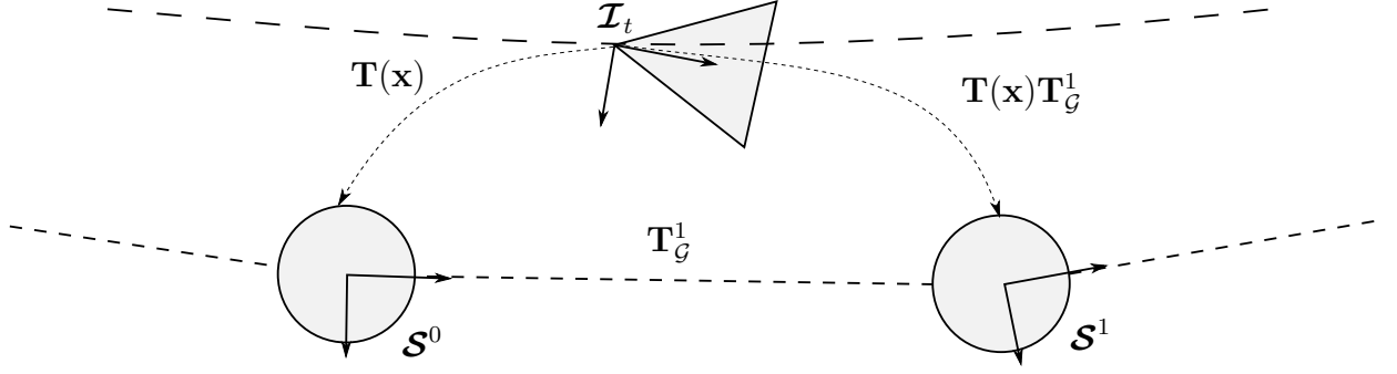
FIG. 6.2 – Schéma d'utilisation simultanée de plusieurs nœuds du graphe. La localisation de l'image I_t est effectuée avec les nœuds S^0 et S^1 .
