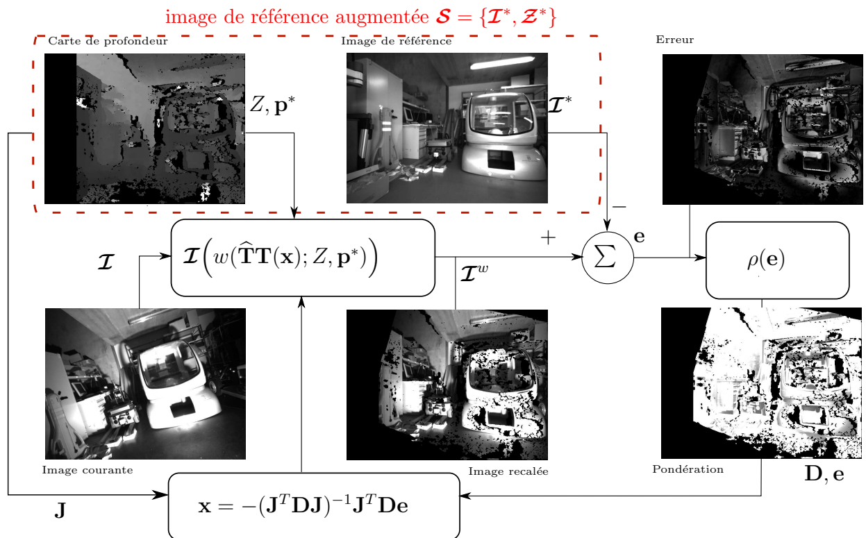
FIG. 2.4 – Processus de minimisation directe robuste : Les intensités de l'image \mathcal{I} , sont itérativement recalées sur l'image \mathcal{I}^* . L'image de pondération \mathbf{D} , calculée en fonction de l'erreur \mathbf{e} permet mettre à jour le déplacement 3D \mathbf{x} de manière robuste.
