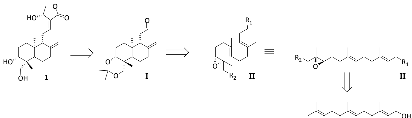
Figure 54 : Analyse rétrosynthétique
