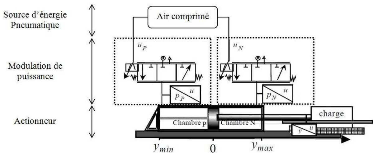
Figure V-2 : Système électropneumatique
