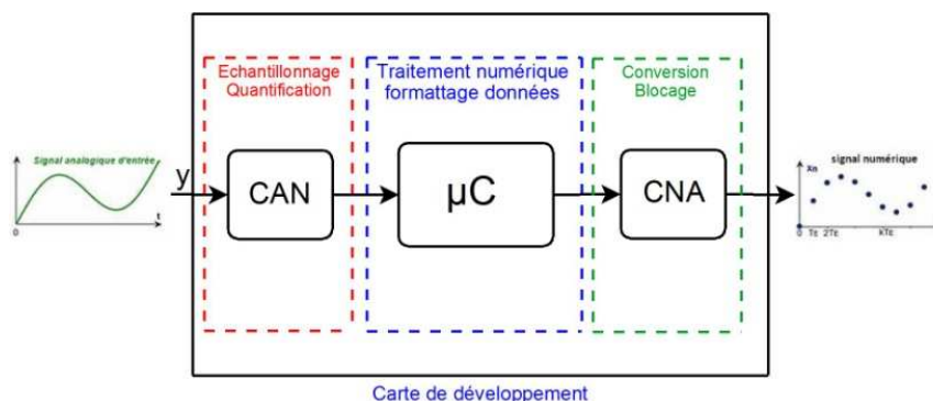
Figure IV-2: Chaîne d'acquisition
