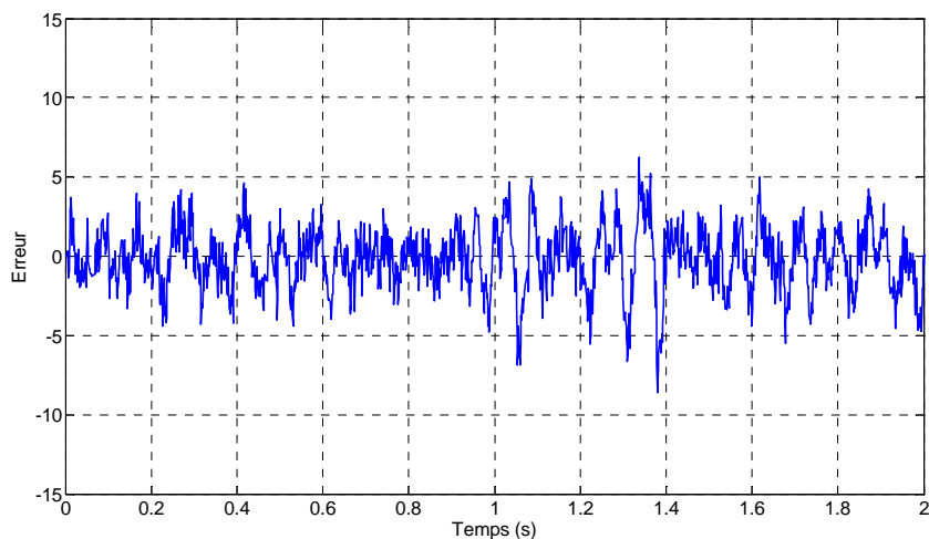
Figure IV-11 : Observateur Grand Gain : erreur de dérivation
