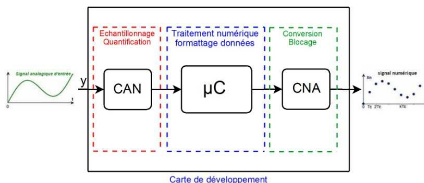
Figure IV-2: Chaîne d'acquisition
