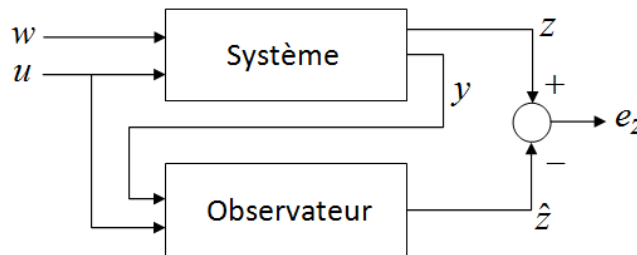
Figure I-6 : Observateur d'état
