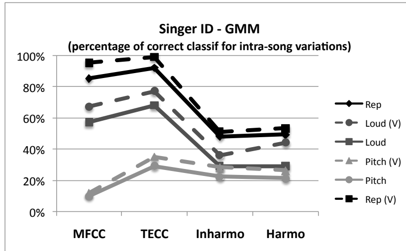
Figure 2.10: Classification Accuracy pour les variations de hauteur et d'intensité obtenus avec des GMM. Résultats obtenus après vote (V) sont tracés avec des lignes pointillées
