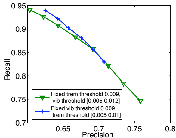
Figure 2.5: Exemples de courbe PR obtenues en variant un seuil
