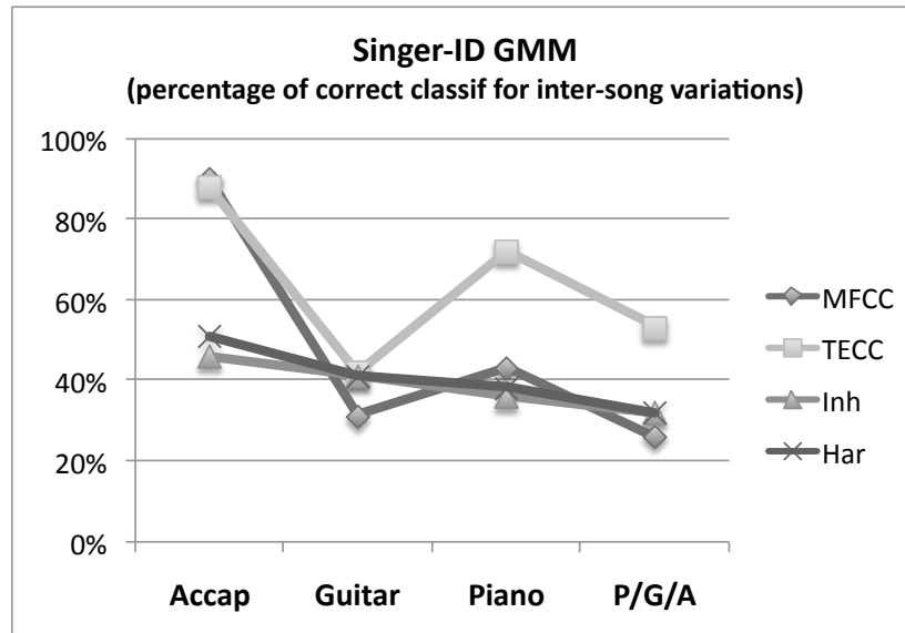
Figure 2.11: Classification Accuracy obtenus pour différents accompagnements instrumentaux avant vote
