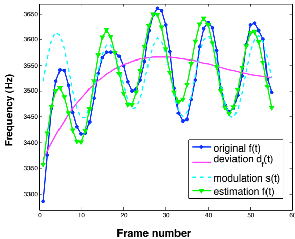
Figure 2.2: Estimation sur une note vibrée
