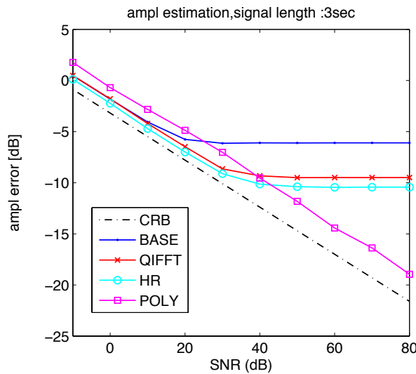
Figure 4.8: CRB : S1- amplitude - (3sec)
