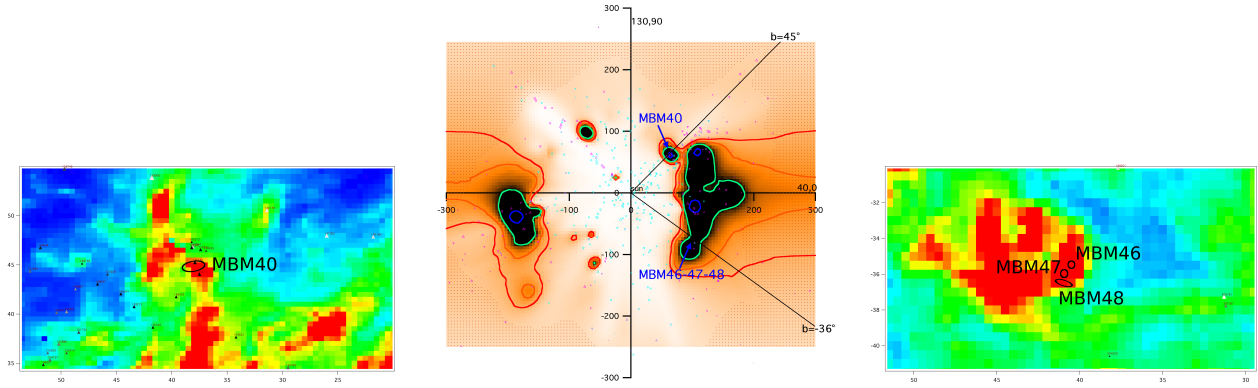
FIGURE 6.2 – Carte HI à 21cm à la vitesse LSR 3.5 \text{ km.s}^{-1} autour de la localisation du MBM40 (à gauche). Distribution du NaI résultant de l'inversion de la base de données interstellaires du sodium. Nous montrons une coupe dans le cube de densité 3D le long du plan vertical contenant le Soleil et orienté vers les longitudes galactiques 40 and 220^\circ (au milieu). Identique à la figure de gauche entre les vitesses LSR 0.5 et 1.5 \text{ km.s}^{-1} autour de la localisation des MBM46-47-48 (à droite).
