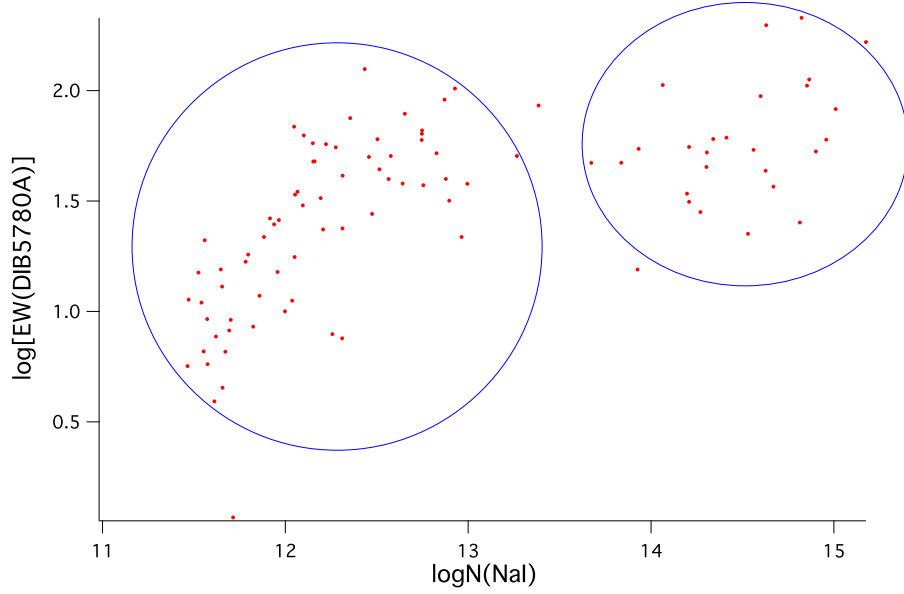
FIGURE 9.1 – \log[\text{EW}(\text{DIB}5780.5\text{\AA})] vs. \log[N(\text{NaI})] . On note la présence de deux nuages de points.
