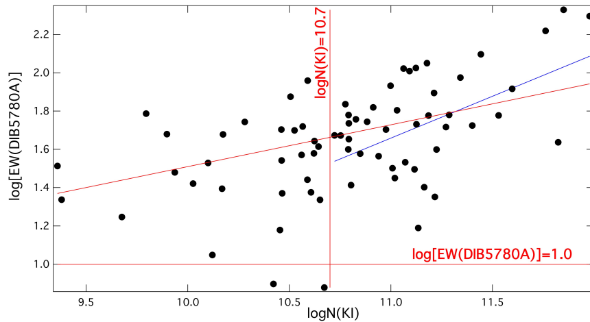
FIGURE 9.7 – \log[EW(DIB5780.5\text{\AA})] vs. \log[N(KI)] . Nous montrons la pente obtenue en utilisant tous les points et celle obtenue en excluant les valeurs inférieures au seuil de détection pour le potassium. On voit qu'il est difficile ici d'établir une relation fiable étant donné l'intervalle étroit dont nous disposons.
