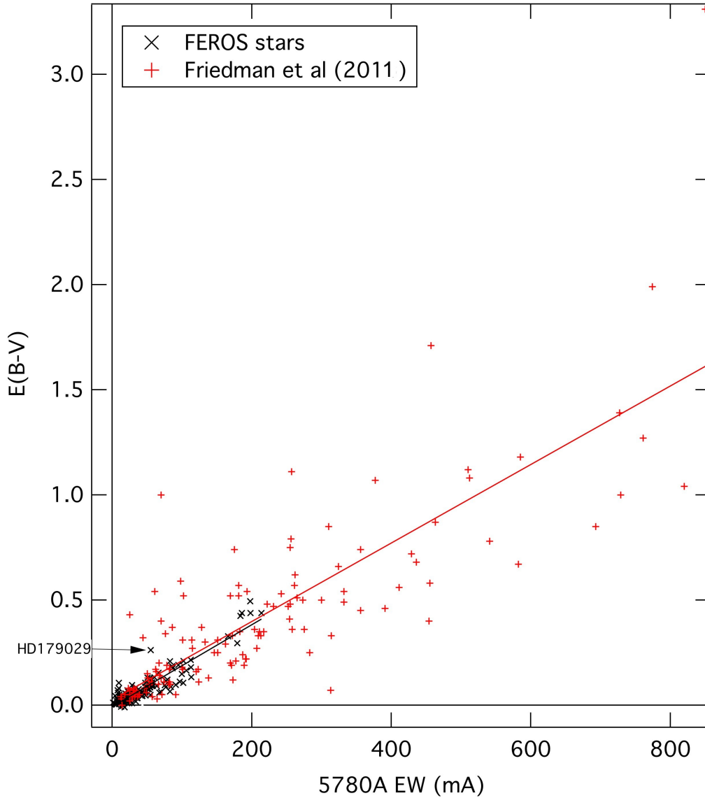
FIGURE 8.11 – Excès de couleur E(B - V) en fonction de la largeur équivalente de la DIB à 5780.5Å. Aux 135 lignes de visée extraites des observations Feros (en noir) sont ajoutées les 133 valeurs de Friedman et al. (2011) (en rouge). On voit que leurs données couvrent un intervalle de rougissemments nettement plus élevé. On voit également que globalement leurs points sont plus dispersés que pour les spectres Feros .
