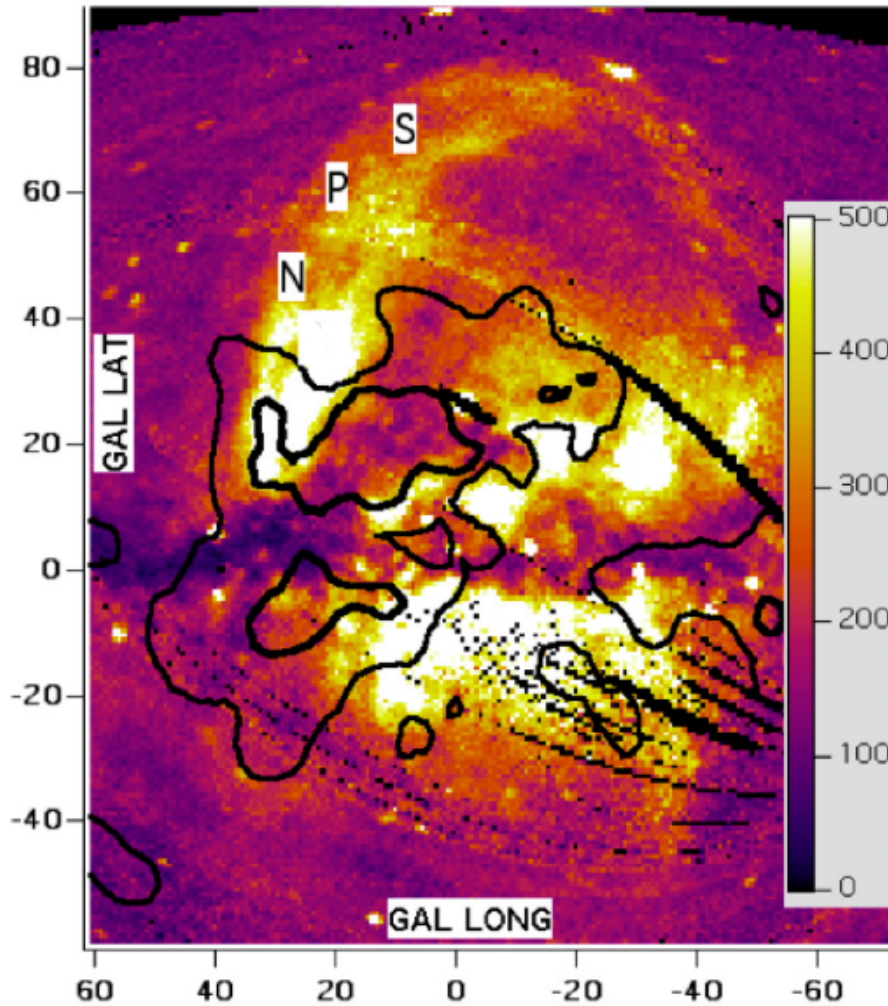
FIGURE 5.20 – Carte ROSAT de l'émission X à 3/4 de keV représentant la NPS/Loop I dans sa globalité.
