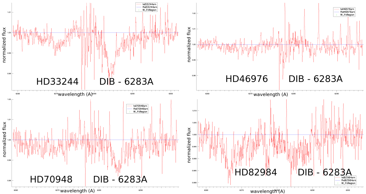
FIGURE 8.7 – DIB à 6283.8\text{\AA} . La DIB est très bruitée et très mal décontaminée.
