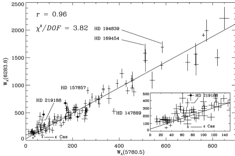
FIGURE 8.17 – EW(DIB6283.8\text{\AA}) vs. EW(DIB5780.5\text{\AA}) mesurés par Friedman et al. (2011).
