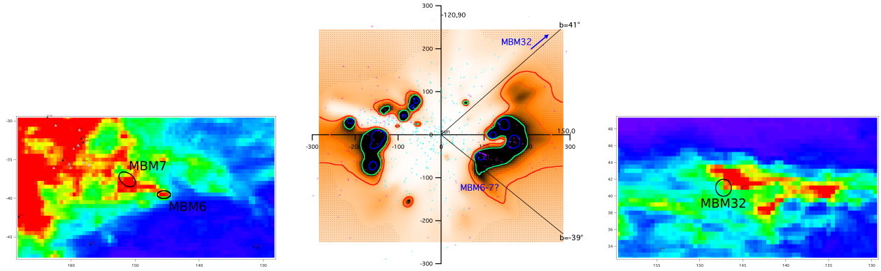
FIGURE 6.8 – Carte HI à 21cm entre les vitesses LSR 4.5 et 6.8 \text{km.s}^{-1} autour de la localisation des MBM6 et MBM7 (à gauche). Distribution du NaI résultant de l'inversion de la base de données interstellaires du sodium. Nous montrons une coupe dans le cube de densité 3D le long du plan vertical contenant le Soleil et orienté vers les longitudes galactiques 150 and 330° (au milieu). Identique à la figure de gauche à la vitesses LSR 4.0 \text{km.s}^{-1} autour de la localisation du MBM32 (à droite).
