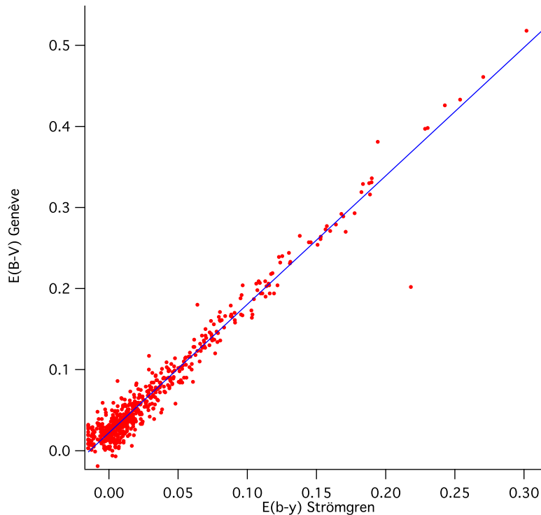
FIGURE 10.1 – Excès de couleur E(B-V)_G dans le système photométrique de Genève en fonction de l'excès de couleur E(b-y)_S en photométrie Strömgen.
