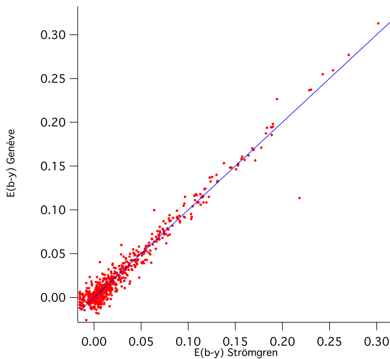
FIGURE 10.2 – E(b - y)_G vs. E(b - y)_S . On représente le E(b - y)_G de la photométrie de Genève en fonction du E(b - y)_S obtenu par Strömgren.
