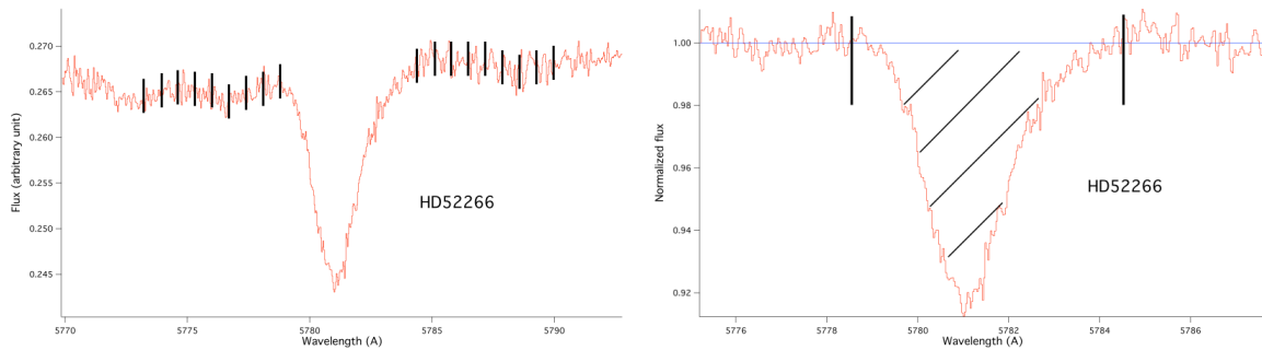
FIGURE 8.5 – Exemple d’ajustement de la DIB à 5780.5 Å pour l’étoile HD52266 : définition du continu stellaire (à gauche) puis détermination de l’intervalle d’ajustement sur le spectre normalisé (à droite). La partie hachurée correspond à la surface permettant le calcul de la largeur équivalente de la DIB.
