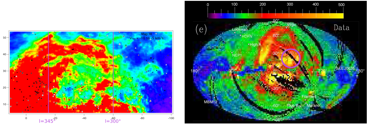
FIGURE 5.25 – Bulle dans la région de Lupus visible dans différentes longueurs d'onde. A gauche, bulle visible en HI dans l'intervalle de vitesse héliocentrique de -10 à -5 \text{km.s}^{-1} . A droite, bulle visible dans la carte X de ROSAT à 3/4 de keV (entourée en violet).
