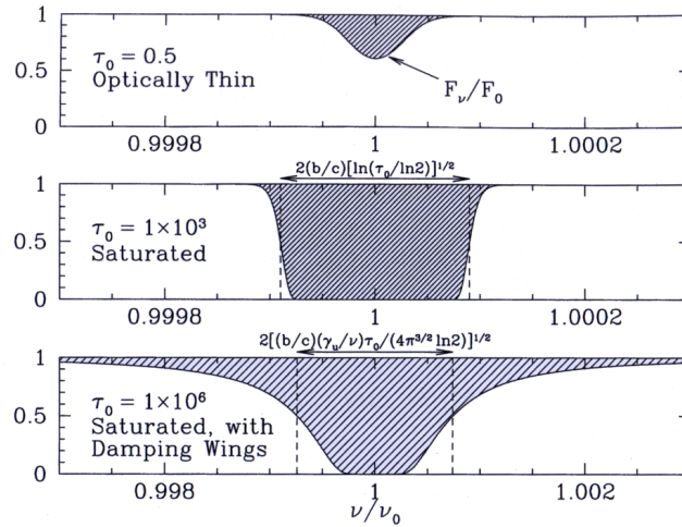
FIGURE 4.3 – Profils d’absorption dans trois régimes, en utilisant comme exemple l’hydrogène Lyman \alpha avec b = 10 \text{ km.s}^{-1} et N(\text{H I}) = 6.6 \times 10^{12} \text{ cm}^{-2} , 1.3 \times 10^{16} \text{ cm}^{-2} , et 1.3 \times 10^{19} \text{ cm}^{-2} respectivement dans les figures du haut, du milieu et du bas. Les régions hachurées correspondent à l’absorption sur la ligne de visée. (Draine 2011)
