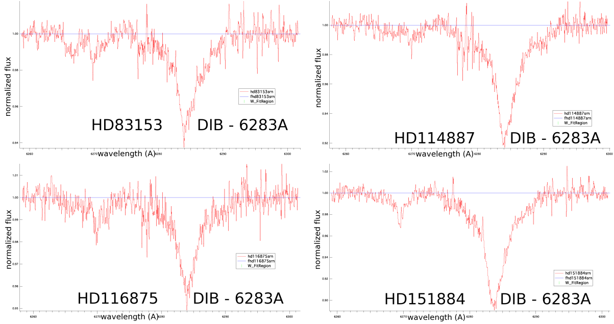
FIGURE 8.6 – DIB à 6283.8\text{\AA} . La DIB est facilement identifiable.
