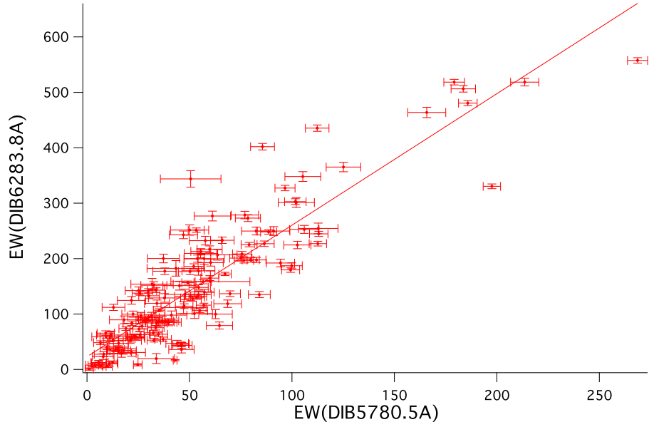
FIGURE 8.16 – EW(DIB6283.8\text{\AA}) vs. EW(DIB5780.5\text{\AA}) mesurés dans cette étude.
