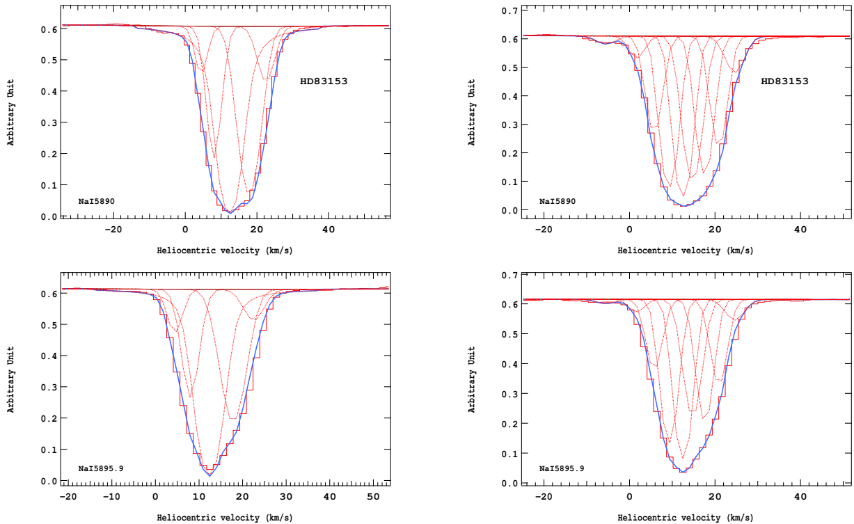
FIGURE 7.8 – A gauche, ancien ajustement du continu de l'étoile HD83153 avec 5 composantes; la densité de colonne est de 1.02335 \cdot 10^{15} \text{cm}^{-2} (en haut la raie D2, en bas la raie D1). A droite, nouvel ajustement du continu de l'étoile HD83153 avec 9 composantes; la densité de colonne est de 1.4962 \cdot 10^{13} \text{cm}^{-2} , soit beaucoup moins importante que lors du précédent ajustement (en haut la raie D2, en bas la raie D1).
