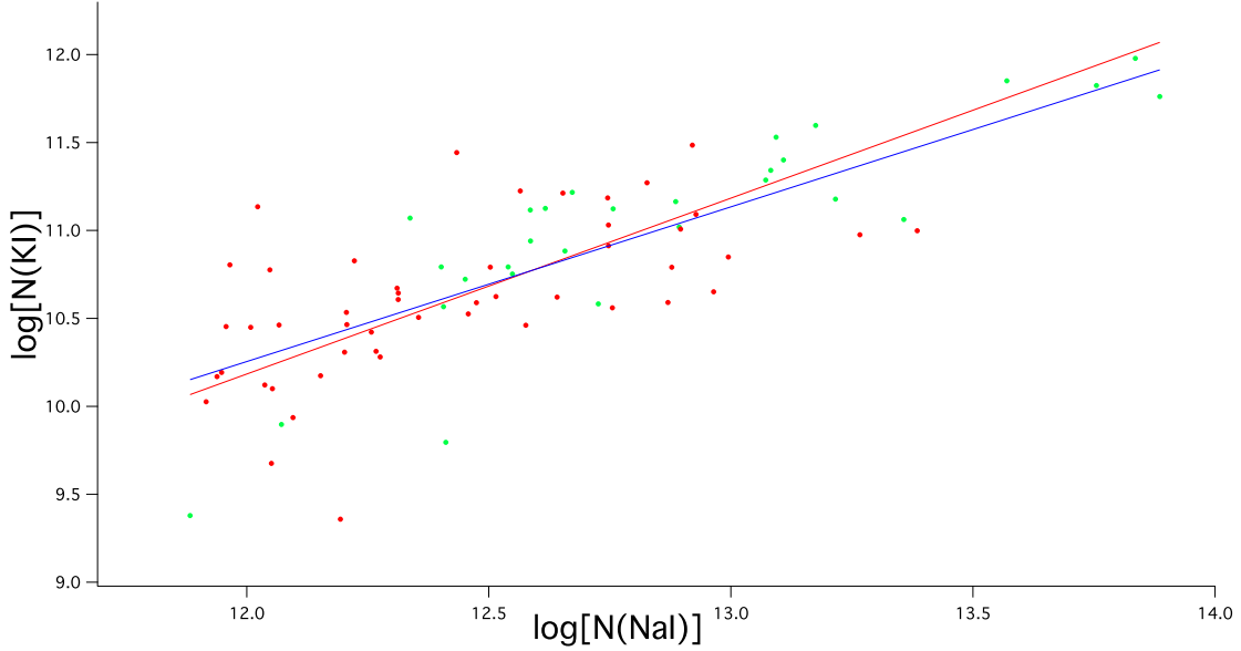
FIGURE 7.12 – \log[N(KI)] en fonction de \log[N(NaI)] . Le graphique montre l’ajustement avec les données Feros en trait bleu (l’ajustement en trait rouge correspond à une pente de 1). Les points rouges correspondent aux étoiles du premier nuage de points pour lesquels la densité de colonne n’a pas été recalculée tandis que les points verts correspondent aux étoiles du deuxième nuage de points pour lesquels la densité de colonne a été mesurée par une nouvelle méthode d’ajustement.
