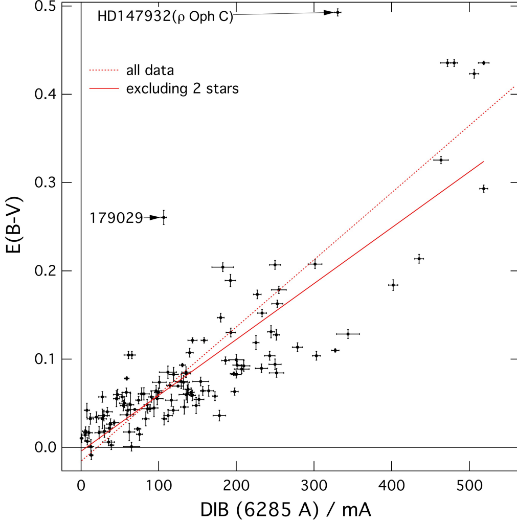
FIGURE 8.13 – E(B - V) vs. EW(DIB6283.8\text{\AA}) pour les 123 mesures Feros .
