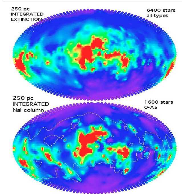
FIGURE 5.12 – Extinction intégrée (en haut) et NaI intégré (en bas) le long des lignes de visée provenant des cubes d'inversion jusqu'à 250pc, représentés en coordonnées Aitoff. Un isocontour d'opacité (la ligne blanche) correspondant à un E(B - V) de 0.028 est dessiné sur la carte en sodium pour une comparaison plus facile.
