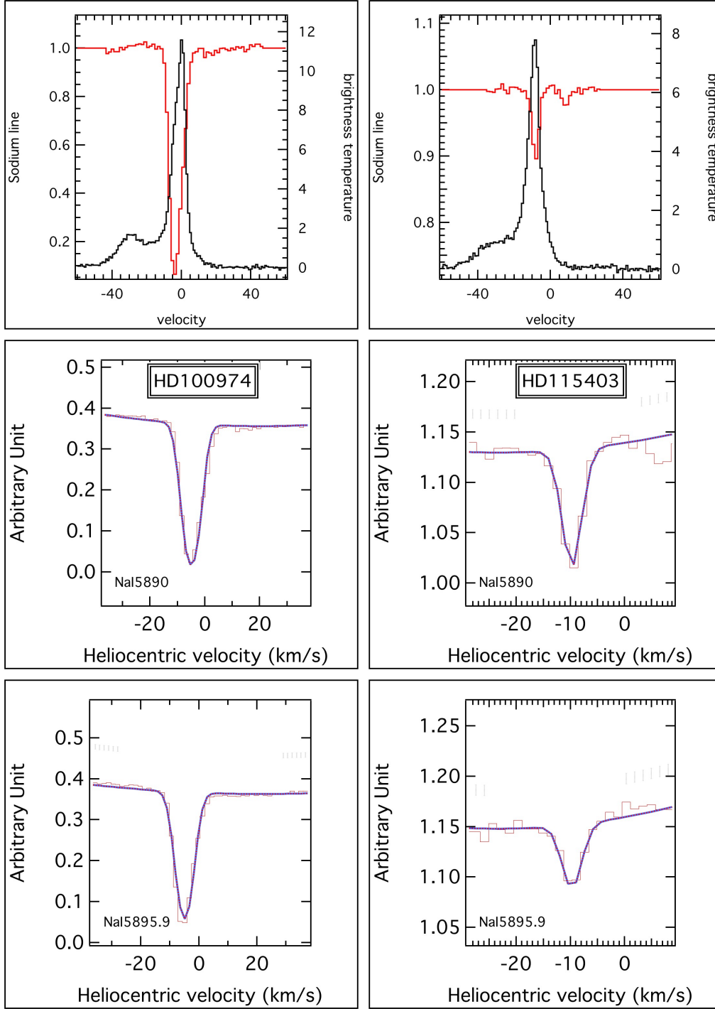
FIGURE 5.23 – Spectre des étoiles HD100974 (à gauche) et HD115403 (à droite) au niveau du doublet du NaI. Les figures du haut montre l'absorption de la raie D2 superposée à l'émission H \alpha sur la même ligne de visée, montrant une même vitesse du gaz H \alpha et NaI. Les figures du milieu présentent l'ajustement de la raie D2 du doublet tandis que les figures du bas montrent l'ajustement de la raie D1 du doublet du sodium neutre.
