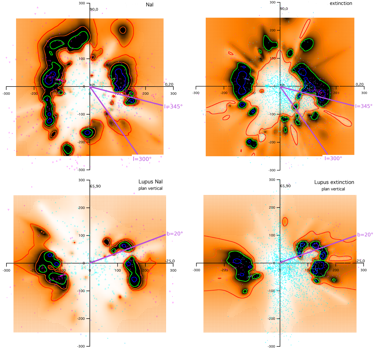
FIGURE 5.24 – Présence de la bulle dans les coupes en NaI et en extinction. En haut, coupes dans les cubes en NaI (à gauche) et en extinction (à droite) passant par ( l=0^\circ, b=20^\circ ) et ( l=90^\circ, b=0^\circ ). En bas, coupes verticales dans les cubes en NaI (à gauche) et en extinction (à droite) à la longitude l=335^\circ .
