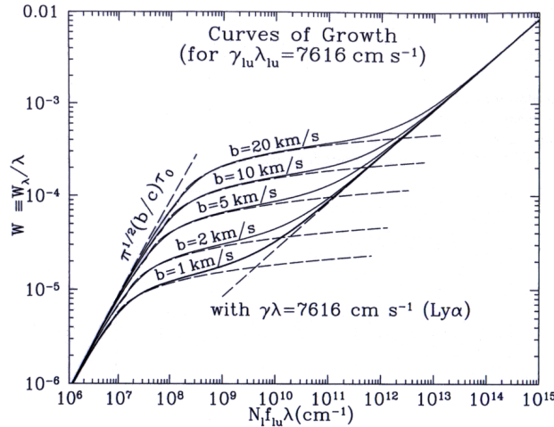
FIGURE 4.4 – Courbes de croissance pour cinq valeurs du paramètre d'élargissement Doppler b , pour une constante \gamma_{lu} \lambda_{lu} = 7616 \text{ cm.s}^{-1} (cette constante est ici appropriée à l'hydrogène Lyman \alpha ). Les lignes pointillées montrent les approximations analytiques aux portions linéaire (régime optiquement mince), plate (régime de saturation) et en racine carré (régime de saturation avec des ailes d'amortissement) des courbes de croissance. (Draine 2011)
