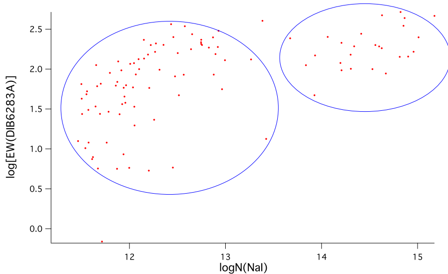
FIGURE 9.2 – \log[\text{EW}(\text{DIB}6283.8\text{\AA})] vs. \log[N(\text{NaI})] . On note la présence de deux nuages de points.
