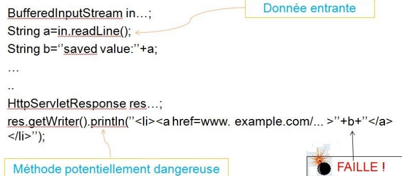
FIGURE 5.3 – Exemple de faille d'injection dans une jsp.
