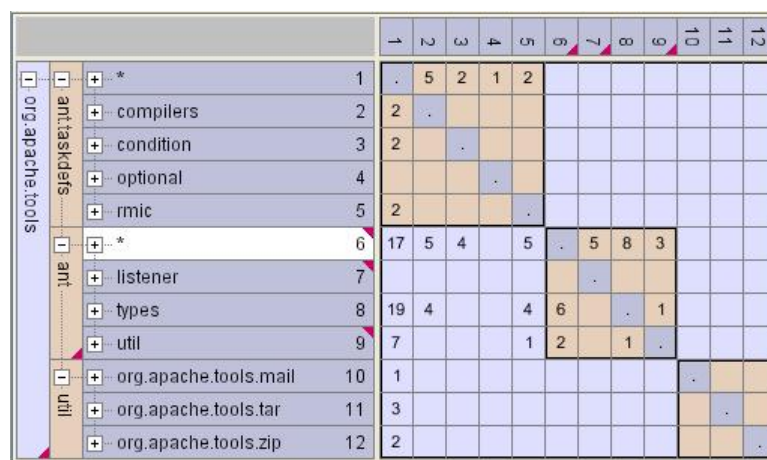
FIGURE C.1 – Représentation matricielle des dépendances
