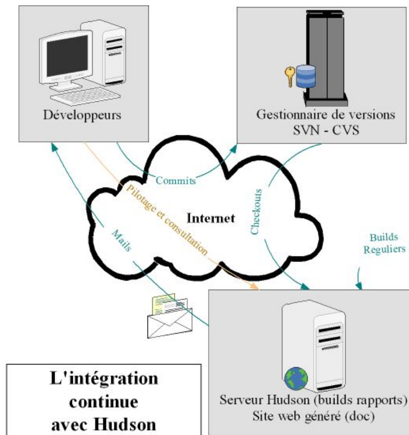
FIGURE A.2 – Intégration continue
