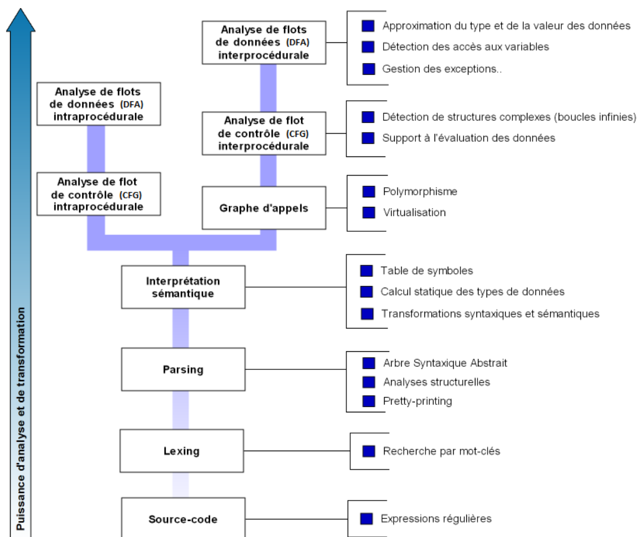
FIGURE 4.8 – Hiérarchie des analyses d'un code.
