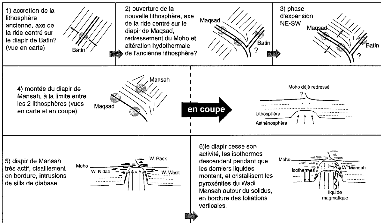
Figure 5.11: scénario possible pour la formation de la région de Mansah (situation des diapirs de Batin, Maqsad et Mansah tirés de la figure 1 de la note du chapitre II (Boudier et al, 1997)).
