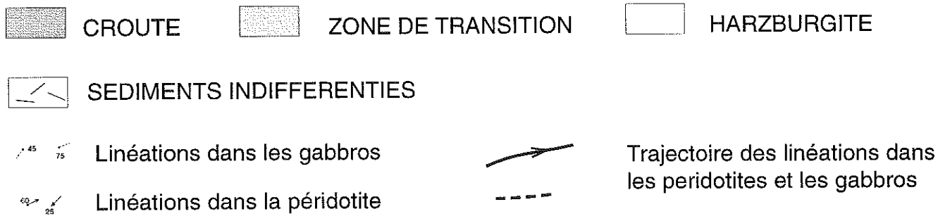
Figure 5.3b: carte des trajectoires des linéations de la région de Mansah
