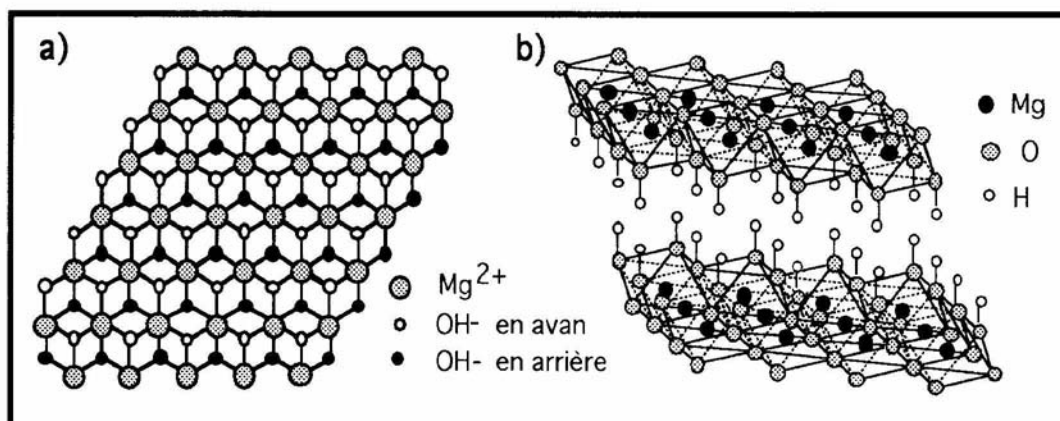
Figure 3. Représentation schématique de Mg(OH)_2 (a) dans le plan (a,b) et (b) selon l'axe c.
