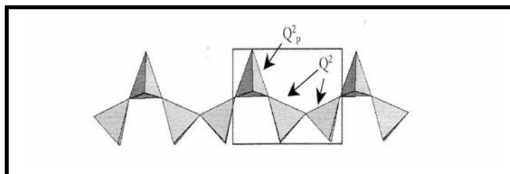
Figure 16. Modèle de chaîne de tétraèdres de silicium dans les C-H-S. Motif "dreierketten" est représenté dans le cadre.
