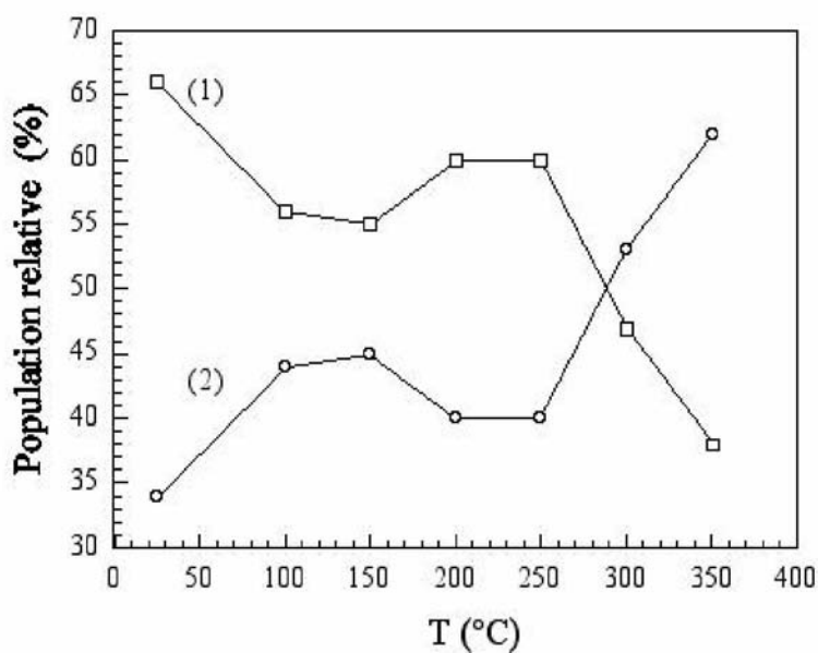
Figure 33. Population relative des sites Fe(1) et Fe(2) en fonction de la température.
