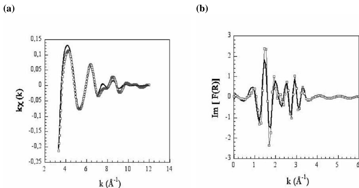
Figure 31. Simulation EXAFS au seuil K du Fe du composé [\text{Ca}_2\text{-Fe-CrO}_4^{2-}] ; (a) à 175^\circ\text{C} et (b) la partie imaginaire, avec ( \square ) expérimentale et (—) théorique.
