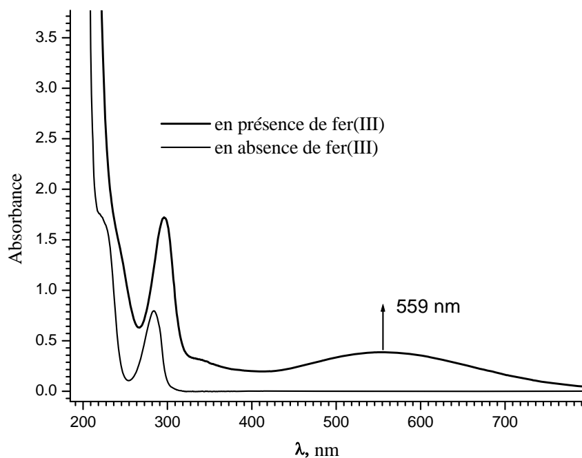
Figure IV.31-b) : Spectres d'absorption UV-visible d'une solution de 4-chlorocatechol ( 3 \times 10^{-4} \text{ mol.L}^{-1} ) en absence et en présence de fer(III) ( 3 \times 10^{-4} \text{ mol.L}^{-1} ).
