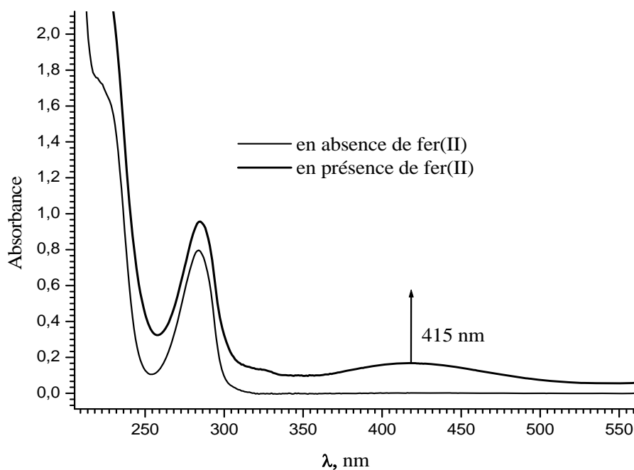
Figure IV.31-a) : Spectres d'absorption UV-visible d'une solution de 4-chlorocatechol ( 3 \times 10^{-4} \text{ mol.L}^{-1} ) en absence et en présence de fer(II) ( 3 \times 10^{-4} \text{ mol.L}^{-1} )
