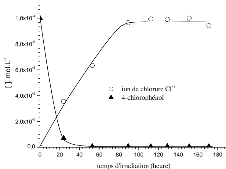
Figure V.27 : Disparition du 4-CP et formation des ions chlorures \text{Cl}^- lors de l'irradiation à 365 nm d'un mélange [\text{FeCitrate}] = 3 \times 10^{-4} \text{ mol.L}^{-1} et [4\text{-CP}] = 1 \times 10^{-4} \text{ mol.L}^{-1} , pH = 3,0, solution aérée
