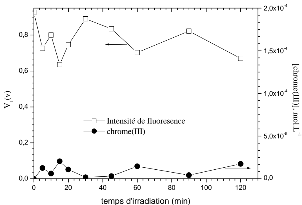
Figure VI.7 : Cinétique de formation du chrome(III) au cours de l'irradiation du chrome(VI) et du complexe FeNTA à pH neutre. [FeNTA] = 3 \times 10^{-4} \text{ mol.L}^{-1} ; [chrome(VI)] = 2 \times 10^{-4} \text{ mol.L}^{-1} ; \lambda_{excitation} = 313 \text{ nm} ; milieu aéré, pH = 7,0 .
