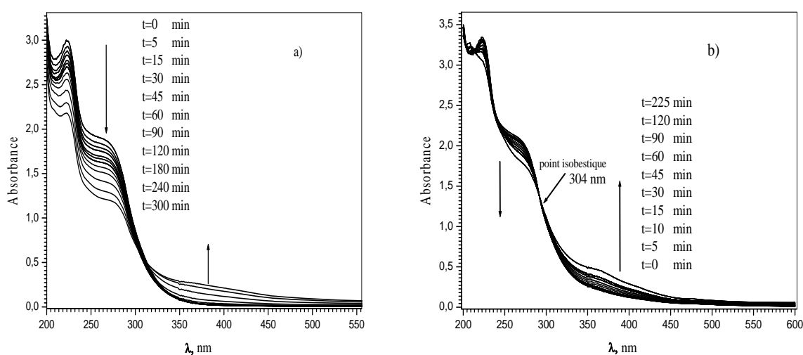
Figure IV.14 : Evolution du spectre d'absorption UV-visible d'un mélange de FeNTA/4-CP ( 3 \times 10^{-4} \text{ mol.L}^{-1} / 10^{-4} \text{ mol.L}^{-1} ) en fonction du temps d'irradiation ; a) pH = 4,0 ; b) pH = 6,0 ; \lambda = 365 \text{ nm} (monochromateur).
