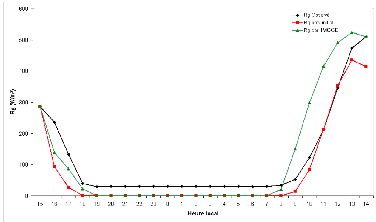
Figure 48. Évolution et comparaison sur 24 heures du rayonnement solaire global observé, prévu initialement par le modèle et prévu après correction par les données de l'IMCCE. Station de Sal Bas journée du 14-02-2003.
