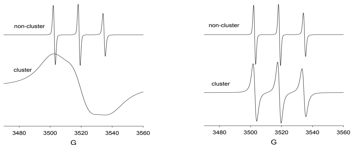
Figure 2-14. Spectres RPE obtenus pour les formes agrégées (en bas) et non-agrégées (en haut) des composés LLF-3-CP (à gauche) et LLH-3-CP (à droite)
