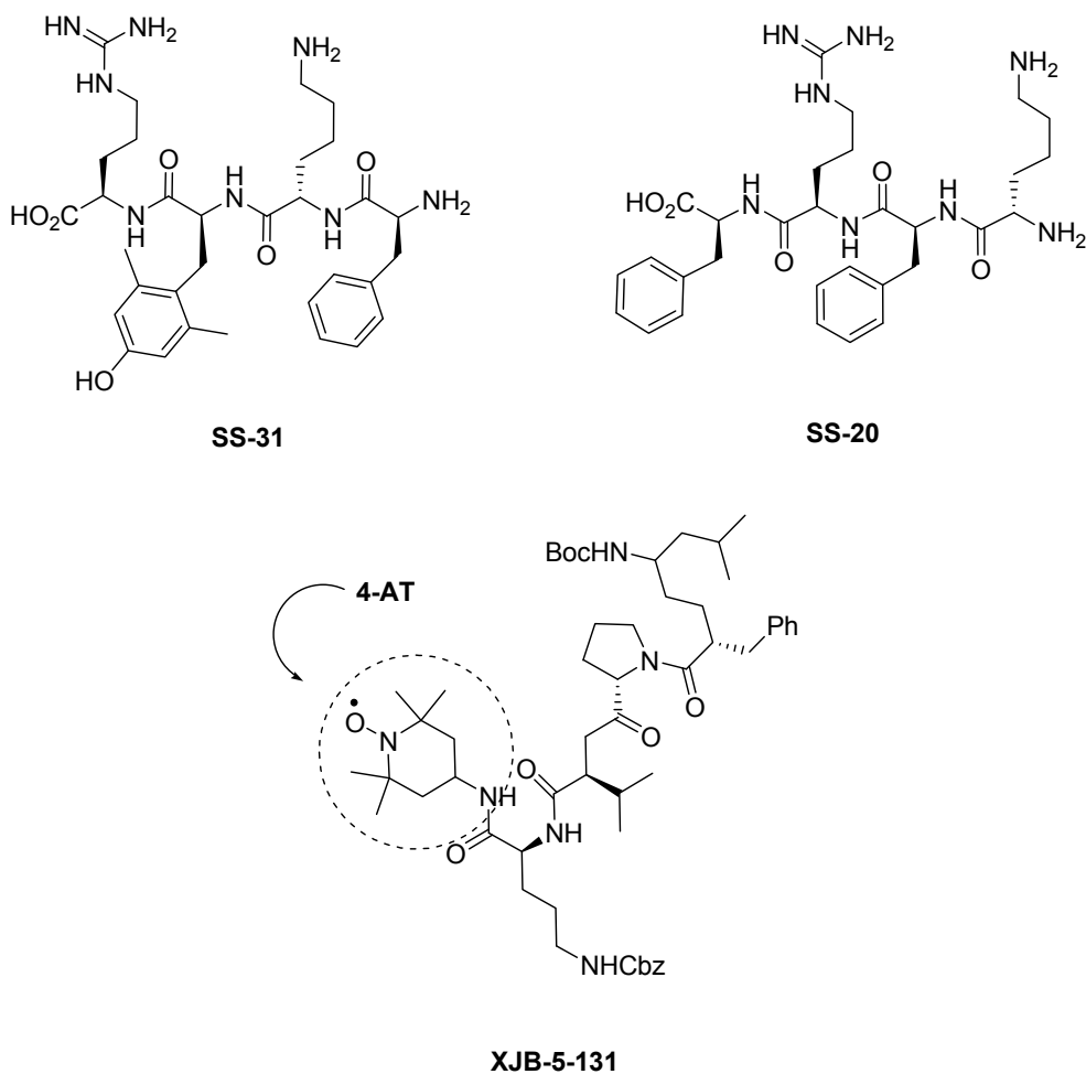
Figure 1-14. Structures des SS-31 et SS-20, ainsi que de la XJB-5-131
