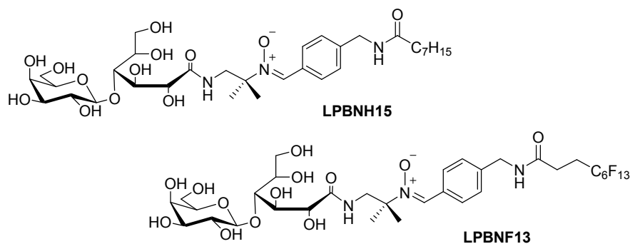
Figure 3-3. Structures chimiques de la LPBNH15 et de la LPBNF13
