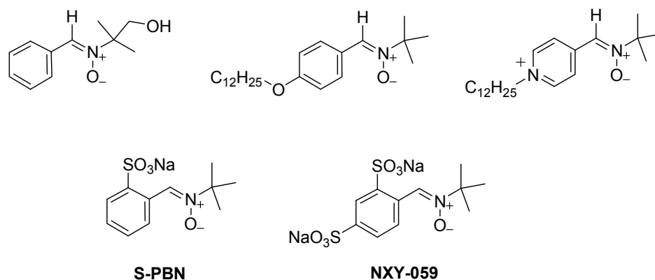
Figure 1-18. Exemples d’analogues de la PBN modifiés soit sur la partie N-terminale, soit sur la partie aromatique
