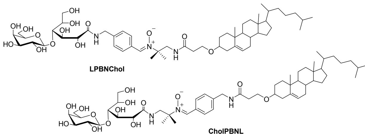
Figure 3-5. Structures chimiques de la LPBNChol et de la CholPBNL
