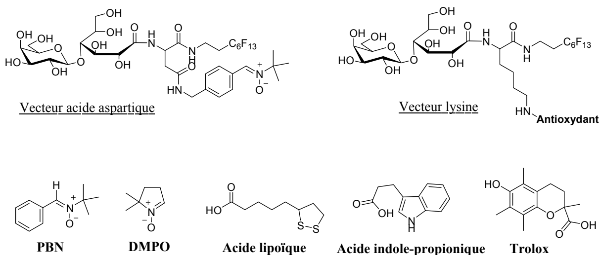
Figure 2-2. Structures chimiques des dérivés amphiphiles transporteurs d'antioxydants.
