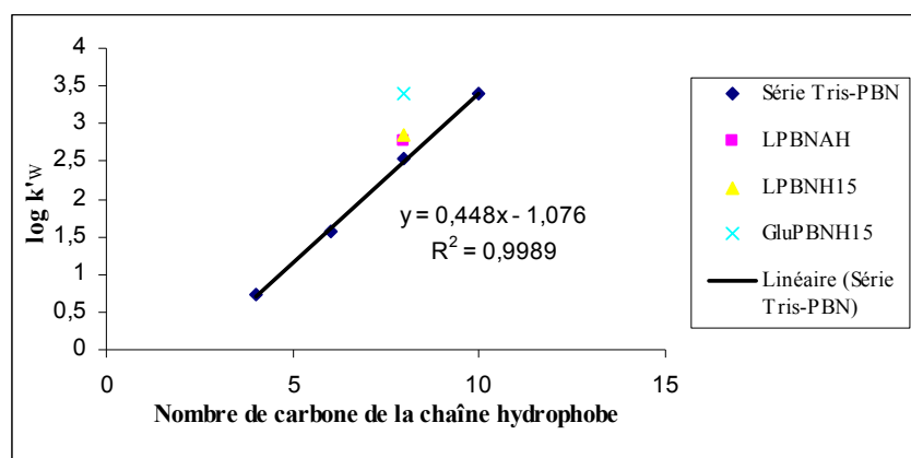
Figure 3-14. Variation de l'hydrophobie des nitrones amphiphiles en fonction de leurs longueurs de chaîne hydrophobe ou de la nature de leurs têtes polaires
