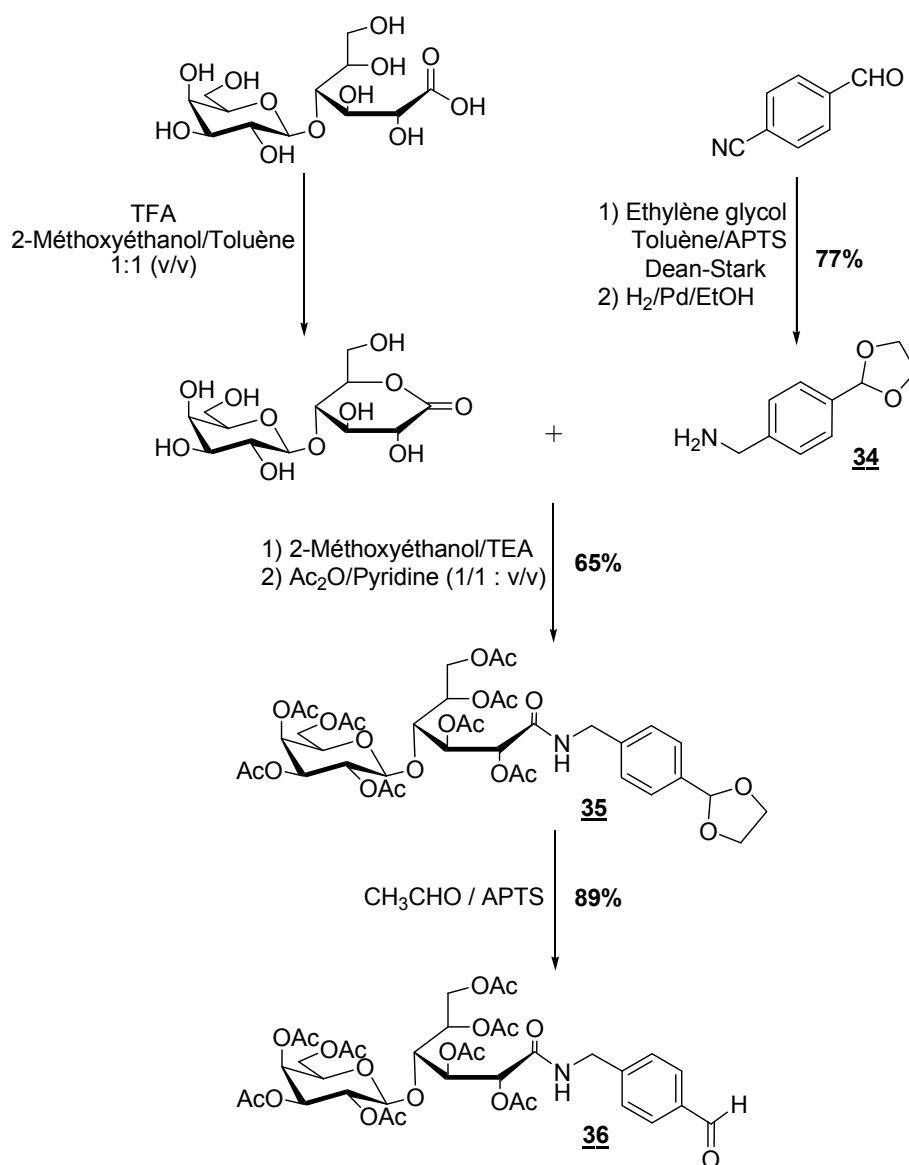
Schéma 3-5. Synthèse de l'aldéhyde à motif lactobionolactone dérivé du 4-cyanobenzaldéhyde
