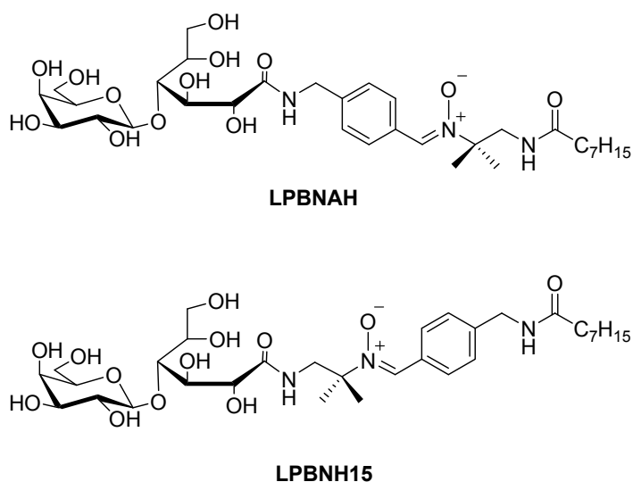
Figure 1-22. Structures chimiques de la LPBNAH et de la LPBNH15
