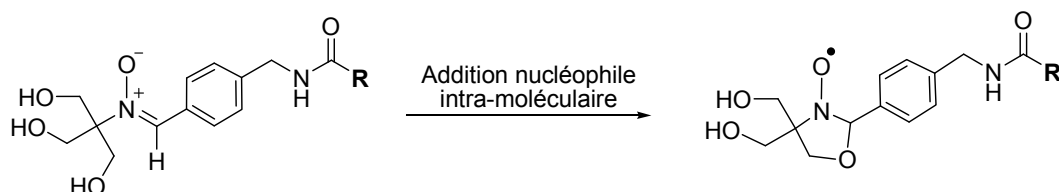
Schéma 3-16. Formation du nitroxyde de type A par addition nucléophile intra-moléculaire
