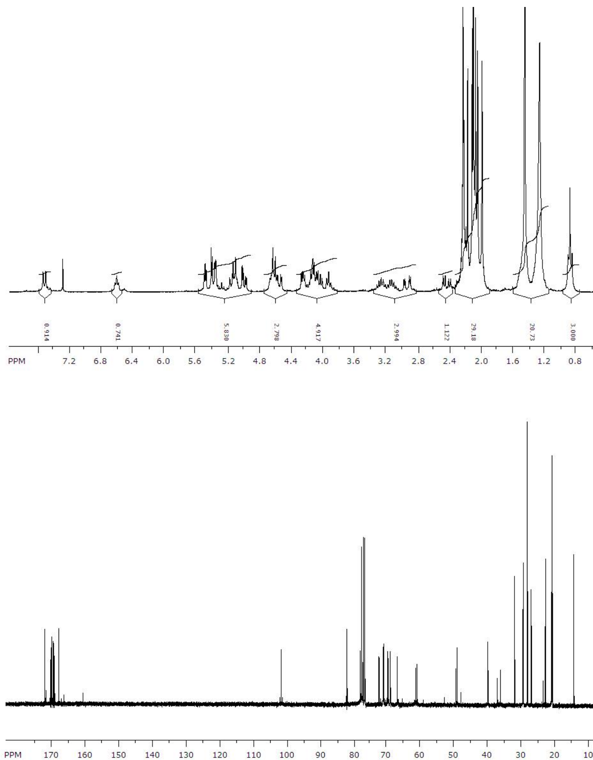
Figure 2-6. Spectre RMN du ^1\text{H} (en haut) et du ^{13}\text{C} (en bas) du composé 5
