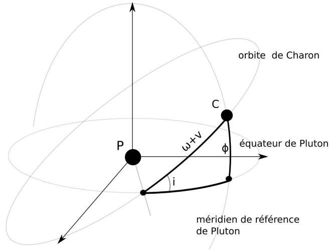
Figure 3.9 – Triangle sphérique liant l'inclinaison, la position sur l'orbite et la hauteur de Charon sur l'équateur de Pluton
