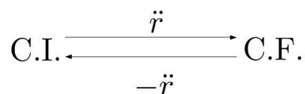
Figure 3.1 – Principe de l'aller-retour : à partir de conditions initiales données, on fait évoluer le système en intégrant les équation du mouvement, puis on le fait évoluer en sens inverse, à partir des conditions finales, jusqu'à retrouver les conditions initiales.
