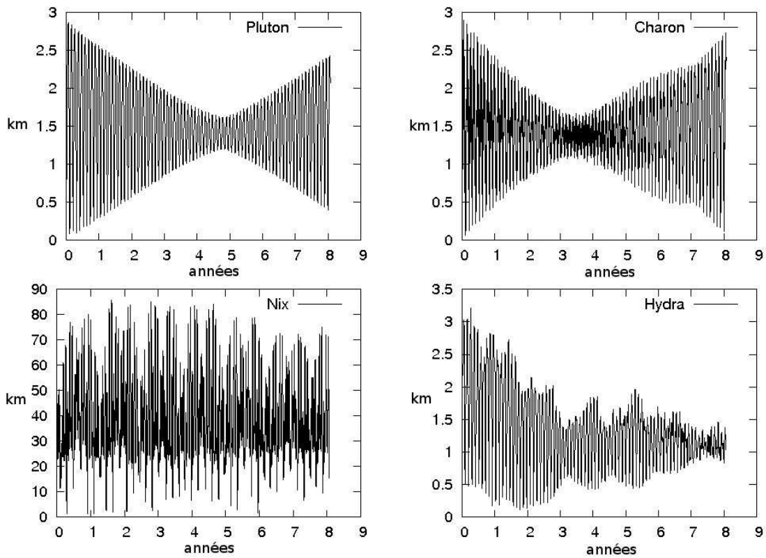
Figure 5.3 – Résidus de l’ajustement d’un modèle où la masse d’Hydra est nulle sur des observations simulées où GM_4 = 0.021 \pm 0.042 \text{km}^3 \text{s}^{-2} . Seules les positions et vitesses initiales des quatre corps ont été ajustées.
