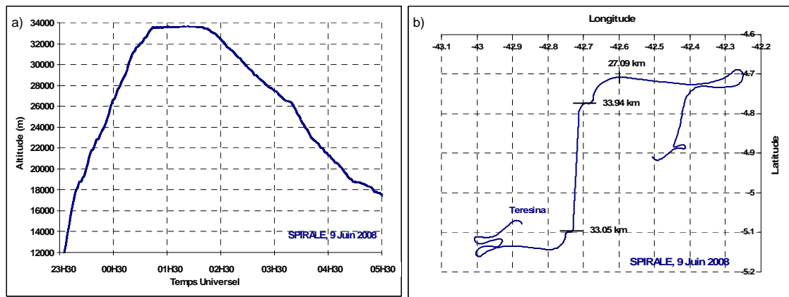
Figure 3-11 – Profil de vol de SPIRALE le 9-10 Juin 2008 à Teresina (a) et trajectoire de la nacelle (b).
