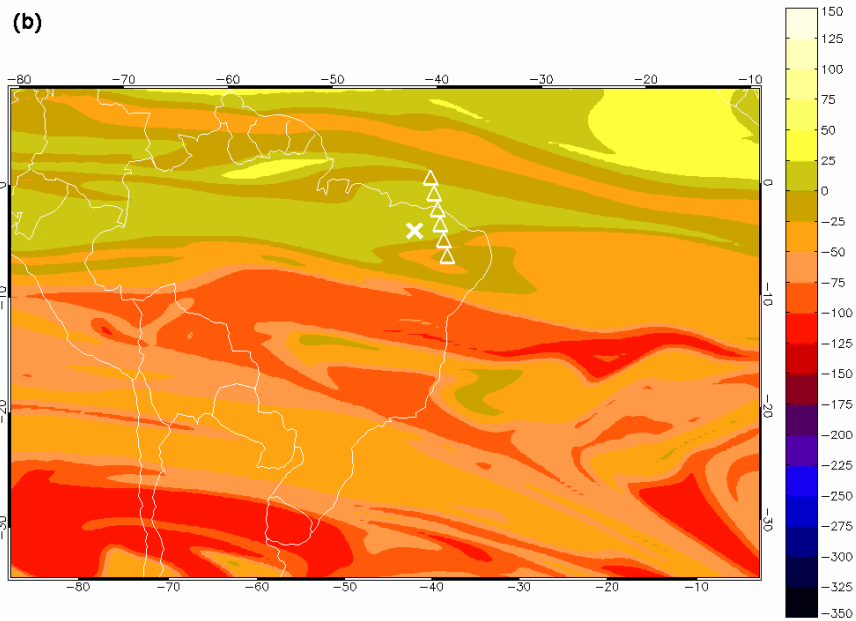
Figure 4-16 – Cartes de vorticité potentielle calculées par le modèle MIMOSA le 22 Juin 2005. La position de SPIRALE est indiquée par une croix, la position de MLS est indiquée par des triangles.
