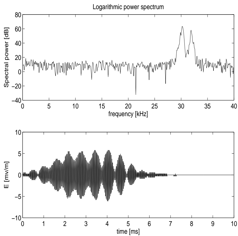
FIG. 22 – Exemple d’une forme d’onde capturée par WBD, où la totalité du paquet d’onde est contenue dans un bloc de données de WBD. La modulation lente est clairement visible.
