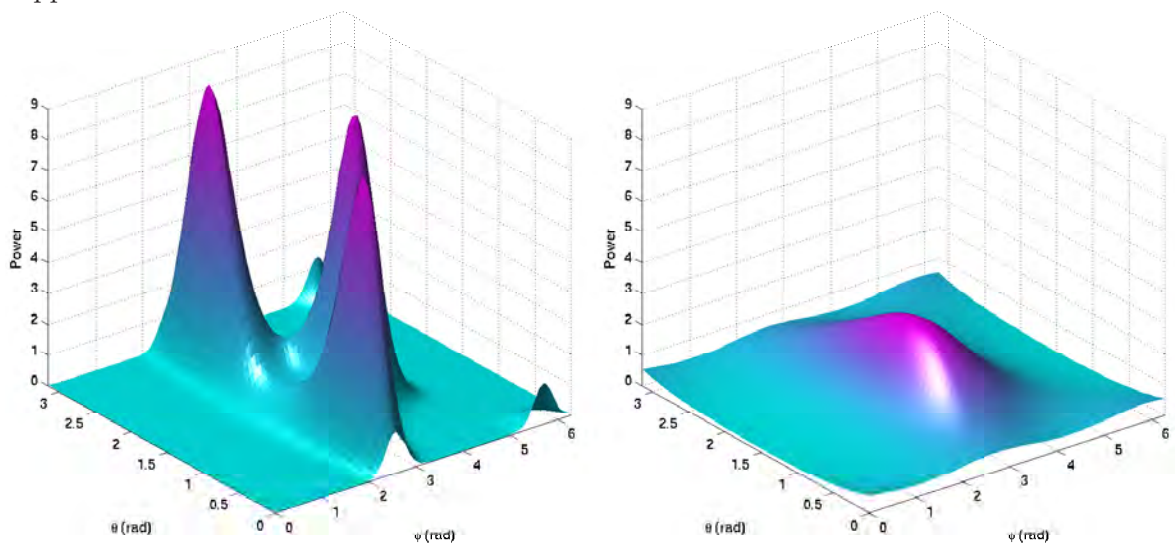
FIG. 5.3 – Calcul de la FDO dans le cas où V a été simulé à l’aide de trois masses de Dirac. A gauche : solution calculée pour \mu = 0.5 . A droite : solution calculée avec \mu = 50 .
