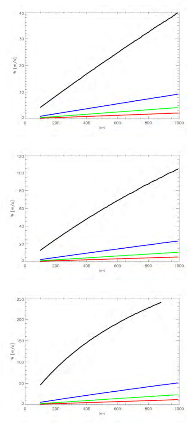
FIG. 3.26 – Elargissements moyens pour 23 extraits en fonction de la distance parcourue pour 9 MHz (en noir), 12 MHz (en bleu), 14 MHz (en vert) et 16MHz (en rouge), pour des fréquences plasma de 5 MHz (en haut), 6 MHz (au milieu) et 7 MHz(en bas).
