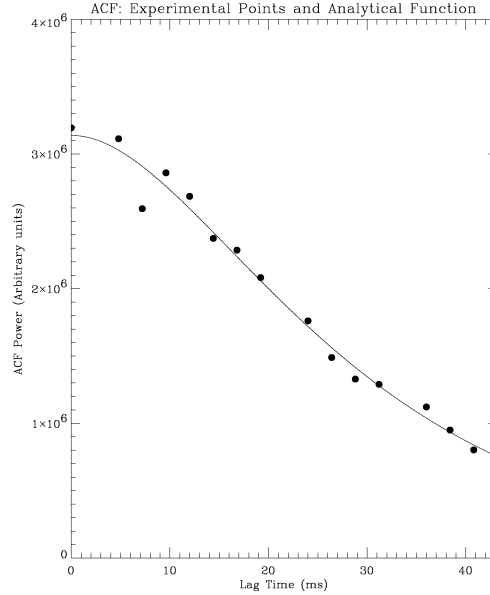
FIG. 2.1 – Exemple d’ajustement d’une fonction d’autocorrélation, d’après André (1997).
