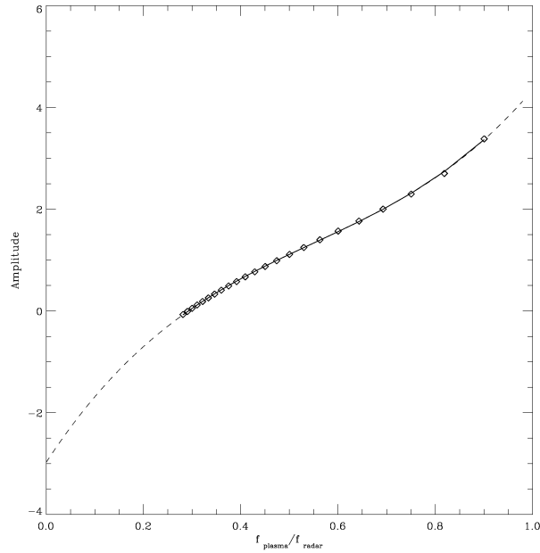
FIG. 3.20 – Exemple de dépendance de l'amplitude du spectre au rapport fréquence plasma sur fréquence radar. Les points expérimentaux sont représentés par les losanges, l'ajustement par un polynôme d'ordre 3 est en trait pointillé. L'échelle verticale est logarithmique.
