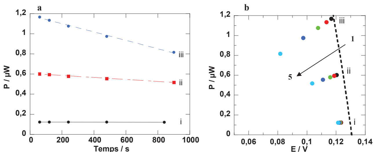
Figure III-10: a- Variation de la puissance de la pile décrite dans la Figure III-8 en fonction du temps de polarisation pour différents courants imposés : i- 1 \mu A , ii- 5 \mu A et iii- 10 \mu A . b- Évolution de la puissance de la pile en fonction du courant imposé et de la durée de la polarisation entre les électrodes : i- 1 \mu A , ii- 5 \mu A et iii- 10 \mu A . De 1 à 5 : 60 s, 120 s, 240 s, 480 s et 900 s. En pointillé, la courbe de puissance de la Figure III-8 pour v_b = 2 \text{ mV.s}^{-1}
