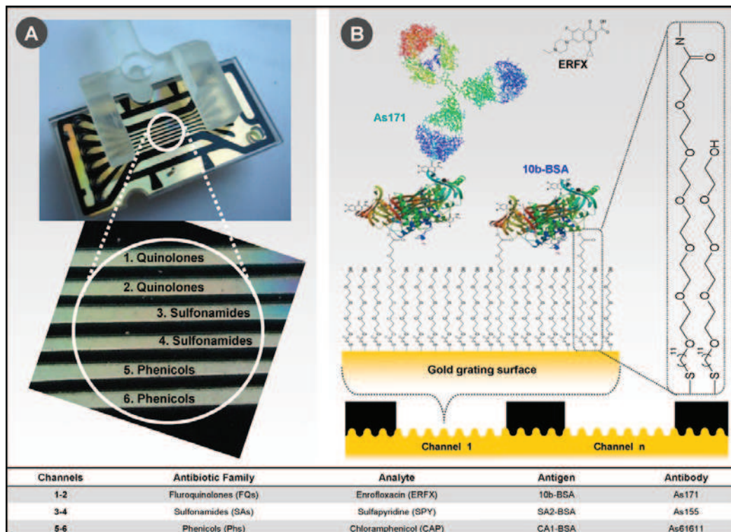
Figure I-4: Photographie de l'immunocapteur multivoies utilisant la SPR pour l'analyse simultanée d'anticorps dirigés contre l'enrofloxacin, la sulfapyridine et le chloramphenicol présents dans le lait. Reproduit de [26]
