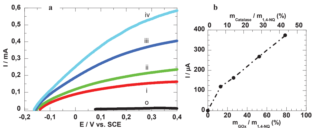
Figure IV-27: a- Courbes de polarisation de bioanodes compressées (Ø = 5 mm) de type GC/14NQ (ratio massique 75 : 25) et immergées dans une solution de NaCl 0,15 mol.L -1 , HEPES 25.10 -3 mol.L -1 , glucose 5,5.10 -3 mol.L -1 pour différents rapports massiques GOx-Catalase/Médiateur : o- 0-0 %, i- 13-7 %, ii- 26-14 %, iii- 52-29 %, iv- 79-43 %, v b = 1 mV.s -1
