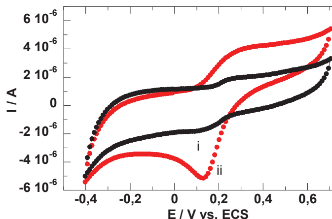
Figure IV-16: Courbes de voltampérométrie cyclique d'électrodes immergées dans une solution de NaCl 0,15 mol.L -1 , HEPES 25.10 -3 mol.L -1 , (pH = 7, 2, T_{\text{ambiante}} , air saturé) d'une micro-électrode à cavité de carbone graphite et remplie de i- Syringaldazine, ii- Ferrocène, v_b = 100\text{ mV.s}^{-1}
