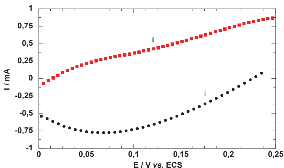
Figure III-3: Courbes courant-tension anodique et cathodique d'électrodes de feutre de carbone placées dans des membranes de dialyse de 100 Da contenant Q/QH_2 3,2 \cdot 10^{-3} \text{ mol.L}^{-1} et immergées dans une solution électrolytique de NaCl 0,15 \text{ mol.L}^{-1} , glucose 5,0 \cdot 10^{-3} \text{ mol.L}^{-1} et urée 3,5 \cdot 10^{-3} \text{ mol.L}^{-1} avec pH induits enzymatiquement : i- pH 3,15 (GOx/Catalase, 22,8/4 mg) ; ii- pH 7,62 (Uréease, 57,3 mg), v_b = 5 \text{ mV.s}^{-1}
