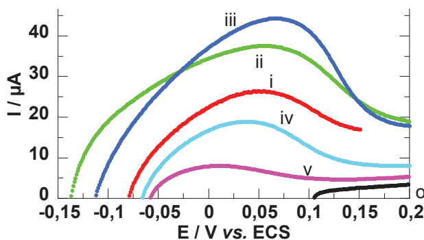
Figure IV-34: Courbes de polarisation de bioanodes compressées (Ø = 5 mm) de type GC/PQ immergées dans des solutions de NaCl 0,15 mol.L -1 , HEPES 25.10 -3 mol.L -1 , glucose 5,5.10 -3 mol.L -1 en faisant varier la proportion massique de PQ suivant le ratio GC/PQ : o- 100 :0, i-95 : 5, ii- 90 :10, iii- 75 :25, iv- 50 :50 et v- 33 :66 et des masses de GOx et de catalase de m GOx = 3,3 mg et m catalase = 1,6 mg ; v b = 1 mV.s -1
