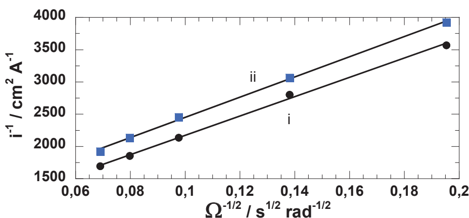
Figure II-4: Courbes de Koutecky-Levich obtenues à partir des courbes de courant-tension en régime stationnaire lors de la réduction de [\text{Ru}^{\text{III}}(\text{NH}_3)_6]^{3+} ( 2.10^{-3} \text{ mol}.\text{L}^{-1} ) dans du tampon phosphate ( 0,1 \text{ mol}.\text{L}^{-1} ; \text{pH} = 7,5 ) entre 0 et -0,65 V vs. ECS, v_b = 10 \text{ mV}.\text{s}^{-1} . i- électrode tournante de carbone vitreux ( \varnothing = 5 \text{ mm} ) modifiée par un film de ppyr-NHS, Q_{\text{polymérisation}} = 2,5 \text{ mC}.\text{cm}^{-2} ; ii- électrode modifiée puis incubée dans une solution du modèle de l'antibiotique ( 5 \text{ mg}.\text{mL}^{-1} + 2 \text{ eq. TEA} dans le DMF)
