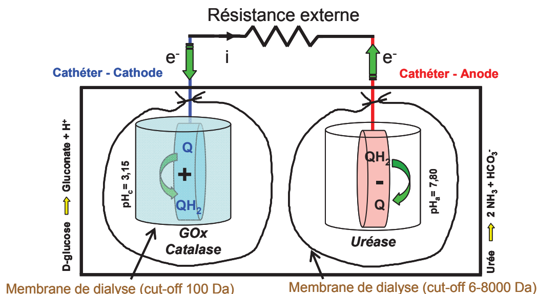
Schéma III-8 : Schéma de principe de la miniaturisation de la biopile à gradient de pH basée sur des électrodes de carbone compressées contenant la sonde rédox Q/QH_2 (77,6 mg) et immergées dans une solution électrolytique de NaCl 0,15 \text{ mol.L}^{-1} , glucose 5,0 \cdot 10^{-3} \text{ mol.L}^{-1} et urée 3,5 \cdot 10^{-3} \text{ mol.L}^{-1} et contenant GOx/Catalase (22,8 / 3,8 mg) côté anodique et Uréase (57,6 mg) côté cathodique
