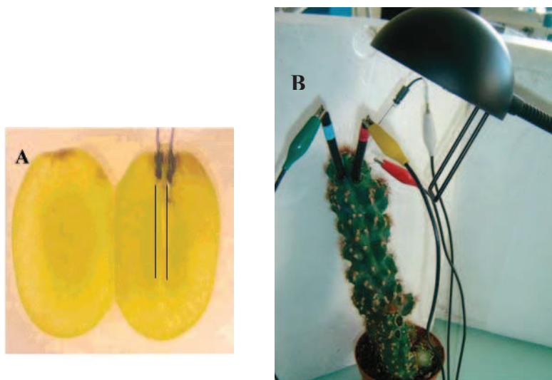
Figure I-16: Photographies de biopiles implantées dans des végétaux. A- Biopile à glucose/oxygène dans un raisin. Reproduit de [175]. B- Biopile à glucose/oxygène implantée dans un cactus. Reproduit de [174]. Pour les deux cas, les enzymes sont la GOx et la BOx immobilisées dans des hydrogels rédox à base d'osmium sur carbone
