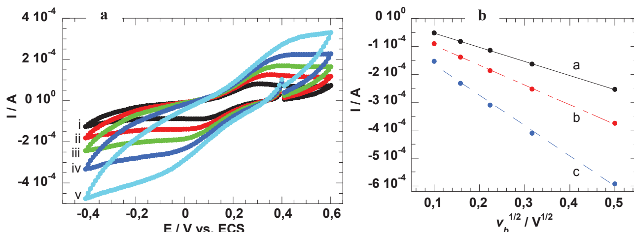
Figure IV-2: a- Courbes de voltampérométrie cyclique d'une électrode compactée ( \varnothing = 5 \text{ mm} ) immergée dans une solution de NaCl 0,15 \text{ mol.L}^{-1} , HEPES 25.10^{-3} \text{ mol.L}^{-1} ( \text{pH} = 7,2 , T_{\text{ambiante}} , air saturé) contenant [\text{Fe}^{\text{III}}(\text{CN})_6]^{3-} 2,5.10^{-3} \text{ mol.L}^{-1} pour différentes vitesses de balayage : i- 10 \text{ mV.s}^{-1} , ii- 25 \text{ mV.s}^{-1} , iii- 50 \text{ mV.s}^{-1} , iv- 100 \text{ mV.s}^{-1} , v- 250 \text{ mV.s}^{-1} . b- Dépendance du courant de pic cathodique par rapport à v_b^{1/2} de l'électrode précédente pour différentes concentrations de [\text{Fe}^{\text{III}}(\text{CN})_6]^{3-} : a- 1.10^{-3} \text{ mol.L}^{-1} , b- 2,5.10^{-3} \text{ mol.L}^{-1} , c- 5.10^{-3} \text{ mol.L}^{-1} . Équation de la régression linéaire de ii- 2,5.10^{-3} \text{ mol.L}^{-1} : y = - 2,426.10^{-5} - 7,089.10^{-4}x
