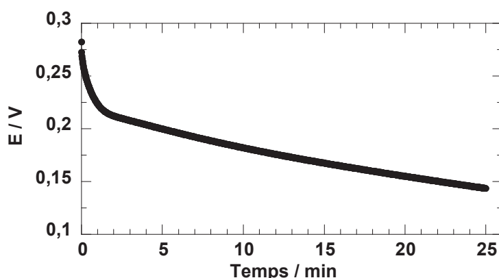
Figure IV-43: Courbe de décharge à courant constant ( I = 100 \mu A ) d'une pile à glucose oxygène TTF/PQ ( \varnothing = 13 \text{ mm} ) immergée dans une solution de NaCl 0,15 \text{ mol.L}^{-1} , HEPES 25.10^{-3} \text{ mol.L}^{-1} , glucose 5,5.10^{-3} \text{ mol.L}^{-1} ( pH = 7,2 , T_{\text{ambiante}} , air saturé)
