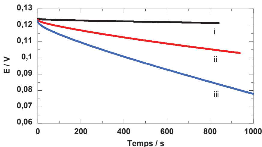
Figure III-9: Courbes de décharge de la pile à gradient de pH décrite dans la Figure III-8 soumise au passage d'un courant. i- 1 \mu A, ii- 5 \mu A, iii- 10 \mu A
