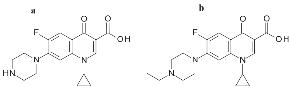
Schéma II-10 : Structure des deux antibiotiques utilisés. a- la ciprofloxacine (CF) et b- l'enrofloxacin (EF)
