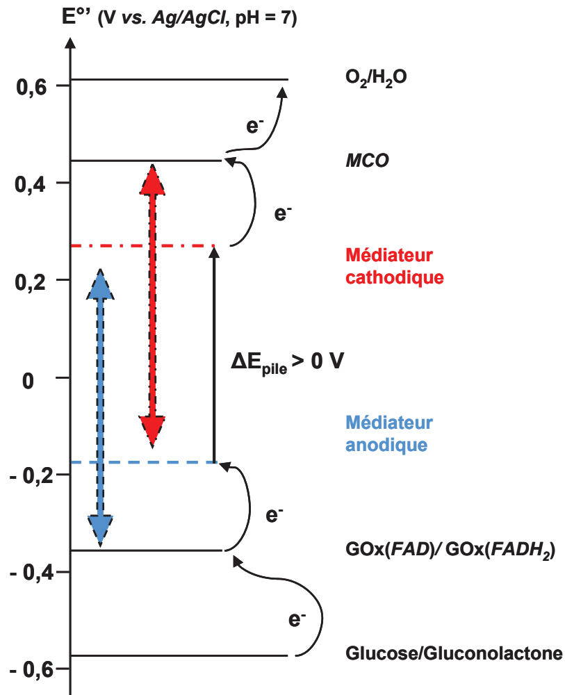
Schéma I-17: Échelles des potentiels standards des différents couples redox mis en contribution dans une pile à glucose/oxygène. Le potentiel représentant le potentiel de la MCO peut varier suivant le type d'enzyme utilisée ou suivant l'organisme d'où celle-ci est extraite. Les flèches indiquent les gammes de potentiel adéquates pour le choix des médiateurs anodiques et cathodiques (flèches bleue et rouge, respectivement)
