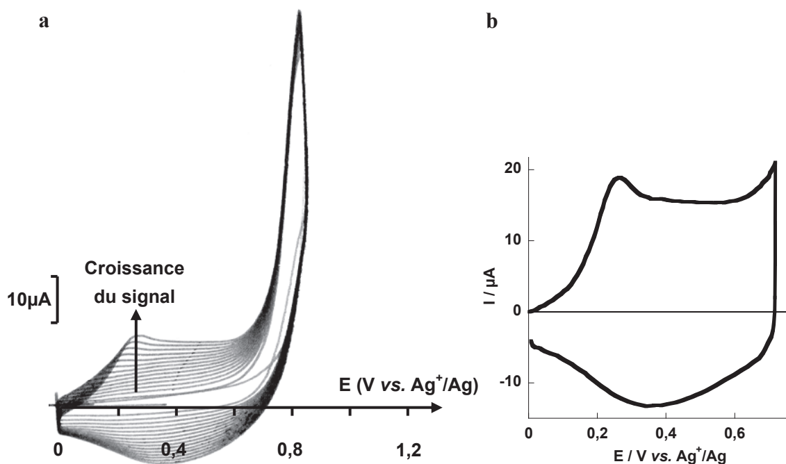
Figure II-2: a- Voltampérométrie cyclique du pyrrole-NHS ( 2.10^{-3} \text{ mol.L}^{-1} ) dans \text{CH}_3\text{CN} + 0,1 \text{ mol.L}^{-1} TBAP sur électrode de carbone vitreux ( \varnothing = 3 \text{ mm} ), v_b = 100 \text{ mV.s}^{-1} , n_{\text{cycle}} = 15 . b- Voltampérogramme d'une électrode de carbone vitreux ( \varnothing = 3 \text{ mm} ) modifiée par le poly(pyrrole-NHS) obtenue par voltampérométrie cyclique après 15 cycles et transférée dans \text{CH}_3\text{CN} + 0,1 \text{ mol.L}^{-1} TBAP exempt de monomère, v_b = 100 \text{ m V.s}^{-1}
