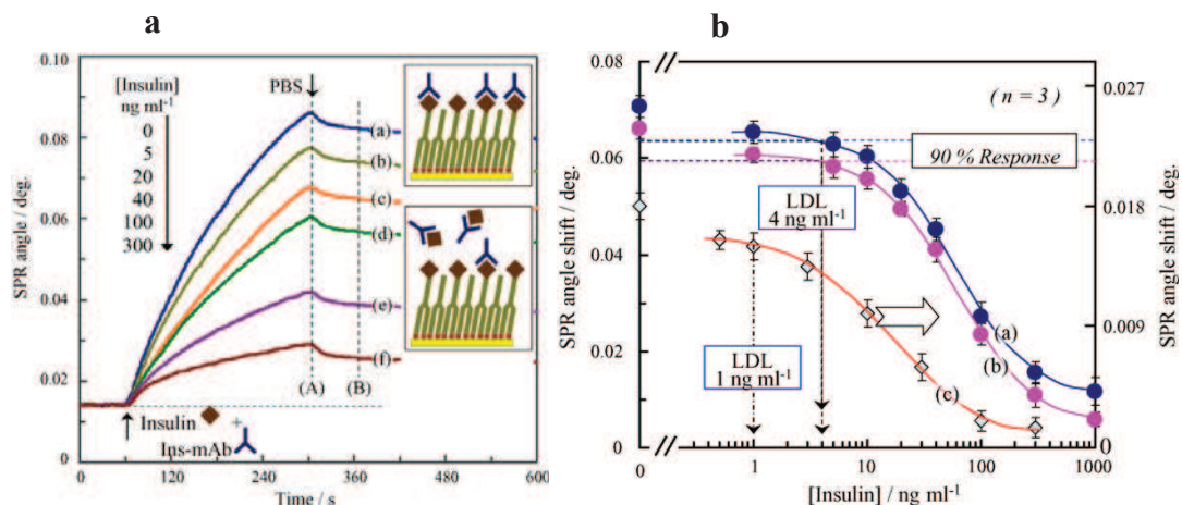
Figure I-3: a- Réponses SPR de la fixation des Ins-mAb en présence de différentes concentrations d'insuline sur la surface modifiée OEG-DCA-Ins . b- Courbes logarithmiques de la variation de l'angle SPR en fonction de la concentration en insuline. Reproduit de [25]
