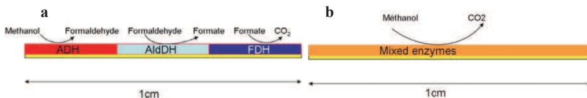
Schéma I-12 : Représentation schématique de la distribution de l'immobilisation des trois enzymes responsables de l'oxydation complète du méthanol. a- distribution successive, b- distribution aléatoire. Reproduit de [109]
