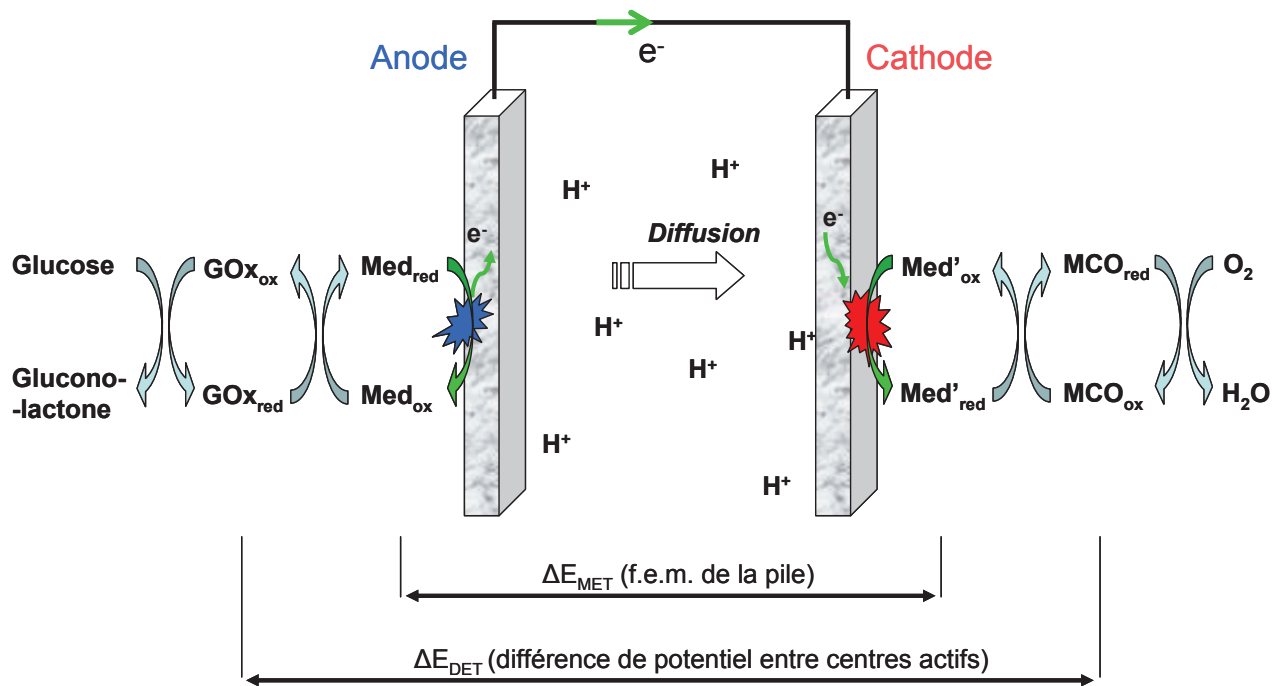
Schéma I-15 : Principe d'une biopile enzymatique à glucose/oxygène utilisant la GOx et une enzyme à base de cuivre (MCO pour Multi Copper Oxidase) comme biocatalyseurs à l'anode et à la cathode respectivement
