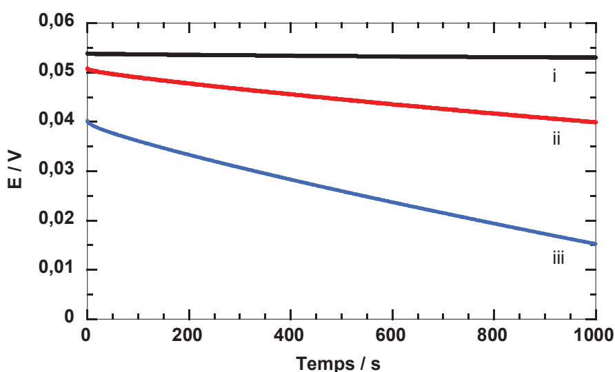
Figure III-7: Courbes de décharge de la pile 1 décrite dans la Figure III-6 soumise à la circulation de différents courants dans le circuit : i- 1 \mu A , ii- 5 \mu A , iii- 10 \mu A
