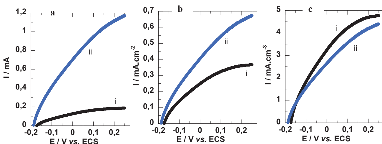
Figure IV-38: a- Courbes de polarisation anodique d'électrodes de type GC/PQ (75 :25 en masse) et de charge enzymatique GOx-Catalase/PQ (52-28 % en masse) immergées dans une solution de NaCl 0,15 mol.L -1 , HEPES 25.10 -3 mol.L -1 , glucose 5,5.10 -3 mol.L -1 (pH = 7,2, T ambiante , air saturé), b- résultats de la courbe a tracés en densité de courant, c résultats de la courbe a tracés en courant « volumique ». Diamètre des électrodes : i- Ø = 5 mm, ii- Ø = 13 mm, v b = 1 mV.s -1
