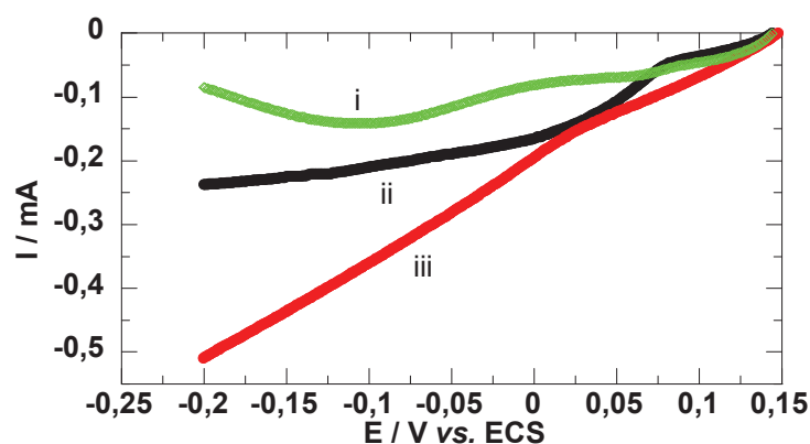
Figure IV-33: Courbes de polarisation de biocathodes compressées de type GC/TTF (ratio massique 95 :5) et un rapport de PPO/TTF de 47 % immergées dans une solution tampon de NaCl 0,15 mol.L -1 , HEPES 25.10 -3 mol.L -1 (pH = 7,2, T ambiante , air saturé) : i- Ø = 5 mm (m GC+TTF = 100 mg, sans membrane de dialyse), ii- Ø = 5 mm (m GC+TTF = 100 mg, avec membrane), iii- Ø = 13 mm (m GC+TTF = 400 mg, avec membrane), v b = 1 mV.s -1
