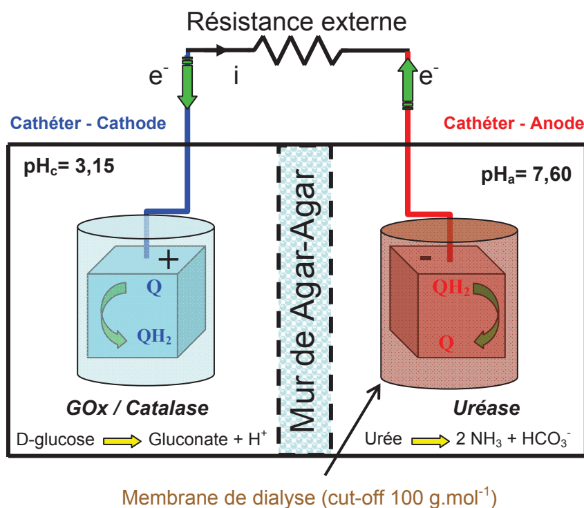
Schéma III-3: Schéma de principe du fonctionnement du prototype d'une biopile à gradient de pH basée sur des électrodes en feutre de carbone et immergée dans une solution électrolytique de \text{NaCl} 0,15 \text{ mol.L}^{-1} , glucose 5,0 \cdot 10^{-3} \text{ mol.L}^{-1} et urée 3,5 \cdot 10^{-3} \text{ mol.L}^{-1} . Les membranes de dialyse de 100 Da contiennent le couple \text{Q}/\text{QH}_2 3,2 \cdot 10^{-3} \text{ mol.L}^{-1}
