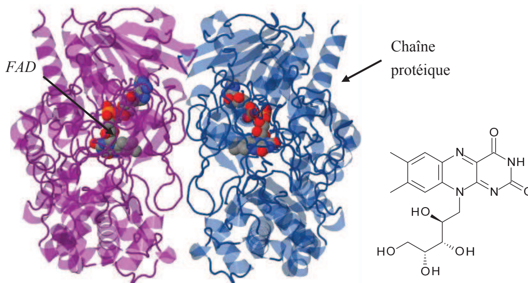
Figure I-14 : Structure tridimensionnelle de la glucose oxydase homodimérique (formée de deux sous unités identiques) composée d'une structure protéique et d'un centre rédox actif ( FAD ) par sous-unité. Structure de la riboflavine participant à l'électroactivité de la protéine. Reproduit de [141]
