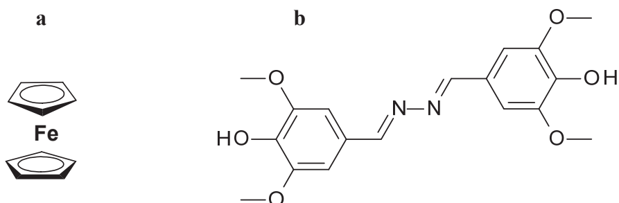
Schéma IV-3: Structure : a- du ferrocène et b- de la syringaldazine
