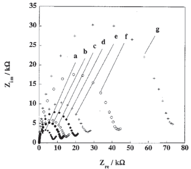
Figure I-8: Principe de l'amplification du signal de l'immunocapteur impédancemétrique pour la détection de la toxine du choléra développé par Alfonta et al. Reproduit de [57]
