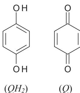
Schéma III-1 : Structure de l'hydroquinone (QH 2 ) et de la quinone (Q)
