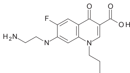
Schéma II-3: Structure du modèle de l'antibiotique ciprofloxacin
