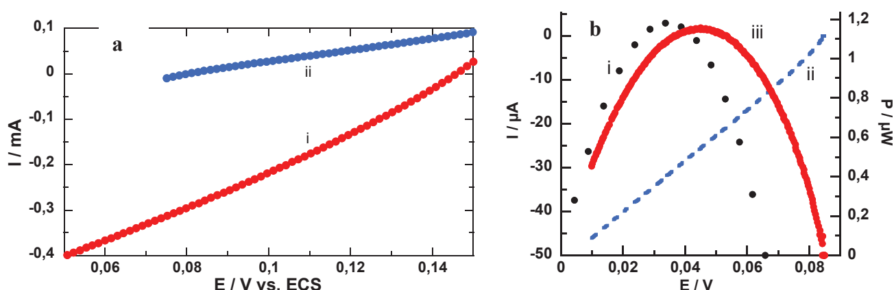
Figure IV-6: a- Courbes de polarisation i- cathodique et ii- anodique de chacune des électrodes constituant la biopile à glucose oxygène \text{QQH}_2/\text{UQ} ( \varnothing = 13\text{mm} ), i- 50 :50 GC/ \text{QQH}_2 ; PPO/ \text{QQH}_2 3 %, ii- 66 :33 GC/UQ ; GOx-Catalase/UQ 13-6 %, immergées dans une solution électrolytique de NaCl 0,15 mol.L -1 , HEPES 25.10 -3 mol.L -1 et glucose 5,5.10 -3 mol.L -1 (pH = 7,2, T_{\text{ambiante}} , air saturé), v_b = 5 \text{ mV.s}^{-1} . b- i- Courbe de puissance théorique construite à partir des courbes de polarisation, ii- courbe de polarisation de la pile après 24 heures d'immersion et iii- courbe de puissance issue de la courbe de polarisation précédente
