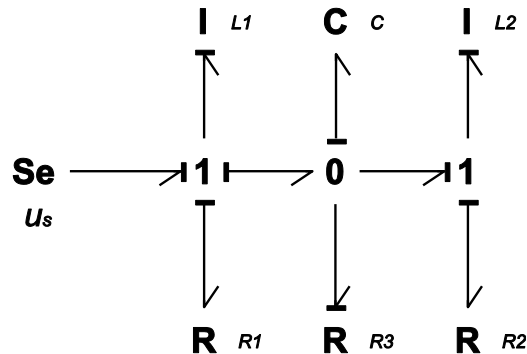
Figure ;Error! Utilice la ficha Inicio para aplicar Titre 2 al texto que desea que aparezca aquí..8 Bond graph avec l'élément parasite.
