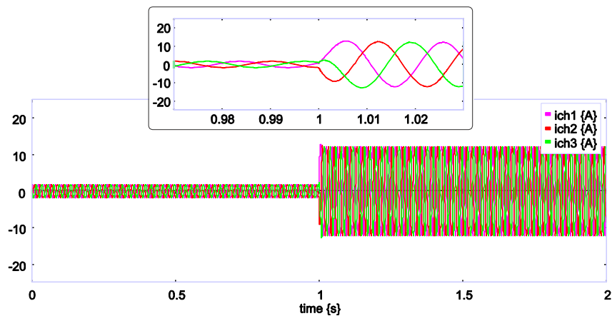
Figure 3.17 Courants à la charge.
