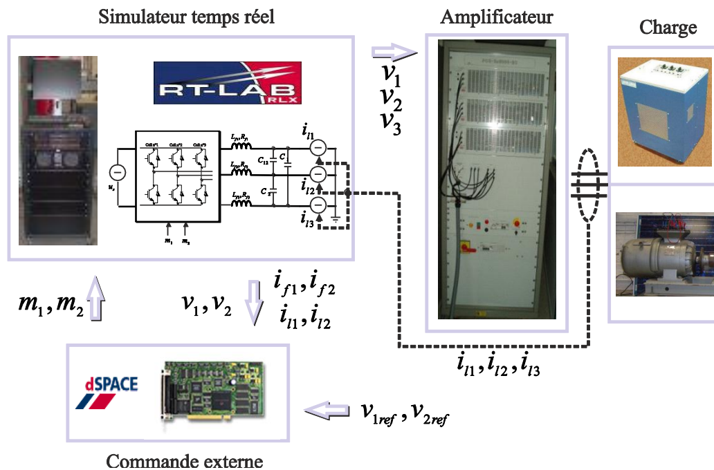
Figure 3.19 Schéma de la mise en œuvre expérimentale.
