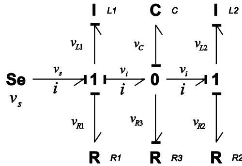
Figure 1.12 BG avec l'élément parasite.
