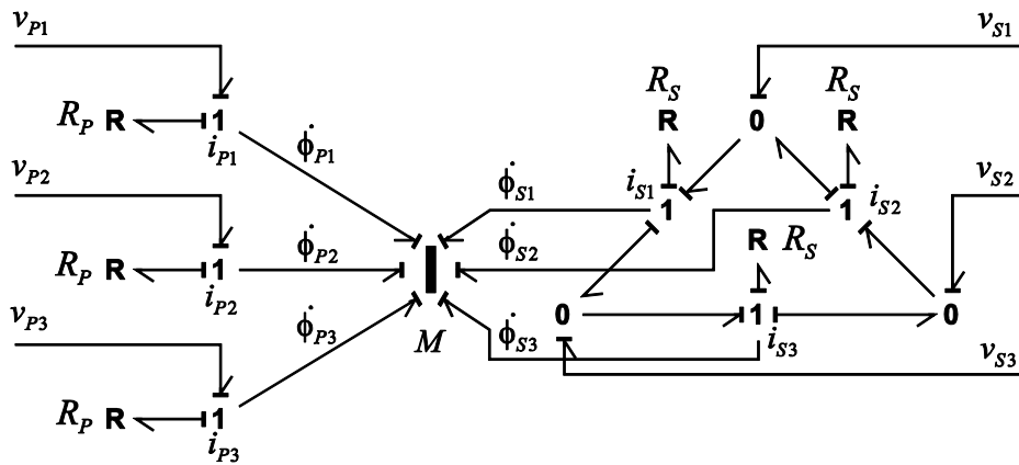
Figure 2.6 Transformateur triphasé connexion Yd.
