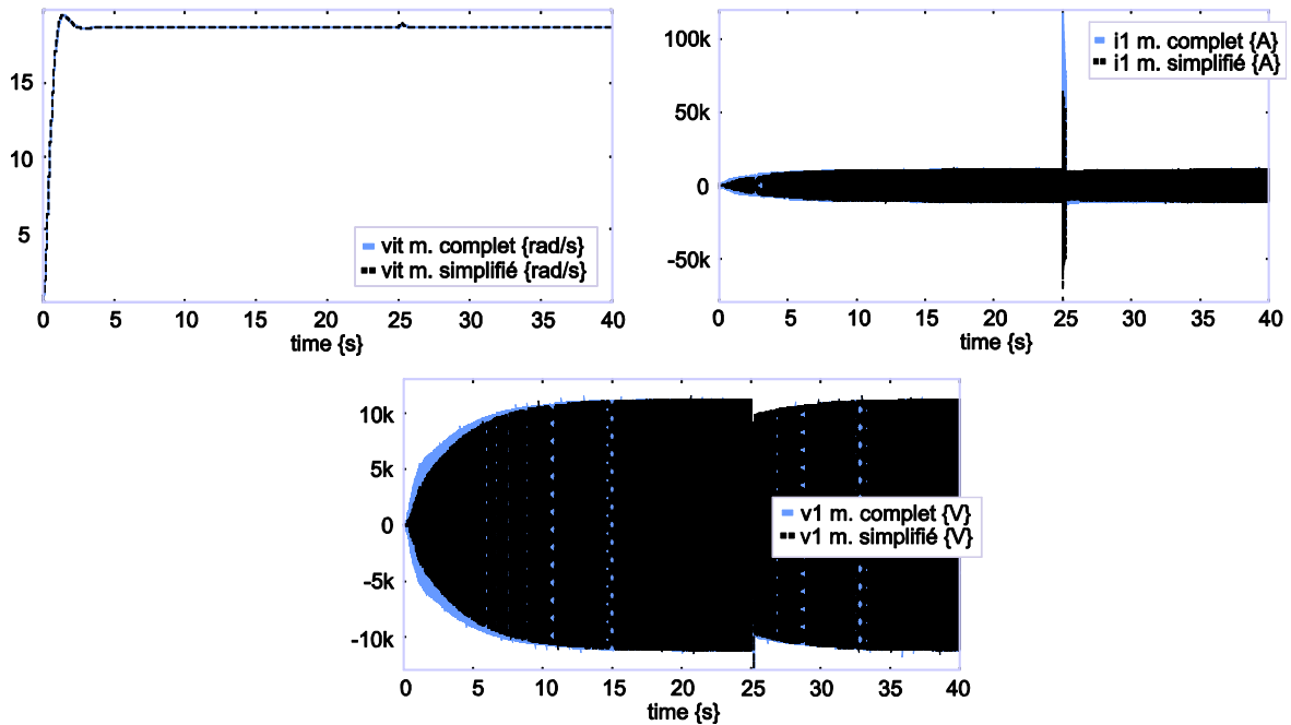
Figure 2.27 Résultat de la simulation du modèle complet et simplifié de la machine synchrone.
