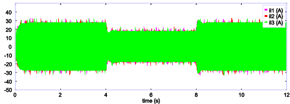
Figure 3.43 Courants injectés sur le réseau.
