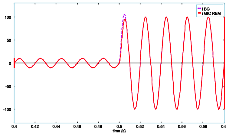
Figure.1.35 Courant de sortie pour la comparaison via simulation.
