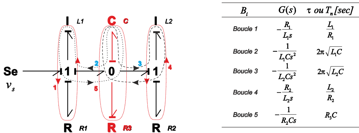
Figure ;Error! Utilise la fiche Inicio para aplicar Titre 2 al texto que desea que aparezca aquí..9 Boucles causales dans de bond graph.
