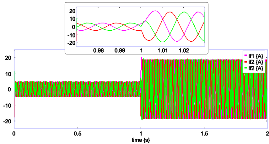
Figure 3.16 Courants triphasés dans le filtre du convertisseur.
