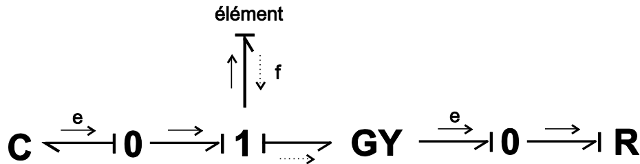
Figure ;Error! Utilisez la fiche Inicio para aplicar Titre 2 al texto que desea que aparezca aquí..3 Chemin causal indirect.
