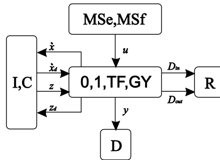
Figure ;Error! Utilice la ficha Inicio para aplicar Titre 2 al texto que desea que aparezca aquí..6 et structure d'un bond graph.
