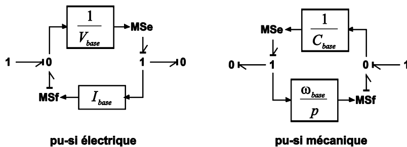
Figure 2.24 Schéma à l'intérieur du block de conversion.
