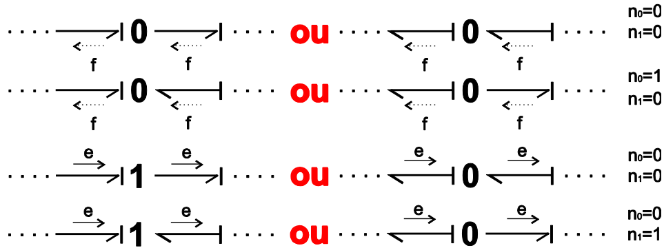
Figure ;Error! Utilisez la fiche Inicio para aplicar Titre 2 al texto que desea que aparezca aquí..2 Exemples pour le calcul de n_0 et n_1 .
