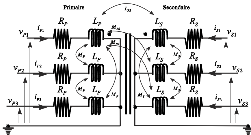
Figure 2.4 Schéma électrique du transformateur triphasé Yy.
