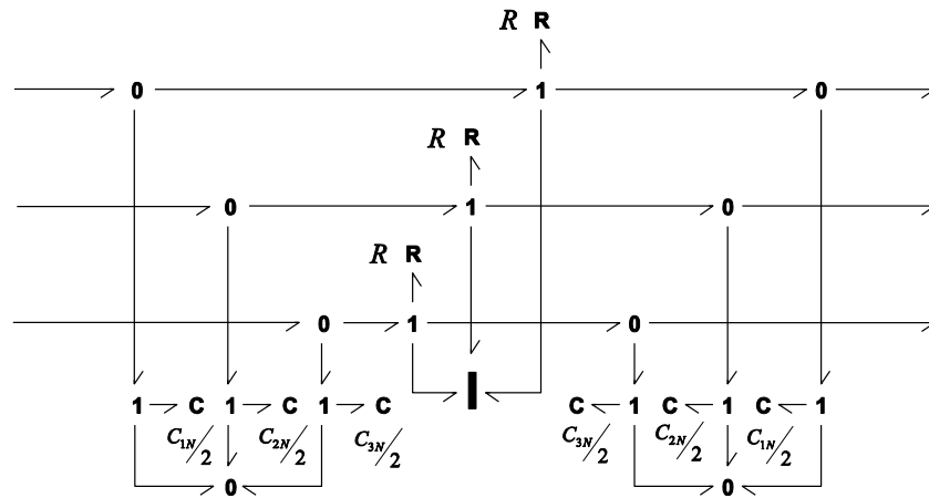
Figure 4.23 Bond graph acausal de la ligne de transmission couplée.
