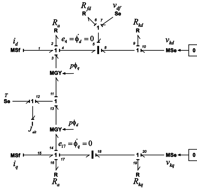
Figure 2.21 Machine synchrone sans dérivées de flux statiques, tension sortie.
