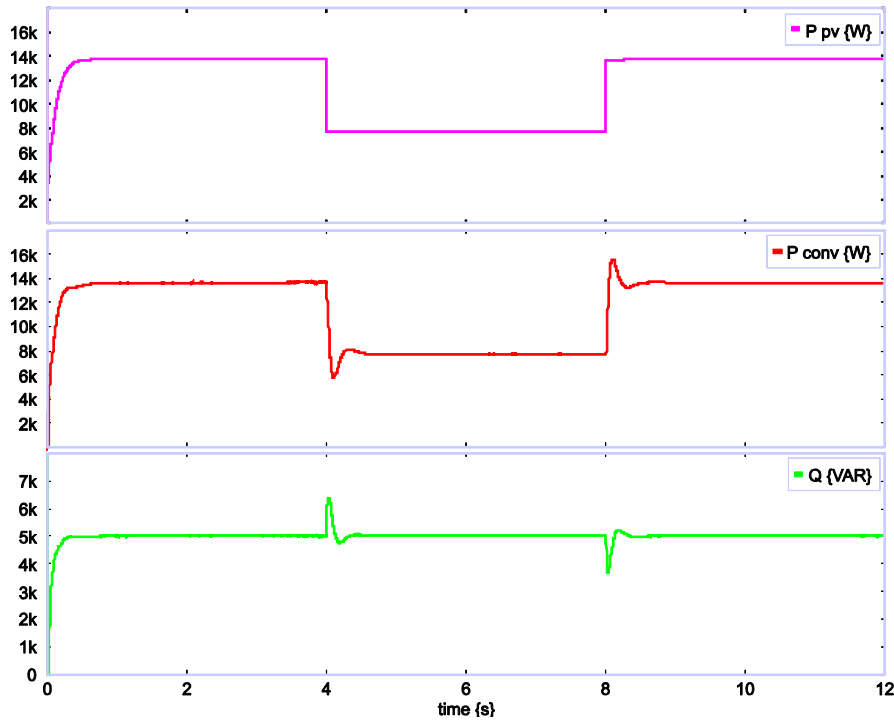
Figure 3.41 Puissances du panneau (pv) et du convertisseur ( P_{conv} , Q ).
