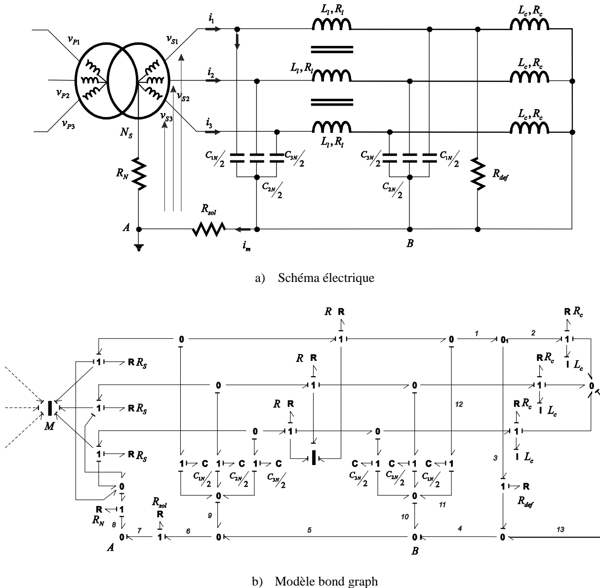
Figure 4.24 Transformateur + Ligne de transmission + défaut.
