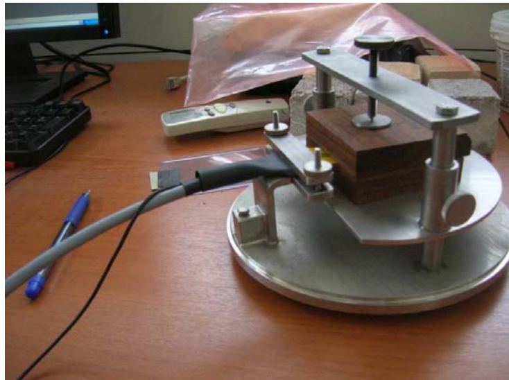
Figure 21 : Mesures de propriétés thermiques du bois
