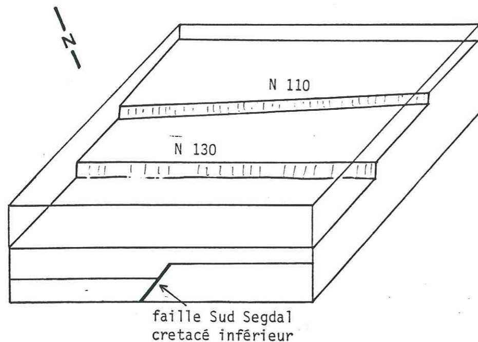
Fracturation cénomanienne N 110- N 130 en extension au sein de l'unité Oued Defla.
