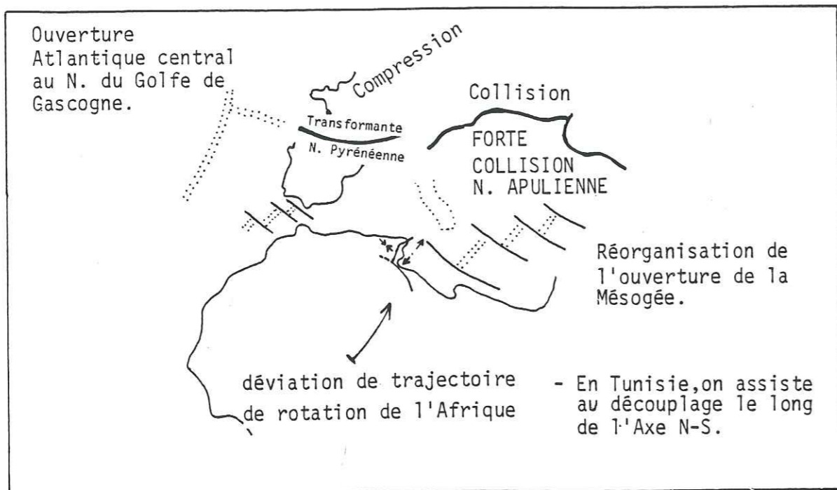
Fig. 163 La crise Sènonienne (- 83 à - 80 Ma), (d'après Olivet, 1978 et Dercourt, 1985).
