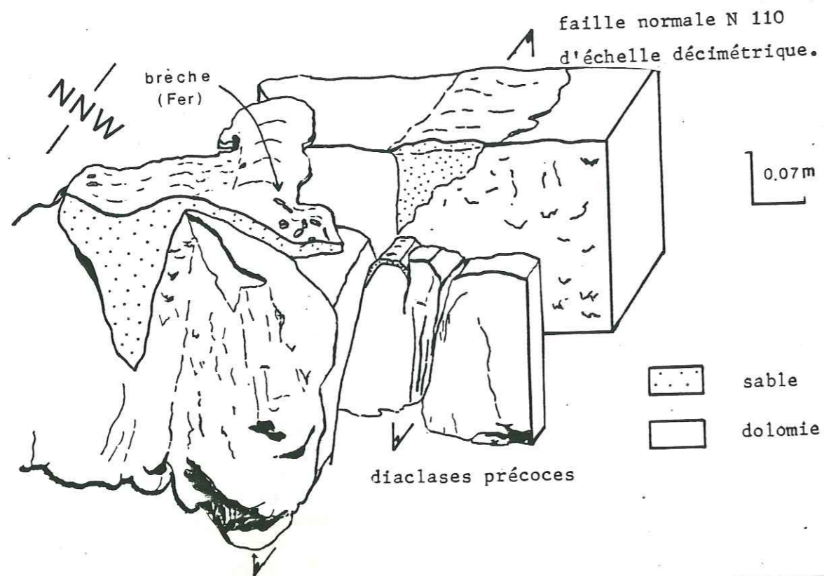
Fig. 60 (vue de détail de la fig 55) Diaclases précoces N 85 - N 110, à la base de la dernière séquence de la formation Meloussi (oued Defla). Ces diaclases sont situées à l'extrados du roll-over et du crochon associés aux fa- illes normales N 65 et N 70 (fig. 52). Les diaclases ont été ouvertes lors du peu synsédimentaire de cette famille de failles normales. Puis elles ont été en- croûtées de fer et enfin colmatées par du sable. Elles résultent de la fractu- ration en extension hauterivienne.
