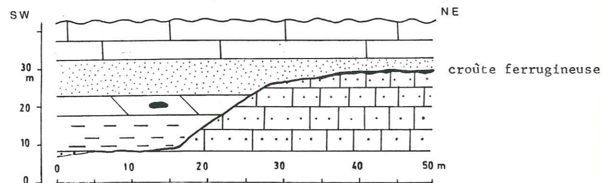
Fig. 46 Paléo-abrupt du Crétacé inférieur de l'unité Segdal-Defla (oued Brahim). Il est actif depuis l'Hauterivién et est ennoyé par la Formation Orbata supérieur (gargasien). La croûte ferrugineuse de la partie orientale de cet escarpement, représente la période asédimentaire de ce domaine. Ce dispositif est accompagné d'une troncature de la Formation Meloussi. Celle-ci est scellée par la Formation Orbata supérieure.
