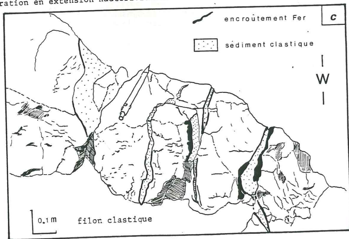
Fig. 60 (vue de détail de la fig 55) Diaclases précoces N 85 - N 110, à la base de la dernière séquence de la formation Meloussi (oued Defla). Ces diaclases sont situées à l'extrados du roll-over et du crochon associés aux fa- illes normales N 65 et N 70 (fig. 52). Les diaclases ont été ouvertes lors du peu synsédimentaire de cette famille de failles normales. Puis elles ont été en- croûtées de fer et enfin colmatées par du sable. Elles résultent de la fractu- ration en extension hauterivienne.
