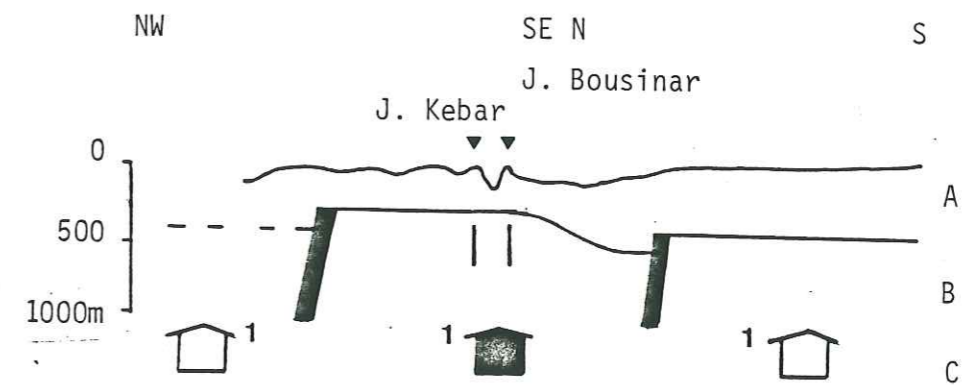
A - courbe de subsidence de l'intervalle Paleocène-Eocène (16 Ma). B - comportement des structures profondes : - rides salifères atlasiques - Limites du bloc atlasique peu actives. C - comparaison avec l'étape précédente : - soulèvement généralisé
