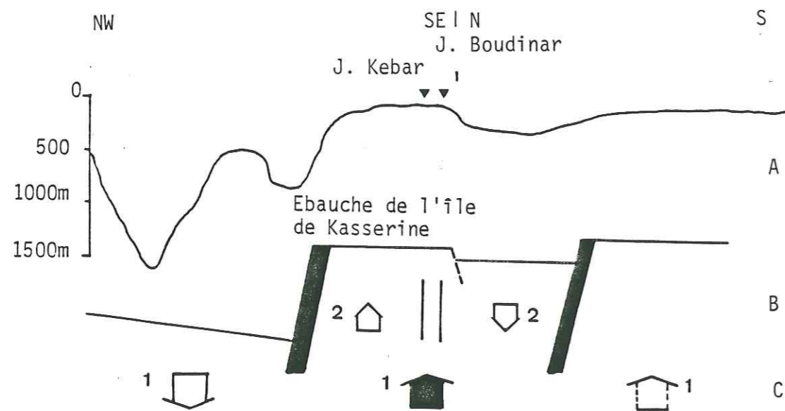
A - courbe de subsidence de l'intervalle Coniacien-Santonien (14 Ma). B - comportement des structures profondes : - subsidence du sillon tunisien - ébauche de l'île de Kasserine - faible jeu de la limite sud du bloc atlasique. C - comparaison avec l'étape précédente: inversion de subsidence du sillon tunisien.
