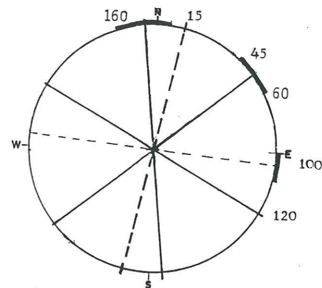
LE RESEAU DE FRACTURATION ( failles et diaclases) DU VRACONIEN-CENOMANIEN. ( formations Fahdène-Zebbag)
