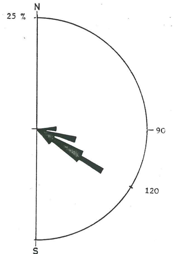
* coin éffondré par le jeu concomittant de petites failles N 90 et N 120. Fig. 64 Diaclases precoces associées N 90- N 120 au toit de la formation Meloussi ( oued Defla ), lors de l'extension hauterivienne.
