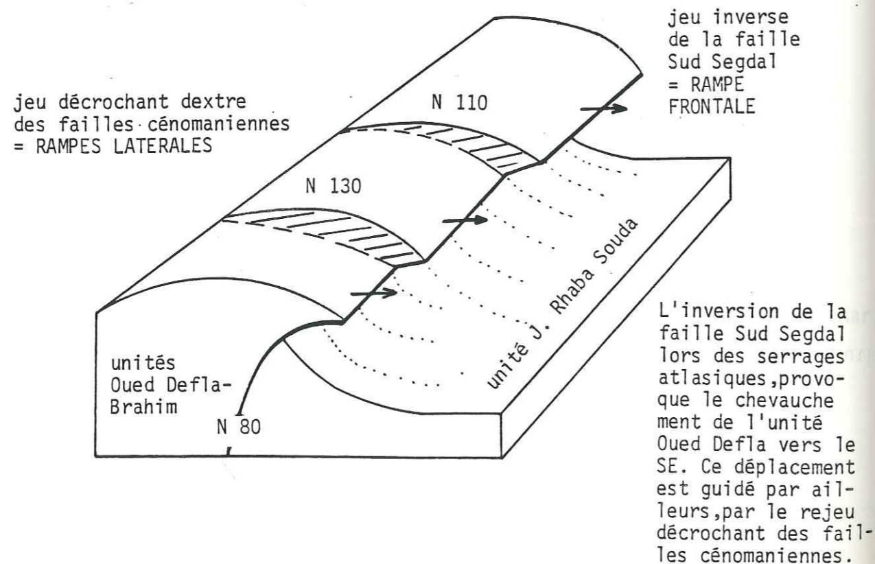
Fig. 130 Serrages atlasiques de paleofailles normales du Crétacé inférieur et du Cénomaniens = jeu selon rampe frontale et rampe latérale.
