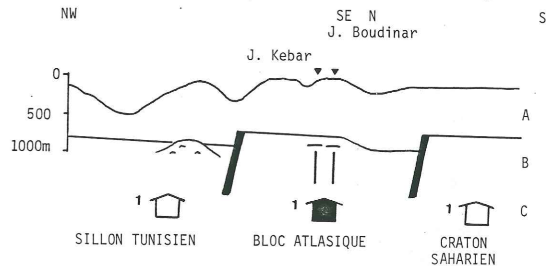
A - courbe de subsidence du Campanien-Maastrichtien (11 Ma). B - comportement des structures profondes - sillon tunisien subsident - soulèvement du bloc atlasique - persistance de l'effondrement du fossé de Gafsa = jeu de la limite sud du bloc atlasique. C - comparaison avec l'étape précédente : - soulèvement généralisé, événement majeur
