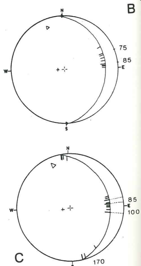
Fig. 52 Fracturation synsédimentaire N 70, en extension, à la base de la dernière séquence sable- dolomie de la Formation Meloussi.
