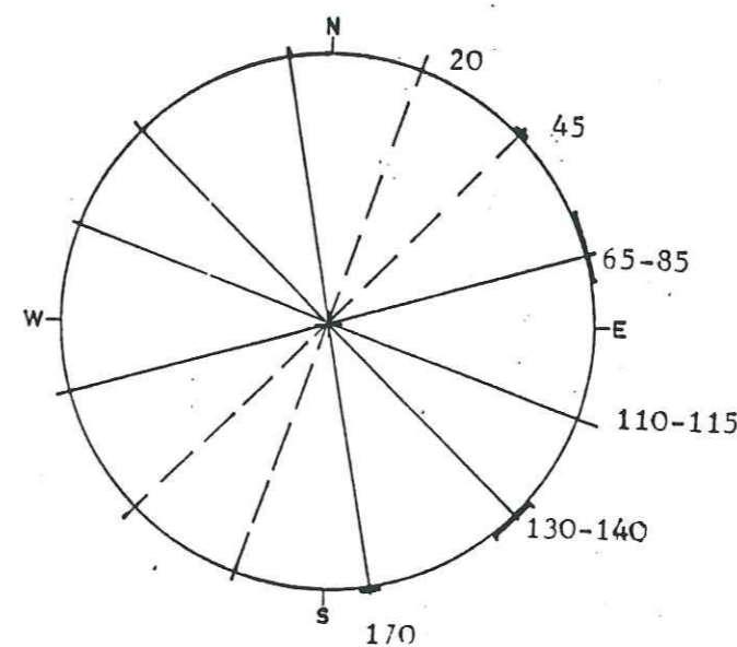
LE RESEAU DE FRACTURATION ( diaclases essentiellement) A LA FIN DU GARGASIEN ( toit de la formation Orbata supérieur , sous les marnes de la formation Fahdène).
