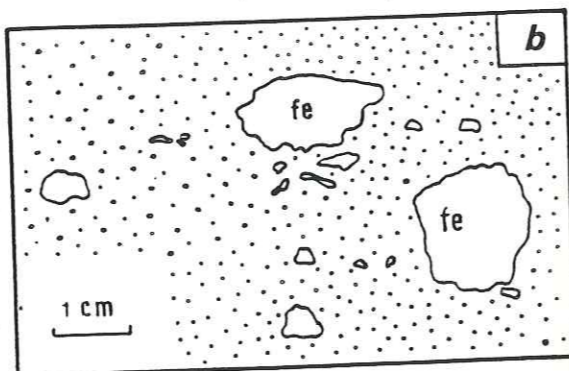
Fig. 60 (vue de détail de la fig 55) Diaclases précoces N 85 - N 110, à la base de la dernière séquence de la formation Meloussi (oued Defla). Ces diaclases sont situées à l'extrados du roll-over et du crochon associés aux fa- illes normales N 65 et N 70 (fig. 52). Les diaclases ont été ouvertes lors du peu synsédimentaire de cette famille de failles normales. Puis elles ont été en- croûtées de fer et enfin colmatées par du sable. Elles résultent de la fractu- ration en extension hauterivienne.
