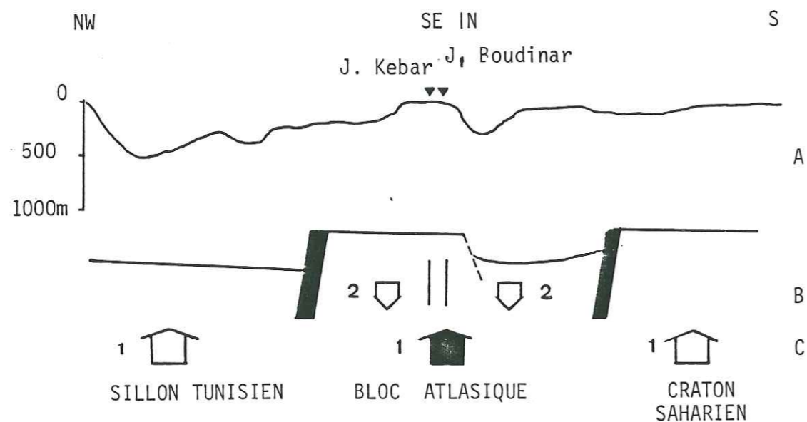
A - courbe de subsidence de l'intervalle Turonien inf. et moyen, (4 Ma). Regression et faible épaisseur de dépôt. B - comportement des structures profondes: faible subsidence soulèvement généralisé ? C - comparaison avec l'étape précédente : tendance au soulèvement de l'ensemble de la Tunisie . Ebauche de la crise du Turonien terminal ?
