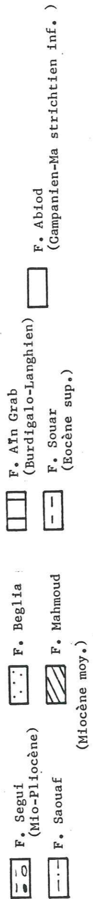
Fig; 110 Les discordances successives de la série tertiaire sur le flanc Nord du J. Boudinar. Les discordances en éventail au sein de la Formation Segui attestent du soulèvement progressif de l'anticlinal du J. Boudinar, au cours du Mio-Pliocène.
