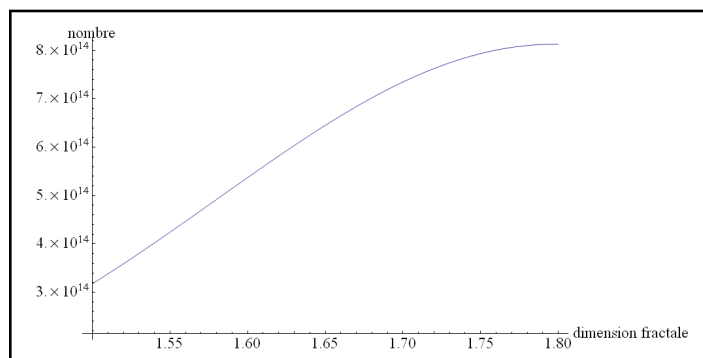
Figure 82. Relation exponentielle entre la dimension fractale et le nombre de boîtes comptées
