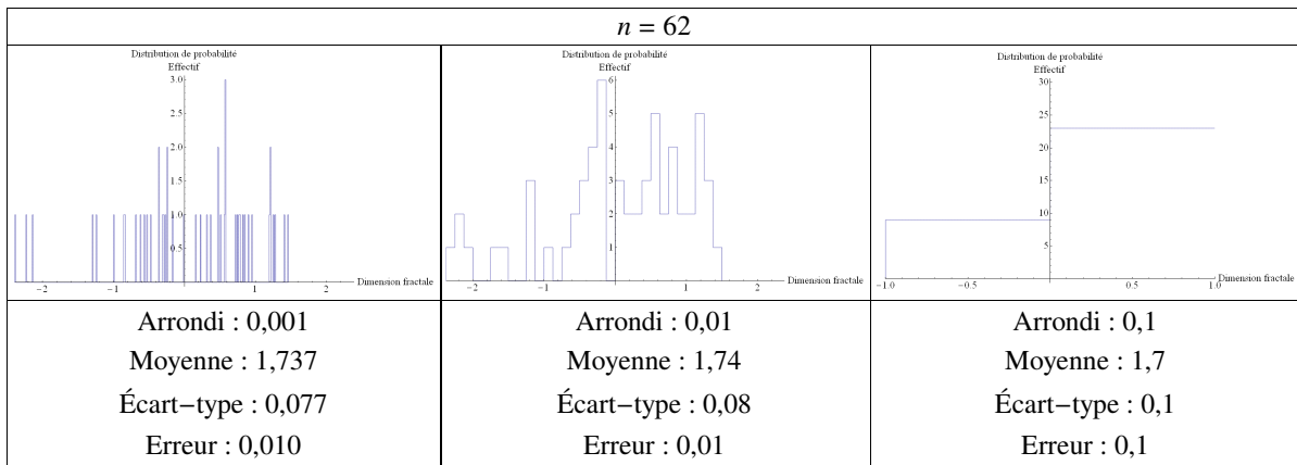
Figure 67. Distribution de probabilité de la dimension fractale centrée et réduite de la base de Christopher Small
