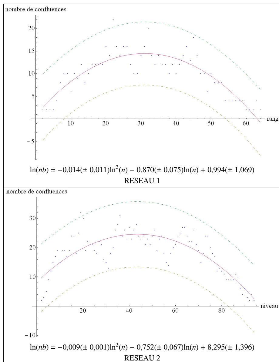
Figure 51. Arborescence : modèle parabolique observé
