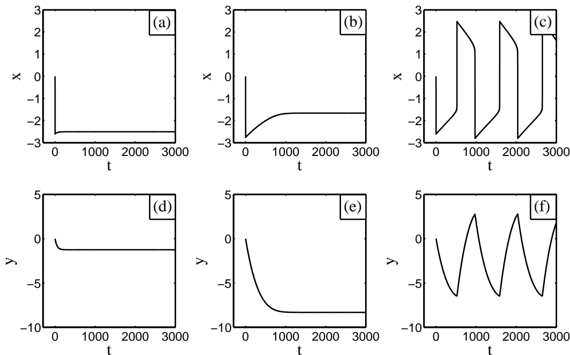
FIG. 2.2 – Différentes formes d'ondes correspondant aux trois régimes de fonctionnement du système de FitzHugh-Nagumo pour la même condition initiale x(t=0)=0 , y(t=0)=0 . Paramètres du système : a = 2.03 , b = -2.53 , A = 0 et \epsilon = 0.01 . (a,d) Régime bistable obtenu pour (\gamma, Z)=(2, -1) ; (b,e) régime excitable obtenu pour (\gamma, Z)=(0.2, -3) et (c,f) régime oscillant obtenu pour (\gamma, Z)=(0.2, -1) .
