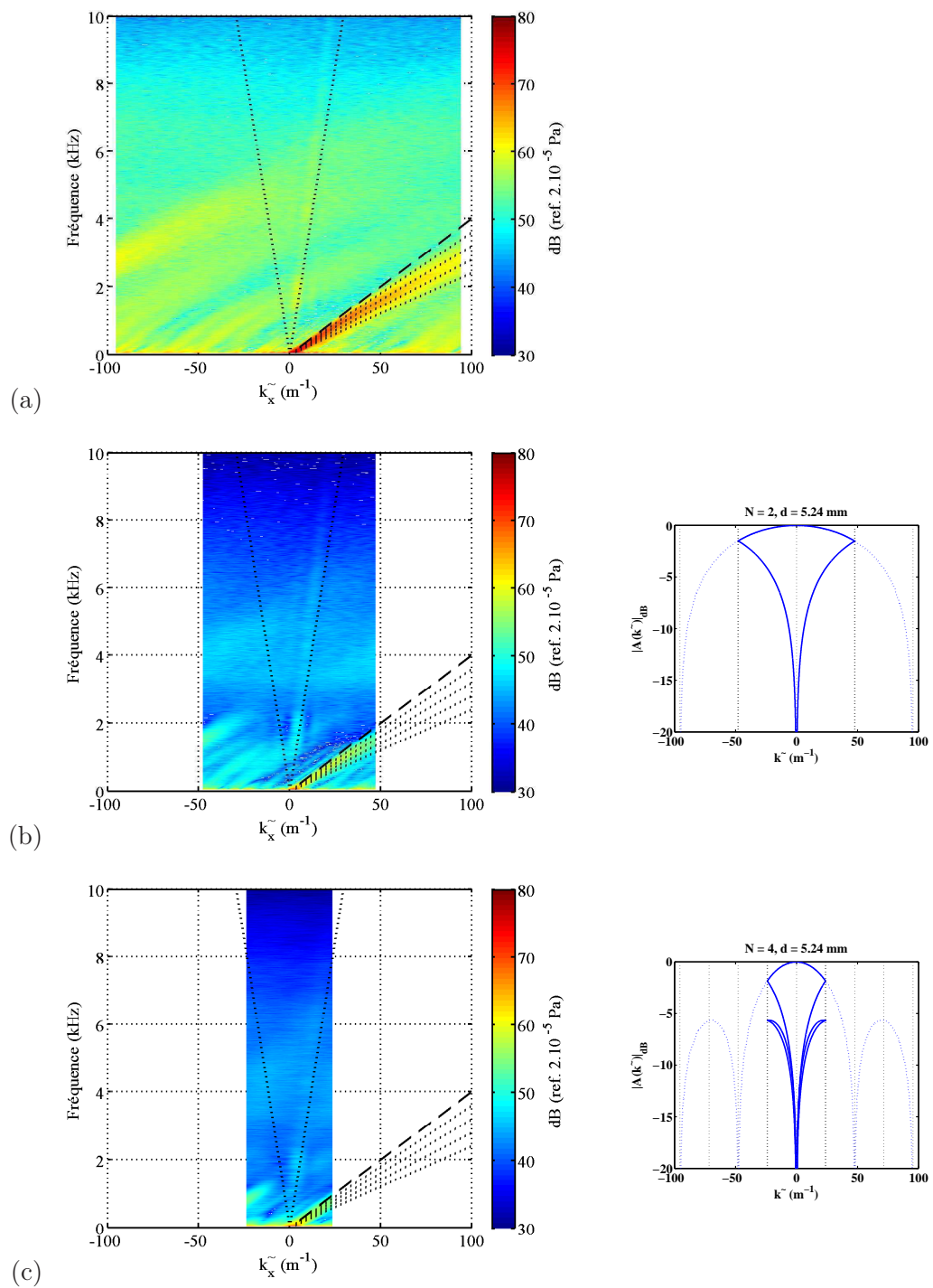
Figure IV.9 – Modules des spectres en nombre d’onde–fréquence \Phi(\tilde{k}, f) des signaux de la CLT avec source LMS non-filtrés (a) et filtrés par Somme de paires (b) ou de quadruplets (c) de capteurs. A droite sont rappelées les réponses en nombre d’onde de chaque type de filtrage, effet du repliement inclus.
