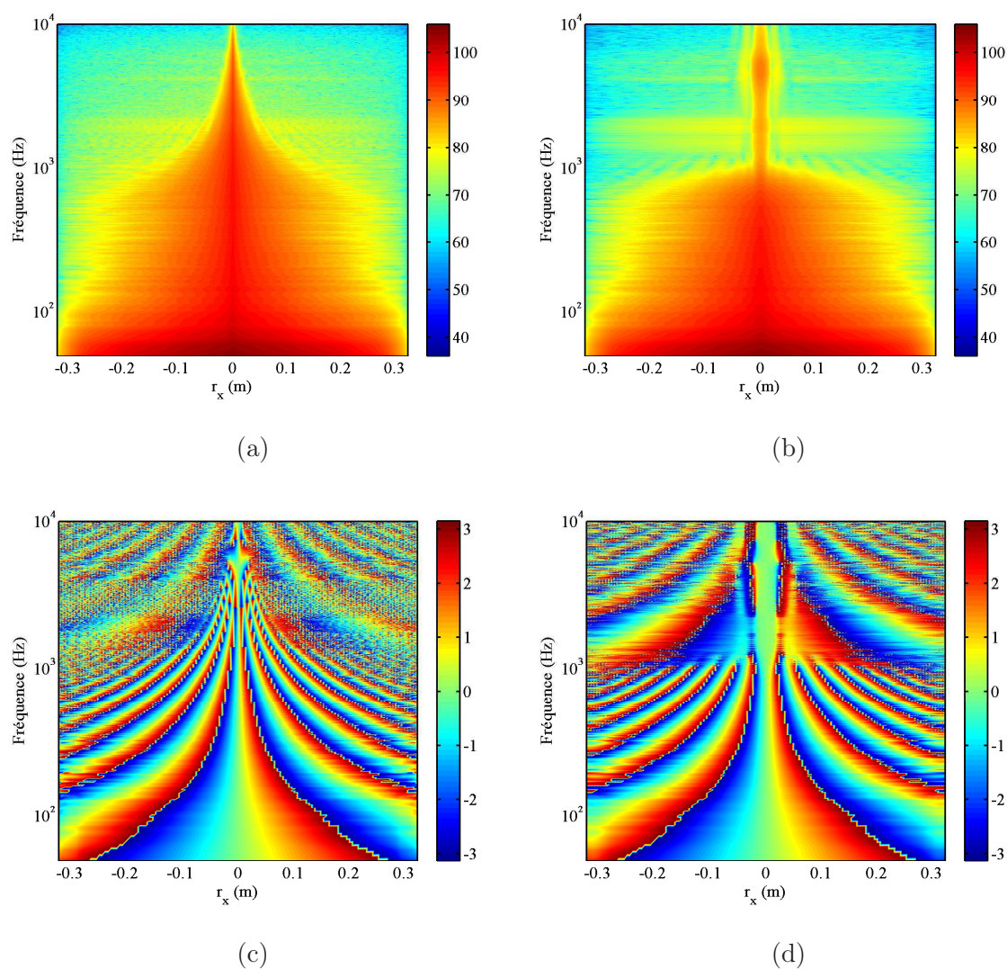
Figure IV.12 – Modules (en dB réf. 2 \cdot 10^{-5} Pa) et phases (en radian) des interspectres (non-référencés) pour la CLT avec la source LMS en position 4 avant et après application de la sEMD. Modules en haut (a)-(b), phases en bas (c)-(d). Interspectres avant sEMD à gauche (a)-(c), après sEMD à droite (b)-(d).
