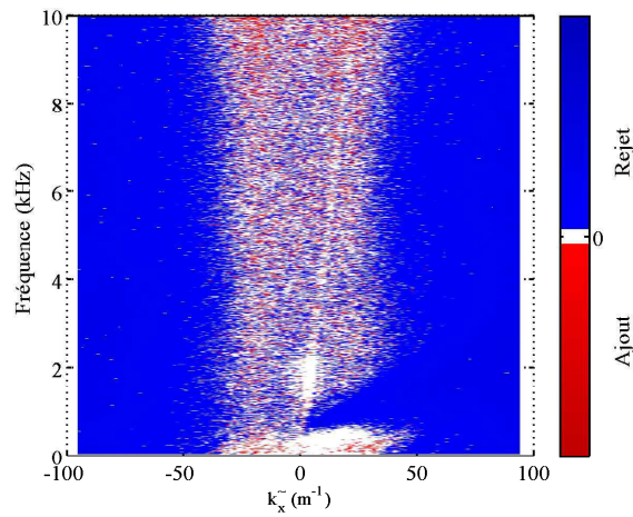
Figure IV.15 – Bilan énergétique de l'application de la sEMD pour la CLT avec source LMS en position 4.
