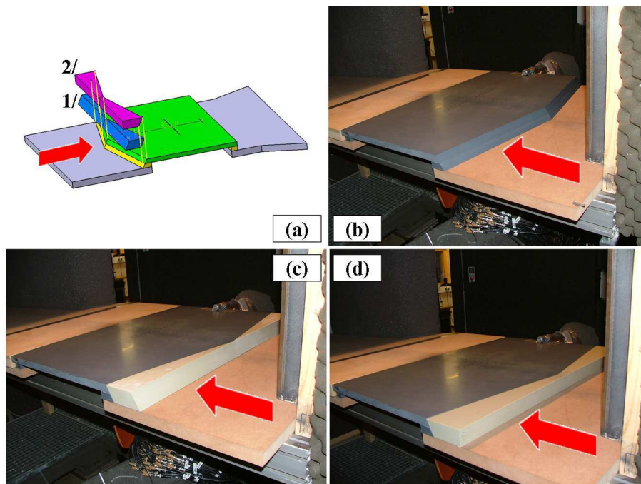
Figure II.9 – Vues des configurations marche montante. Le schéma (a) présente la marche montante dite “en chevron” (photographie (b)) sur laquelle s’ajoutent des modules permettant d’obtenir respectivement une marche inclinée sans dérapage (modules 1/ sur (a) et photographie (c)), ou droite sans dérapage (modules 2/ sur (a) et photographie (d)). La flèche indique le sens de l’écoulement.
