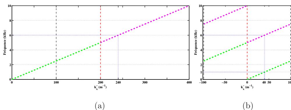
Figure III.10 – Illustration du principe de repliement : phénomène caractérisé par une vitesse de phase de 25 m.s^{-1} , représenté sans (a) et avec (b) repliement. Ici, \tilde{k}_{max} = 200 m^{-1} .
