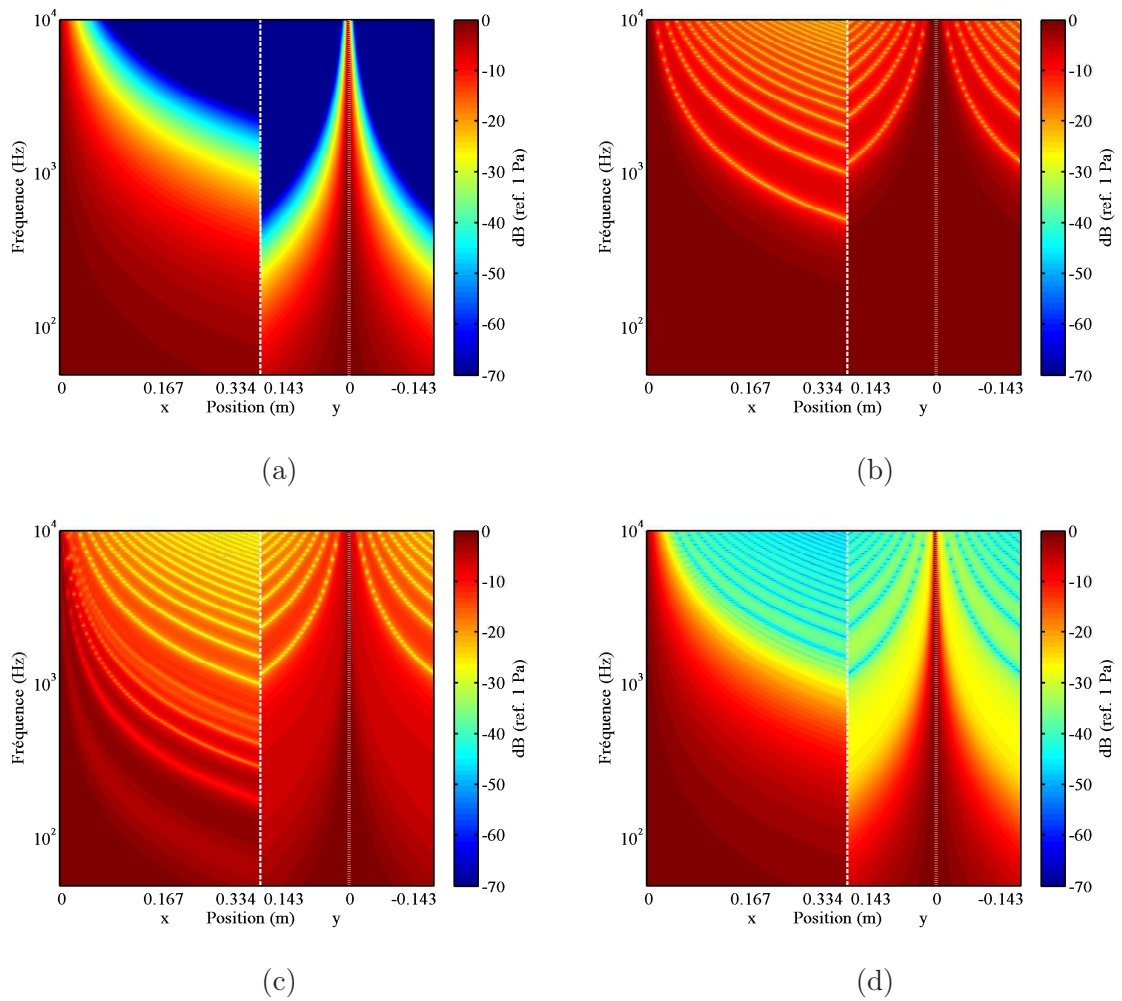
Figure III.6 – Modules (en dB réf. 1 Pa) de diverses simulations d'interspectres référencés : (a) modèle de Corcos, (b) modèle du champ diffus, (c) et (d) combinaisons des deux modèles de rapport énergétique r_{ac} = 1 (c) et r_{ac} = 1/100 (d).
