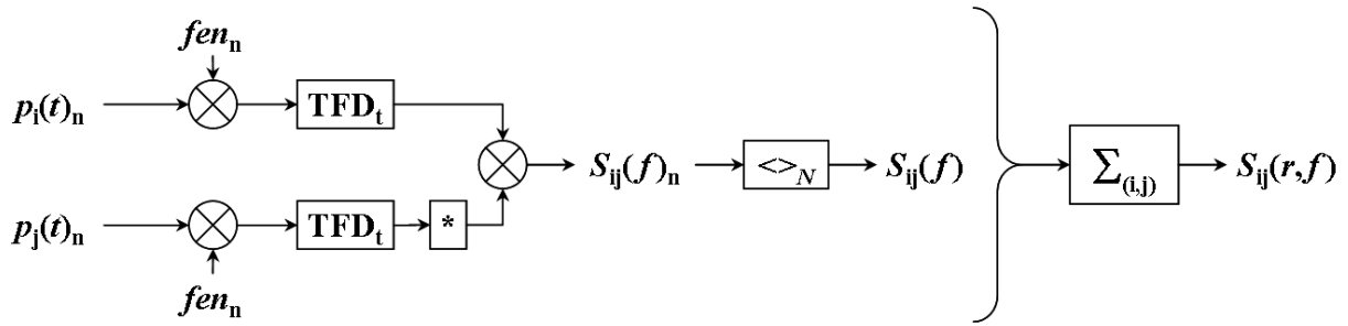
Figure III.5 – Algorithme de calcul d'une matrice interspectrale.
