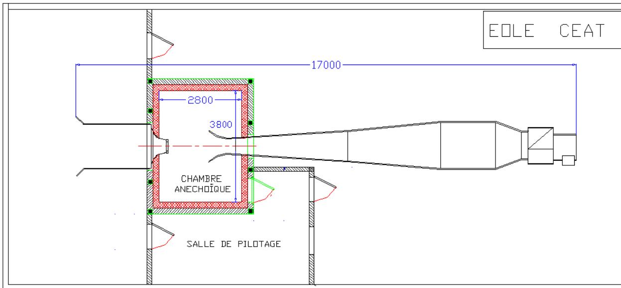
Figure II.1 – Schéma de la soufflerie EOLE. L'écoulement se fait de gauche à droite.
