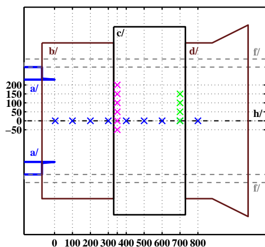
Figure IV.1 – Positions \times des profils de vitesse par rapport aux plaques. Les étiquettes a/ à h/ sont identiques à celles de la figure II.5 page 30.
