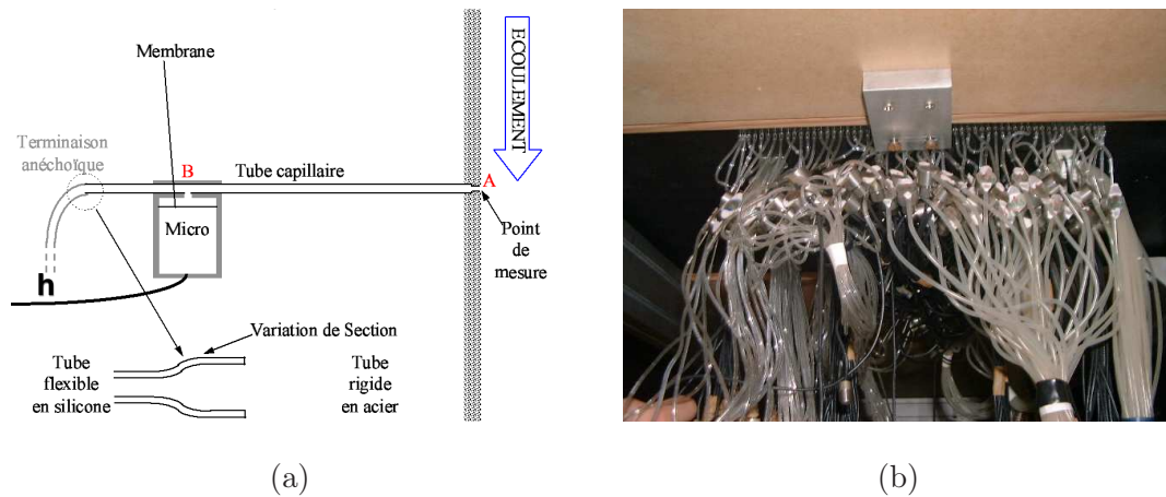
Figure II.19 – Schéma (a) et photo (b) des microphones déportés.
