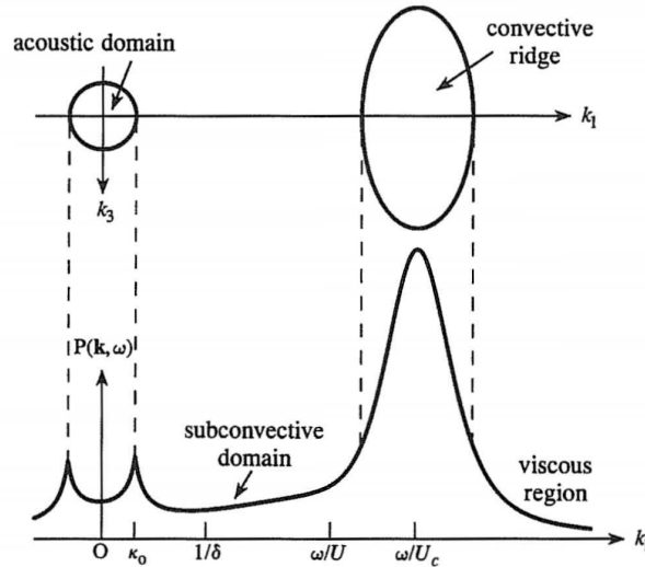
Figure I.6 – Spectre en nombre d'onde–fréquence de pression pariétale d'une couche limite turbulente à faible nombre de Mach à une fréquence donnée (d'après Howe 1998 [54]). Le pic convectif et le domaine acoustique sont clairement identifiables.
