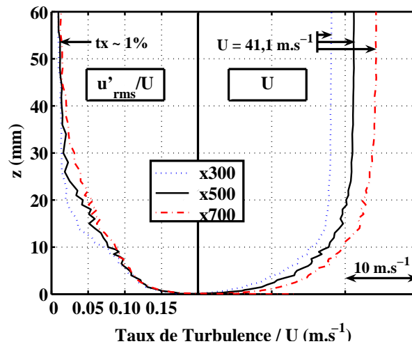
Figure II.2 – Profils de vitesse U (à droite) et taux de turbulence u'_{rms}/U associés (à gauche) pour trois positions x (à 300, 500, 700 mm du convergent). La partie gauche présente les trois taux de turbulence, la partie droite, les profils de vitesse moyenne U , décalés pour plus de lisibilité.
