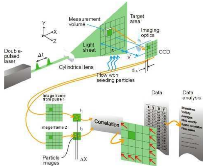
Figure II.16 – Principe de la PIV, tiré du site de © DANTEC DYNAMICS [23]
