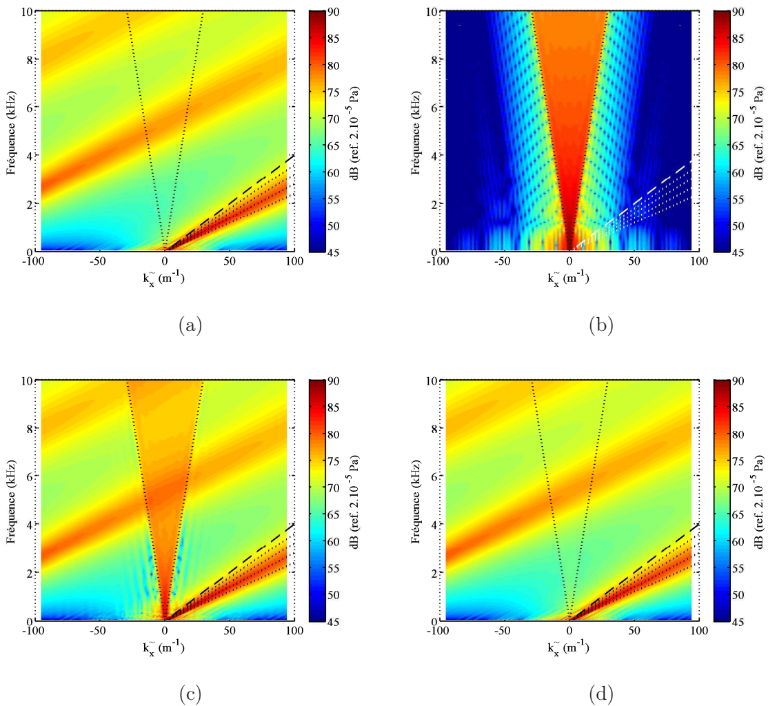
Figure III.11 – Modules (en dB réf. 2.10^{-5} Pa) des simulations de spectres en nombre d'onde–fréquence \Phi(\tilde{k}_x, f) : (a) modèle de Corcos, (b) modèle du champ diffus, (c) et (d) combinaisons des deux modèles de rapport énergétique r_{ac} = 1 (c) et r_{ac} = 1/100 (d).
