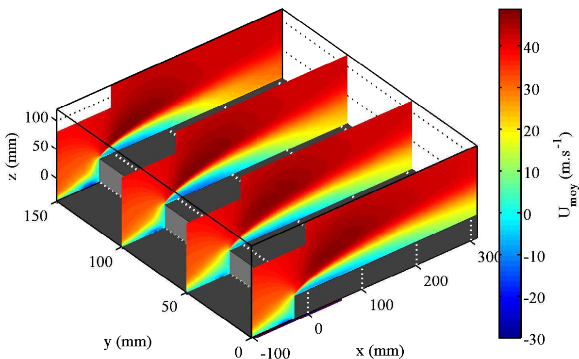
Figure 9 – Visualisations de la vitesse moyenne longitudinale U_{moy} par PIV sur la marche droite M1D.
