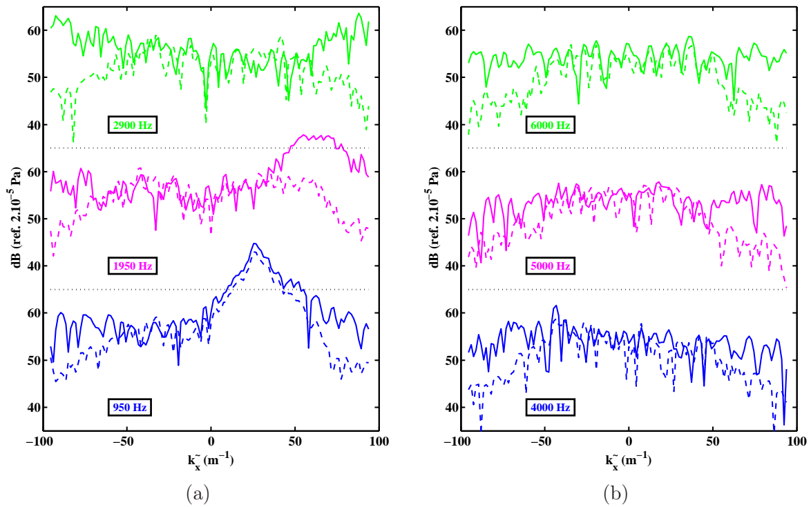
Figure IV.19 – Coupes en fréquence des spectres avant (trait plein) et après (tirets) application de la sEMD pour la CLT seule.
