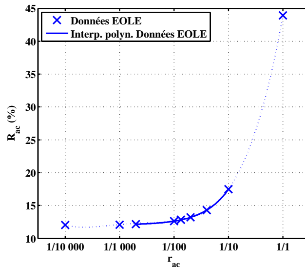
Figure IV.8 – Courbe de correspondance des seuils énergétiques r_{ac} et R_{ac} .
