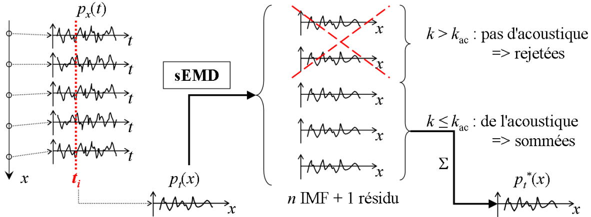
Figure III.15 – Illustration du principe de filtrage spatial par sEMD.
