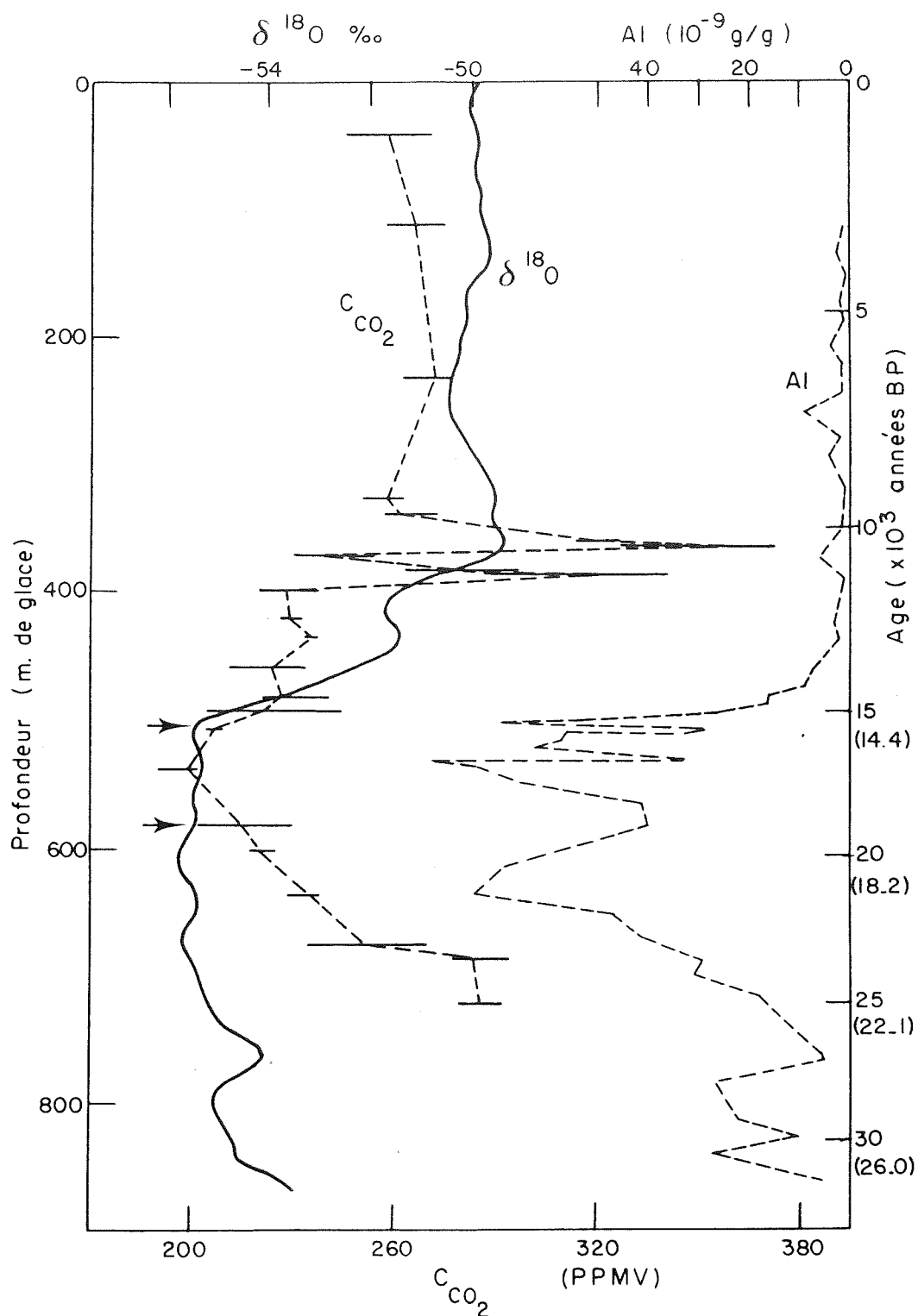
Figure 32 : DOME C Profil des teneurs en CO_2 (piégeage rapide) et les autres paramètres climatiques (aluminium et \delta^{18}O Petit et al.1981, Lorius et al. 1979)
