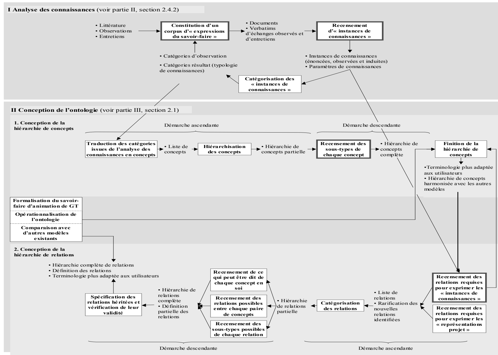
FIG. A.6 – Méthode de conception de l'ontologie OCM (processus complet) - voir signification des étapes encadrées en gras en 4.3.2
