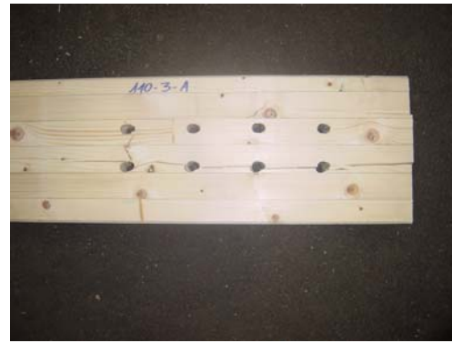
Rupture de bloc
