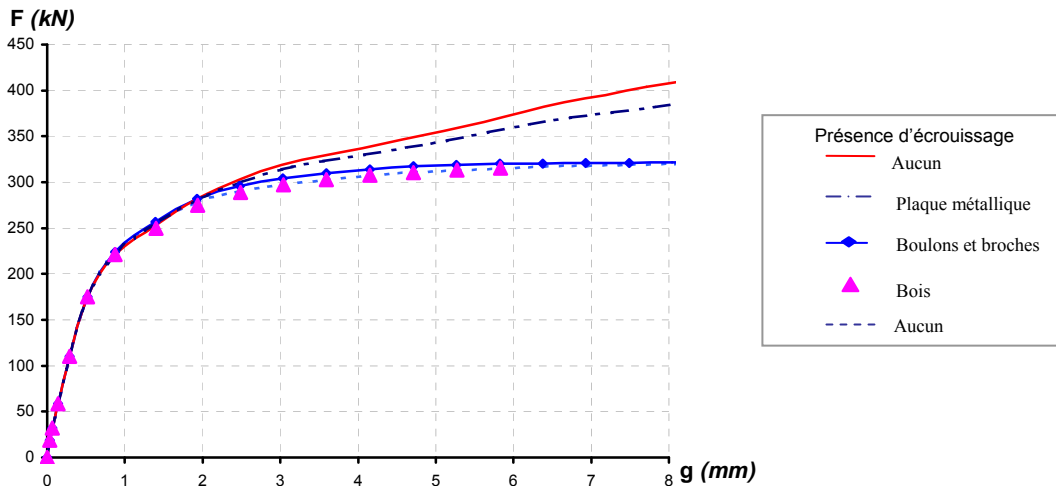
Figure B.30 : Influence de l'écrouissage sur le comportement global de l'assemblage
