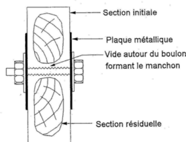
Figure A.39 : Formation d'un manchon autour du boulon [LOG 98]
