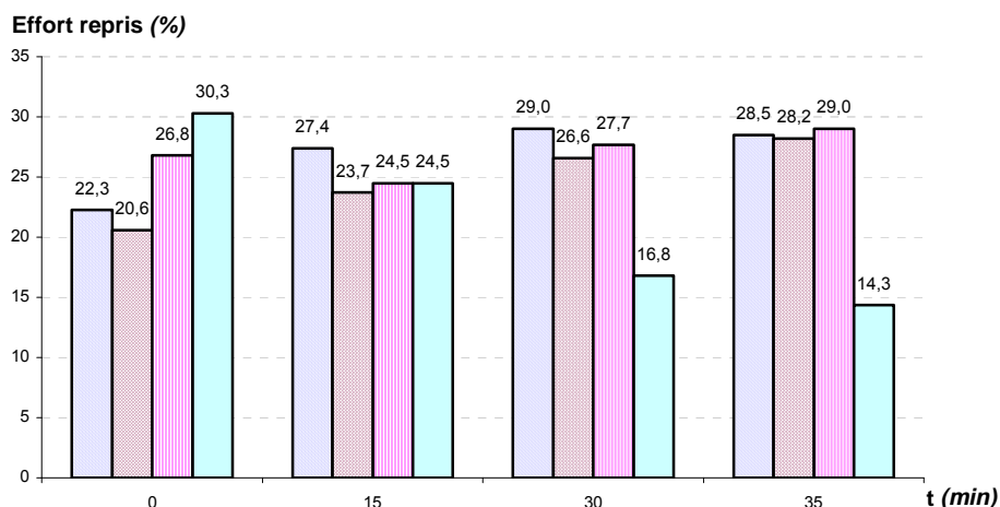
Figure C.33 : Répartition des efforts repris par les organes d'assemblage en fonction de la durée d'exposition au feu ( t_{fi} = 40 min)
