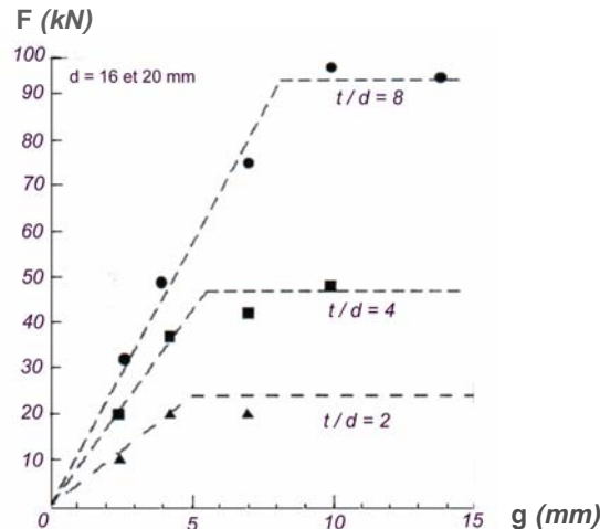
Figure A.18 : Effet du talon sur la capacité maximale d'assemblages unitaires bois-métal en double cisaillement en traction longitudinale (essence Epicéa)
