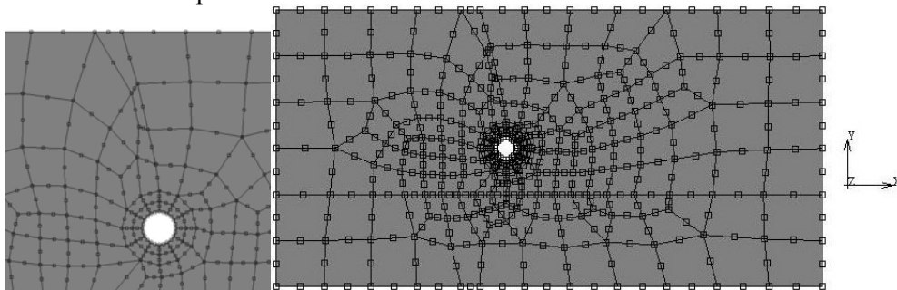
Figure B.14 : Maillage concentrique autour de l'organe d'assemblage
