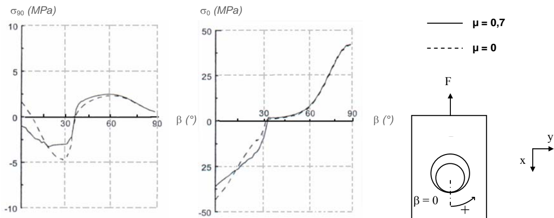
Figure A.11 : Effet du frottement sur les contraintes
