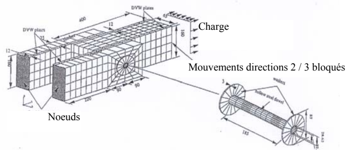
Figure B.11 : Assemblage simulé
