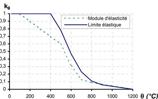
Figure A.50 : Coefficients de réduction des propriétés mécaniques de l'acier [EUR3 01]
