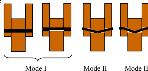
Figure A.14 : Modes de rupture des assemblages bois-bois
