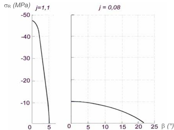
Figure A.12 : Effet du jeu diamétral (j) sur la pression radiale pour de l'Épicéa
