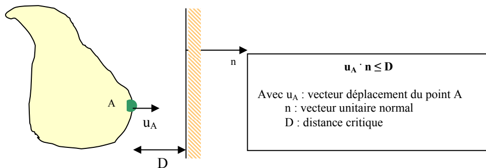
Figure B.20 : Critère de non-pénétration
