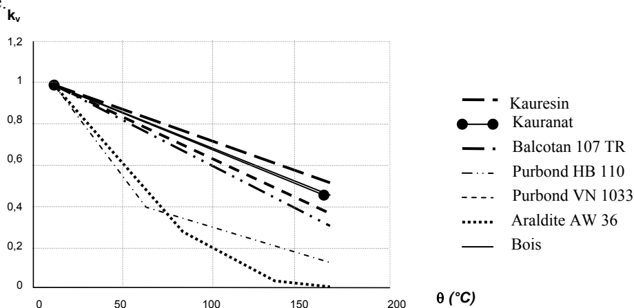
Figure A.32 : Coefficient de réduction de la résistance en cisaillement des joints de collage et du bois
