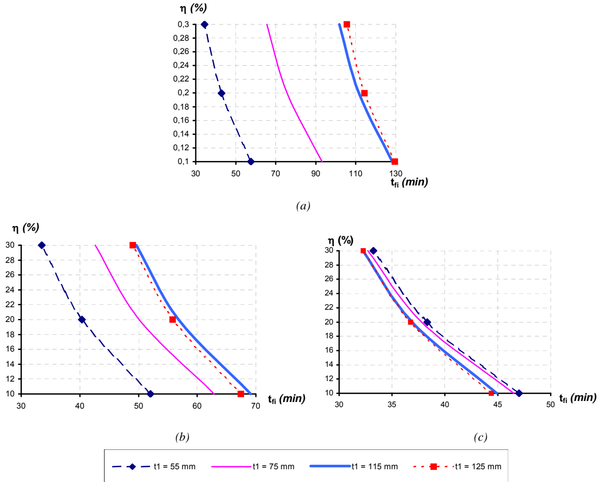
Figure C.41 : Evolution du taux de chargement en fonction de la durée de résistance au feu : (a) bois-bois d=20\text{mm} , (b) bois-métal d=20\text{mm} , (c) bois-métal d=12\text{mm}
