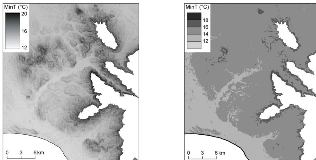
Figure 34 : Modélisation multicritères des températures minimales moyennes dans le district viticole de Stellenbosch (a) et discrétisation suivant les températures utilisées pour la maturité de la vigne (b) (réalisation M. Madelin).
